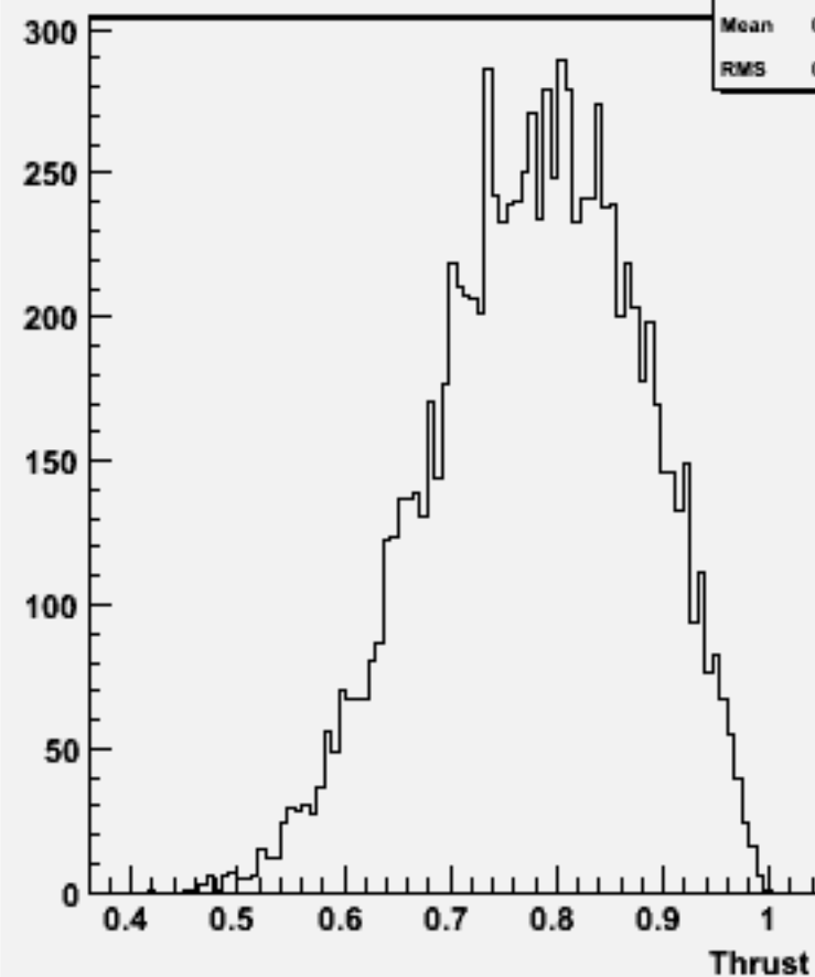
Thrust w101705 ccn1e1e3n3_o
