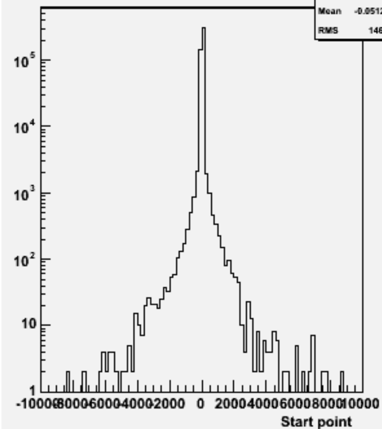
Start point Z : w101705 ccn1e1e3n3_o
