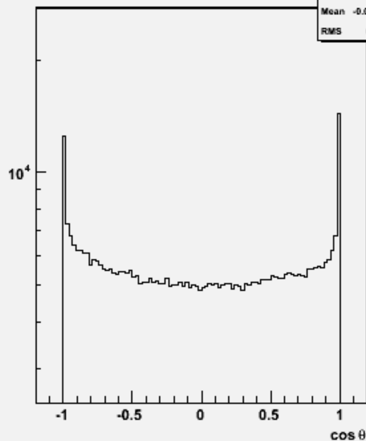
Particle cosθ : w101705 ccn1e1e3n3_o
