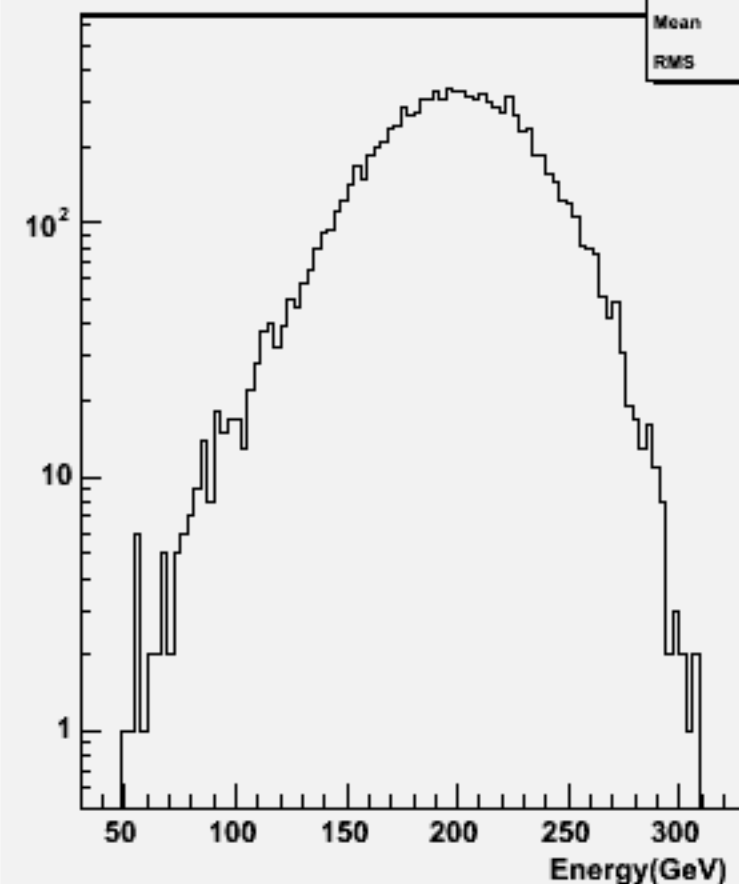
Thrust w101705 ccn1e1e3n3_o
