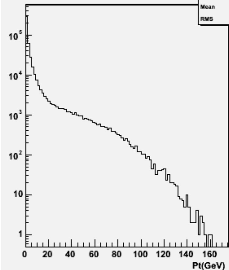
Particle Pt : w101705 ccn1e1e3n3_o
