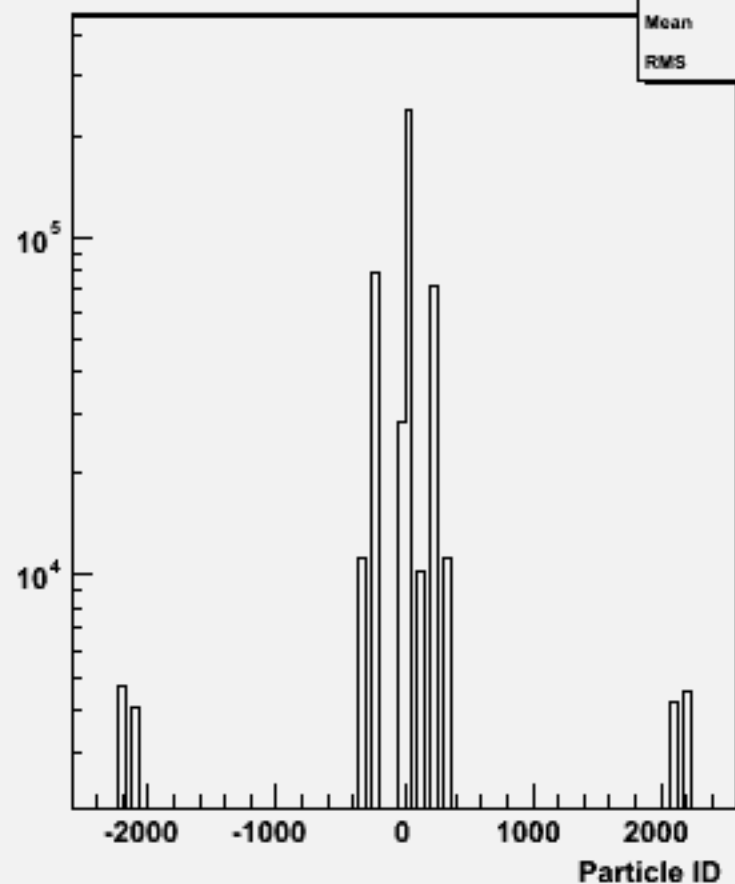
Particle ID : w101705 ccn1e1e3n3_o
