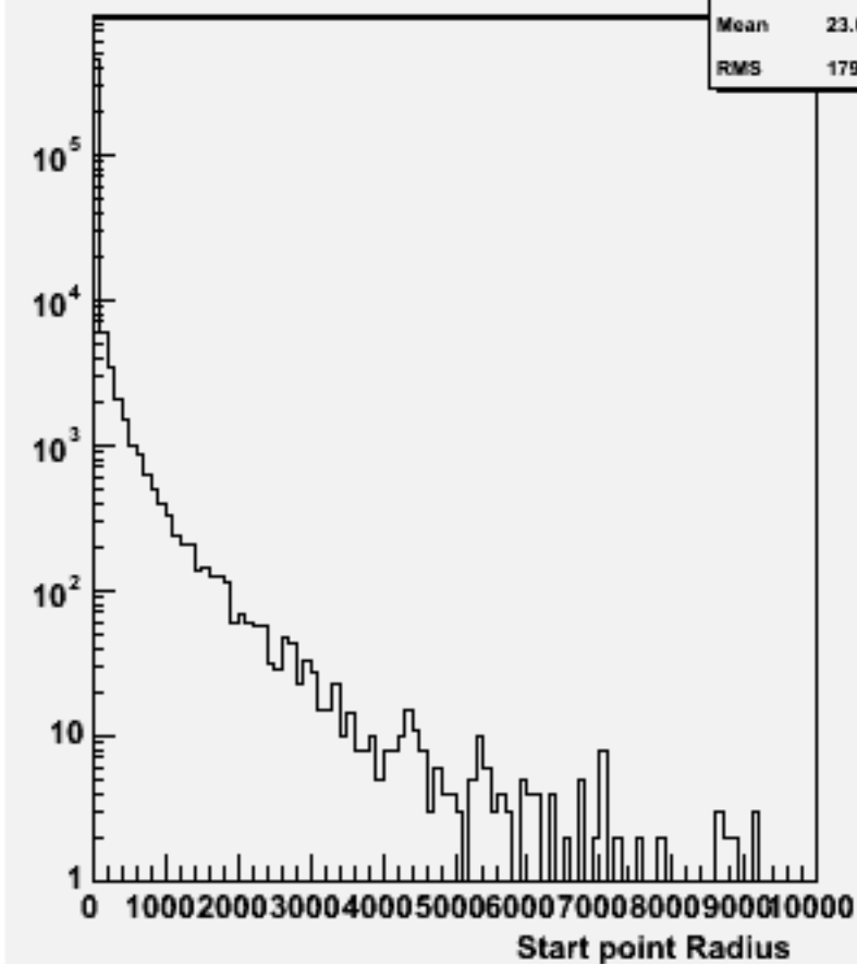
Start point R : w101705 ccn1e1e3n3_o
