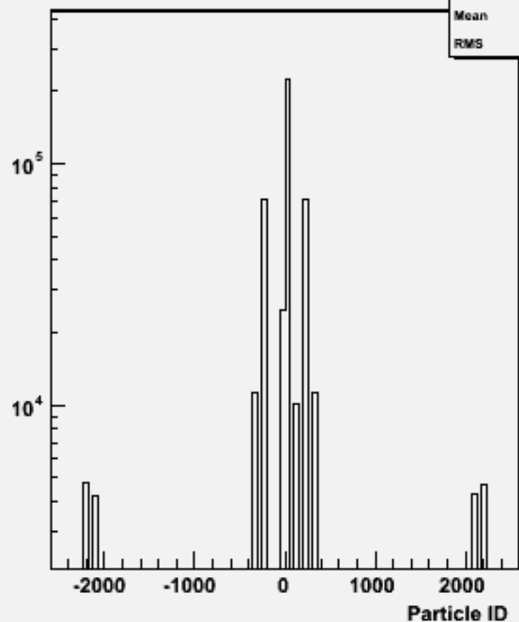
Particle ID : w101701 ccn1e1e2n2_o
