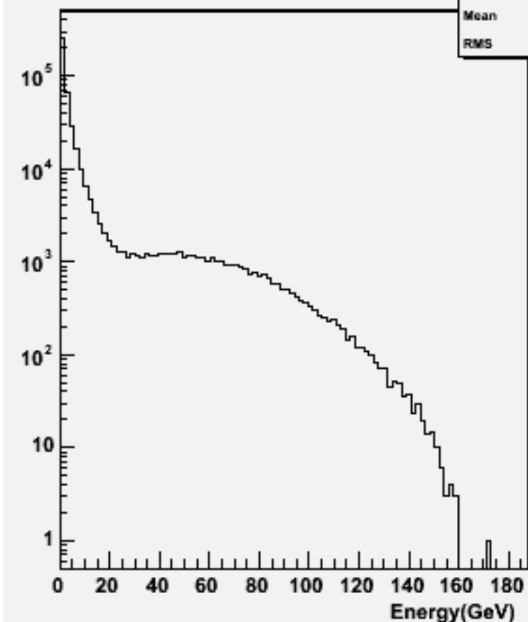
Particle Energy : w101701 ccn1e1e2n2_o
