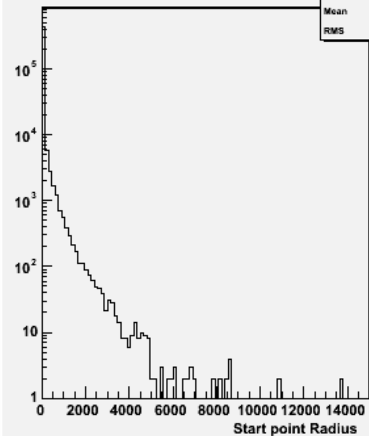
Start point R : w101701 ccn1e1e2n2_o
