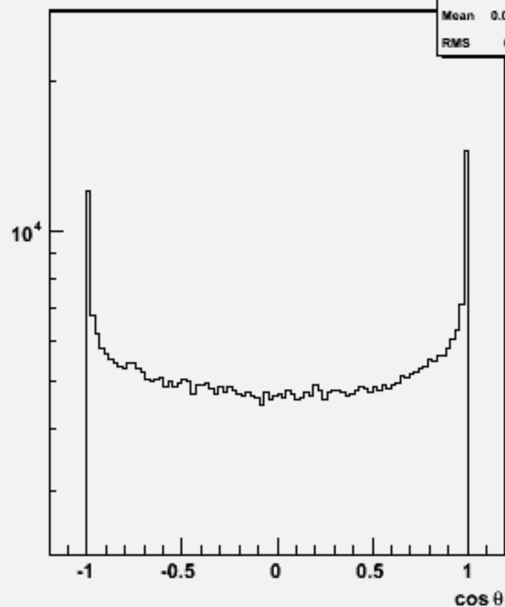
Particle cos \theta : w101701 ccn1e1e2n2_o
