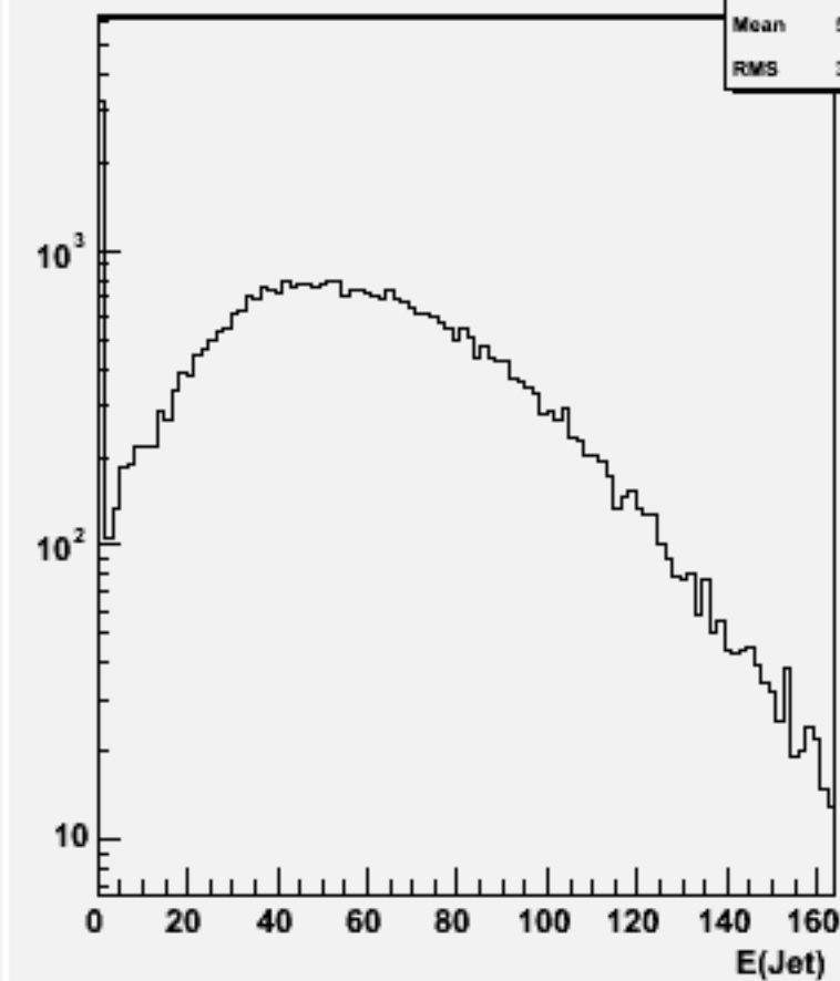
Jet energies(All jets)w101701 ccn1e1e2n2_o
