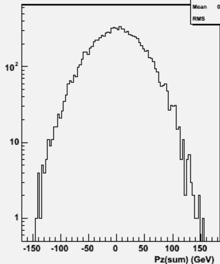
Pz Sum: w101701 ccn1e1e2n2_o
