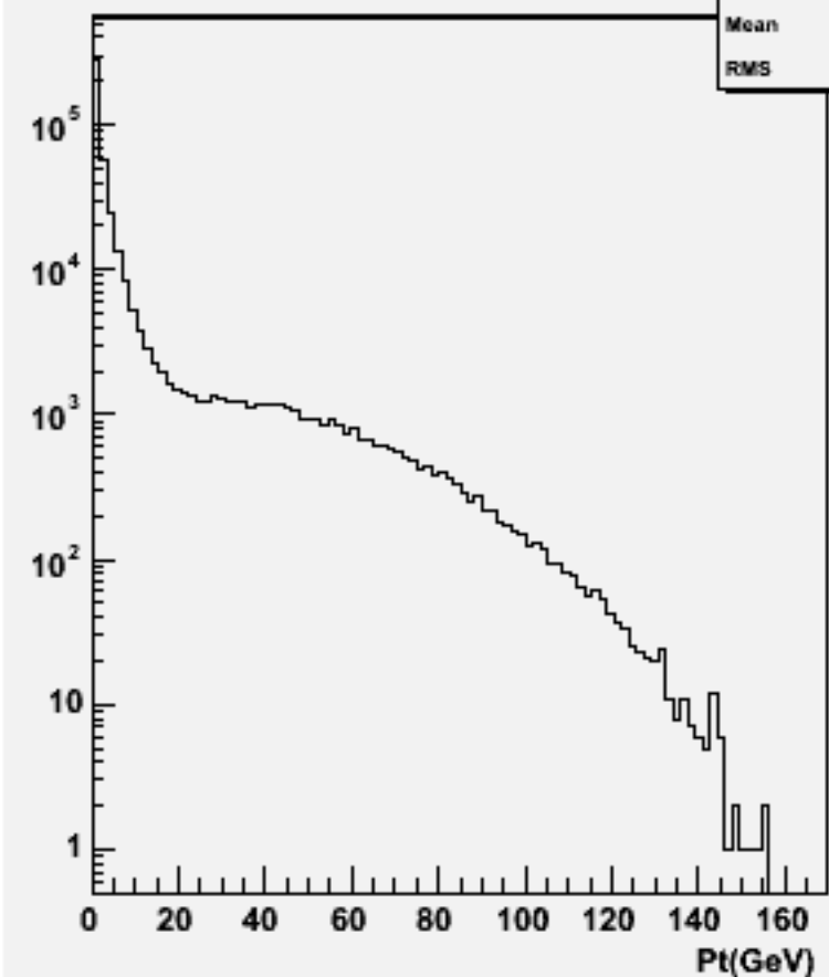
Particle Pt : w101701 ccn1e1e2n2_o
