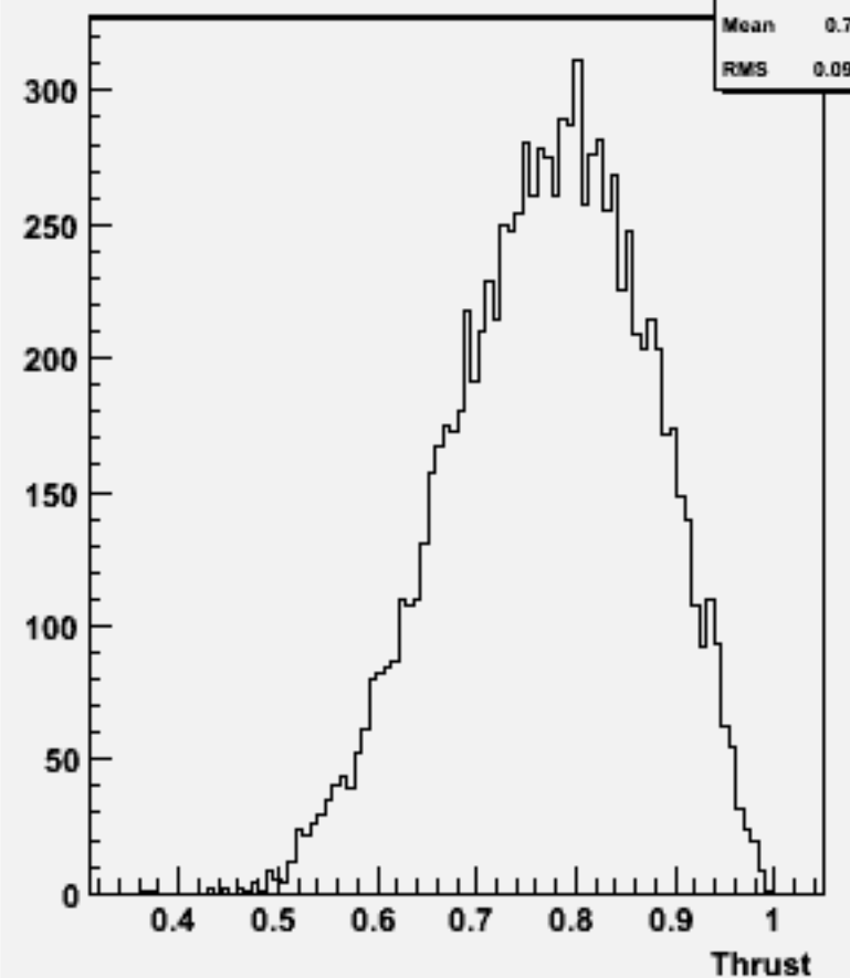
Thrust w101701 ccn1e1e2n2_o
