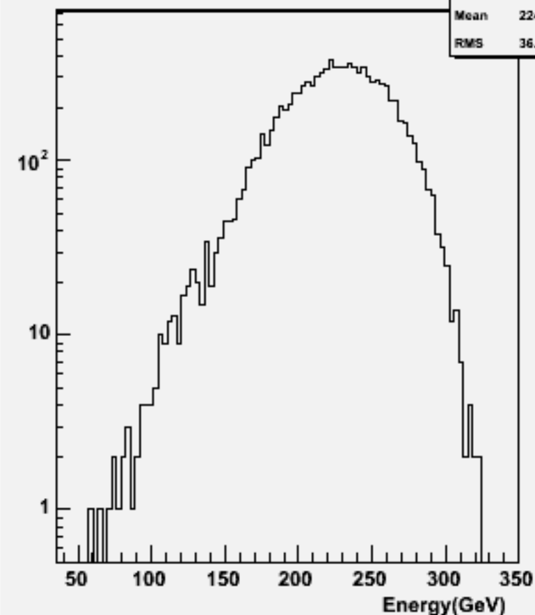
Thrust w101701 ccn1e1e2n2_o
