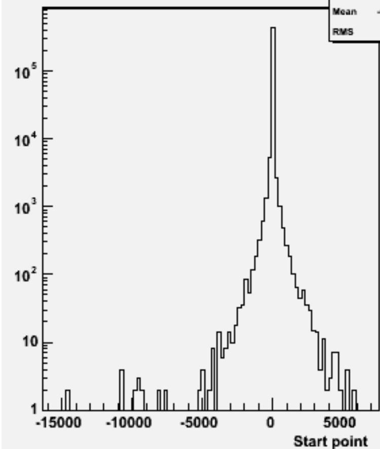
Start point Z : w101701 ccn1e1e2n2_o
