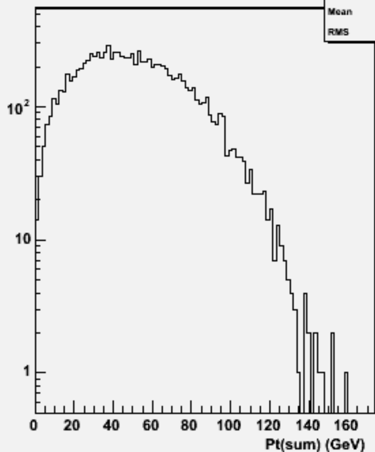
Pt Sum: w101701 ccn1e1e2n2_o
