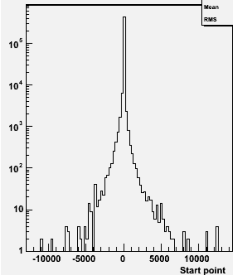
Start point Z : w101700 ccn1e1e2n2_o
