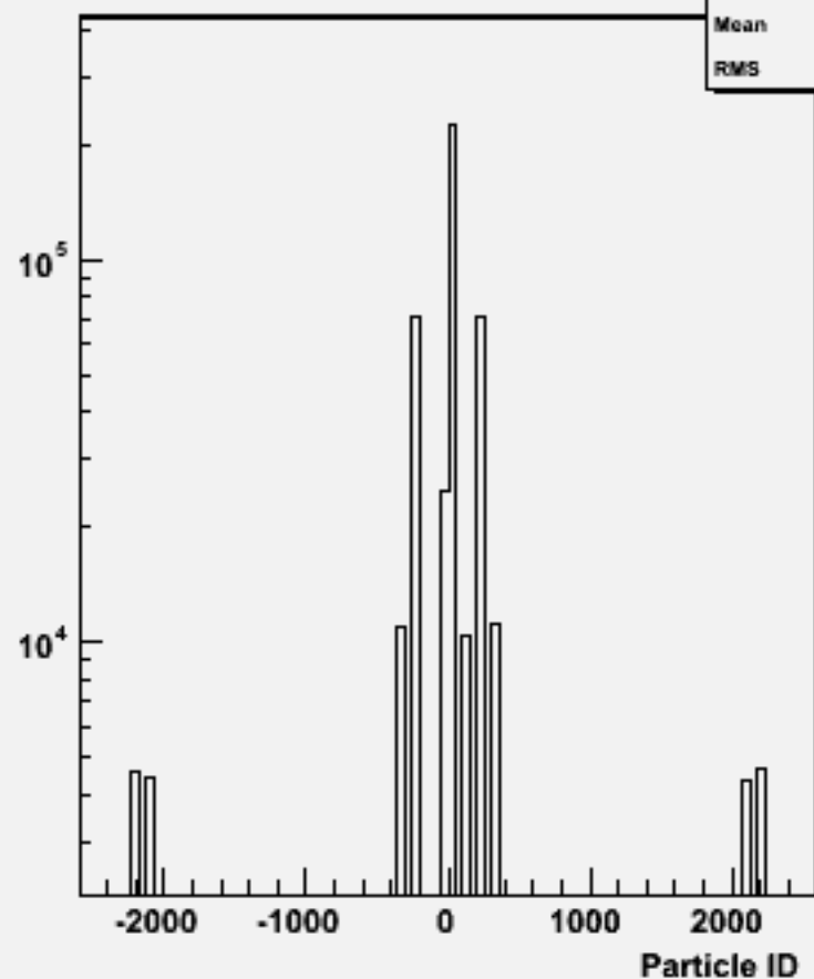
Particle ID : w101700 ccn1e1e2n2_o
