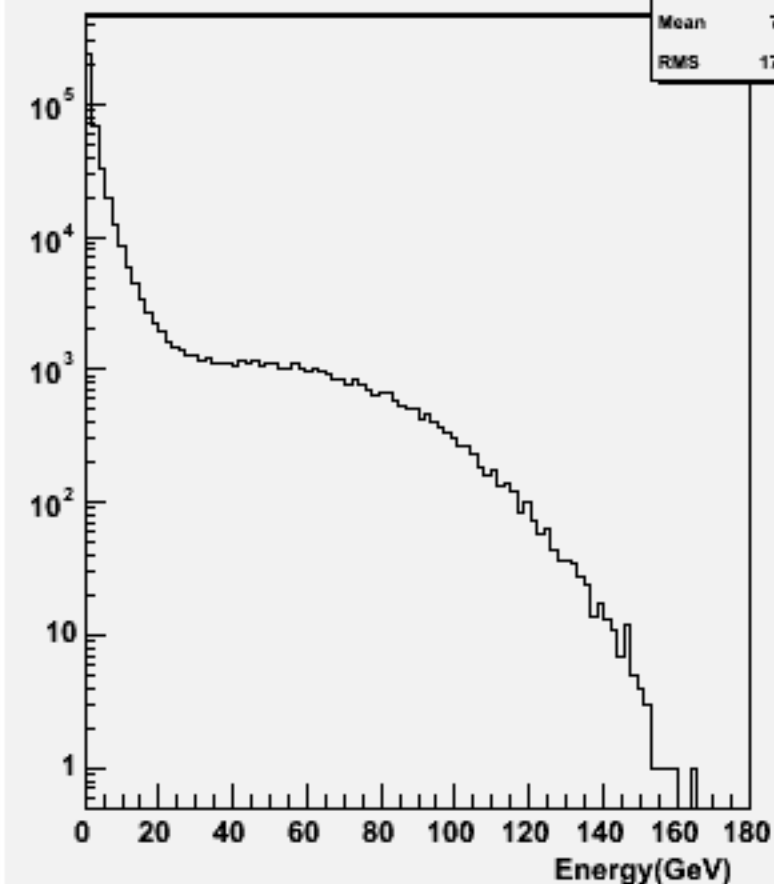
Particle Energy : w101700 ccn1e1e2n2_o
