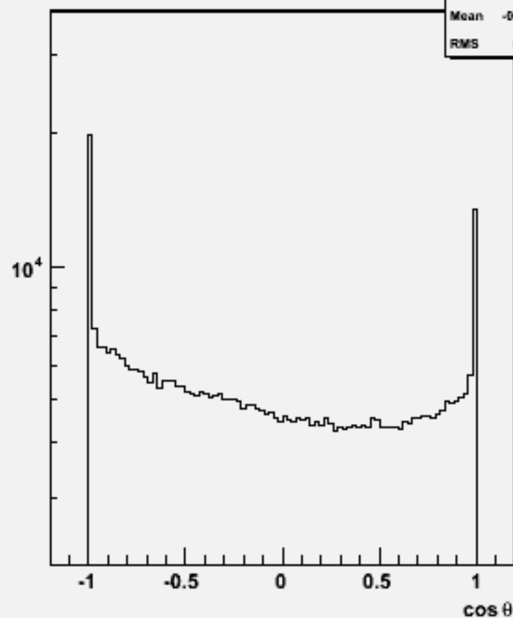
Particle cosθ : w101700 ccn1e1e2n2_o
