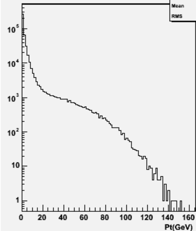
Particle Pt : w101700 ccn1e1e2n2_o
