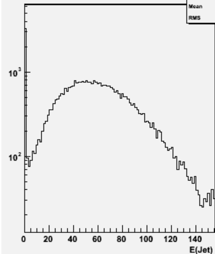
Jet energies(All jets)w101700 ccn1e1e2n2_o
