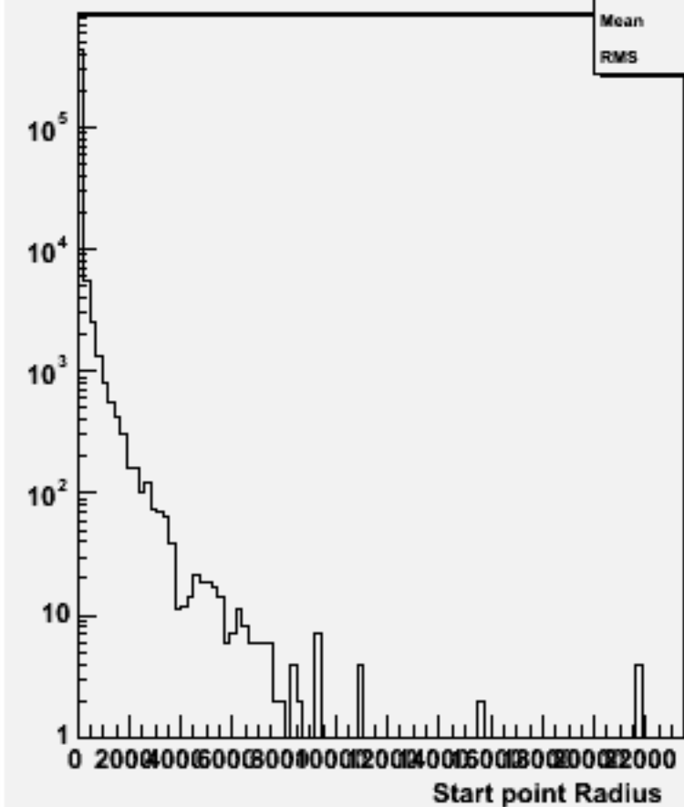
Start point R : w101700 ccn1e1e2n2_o
