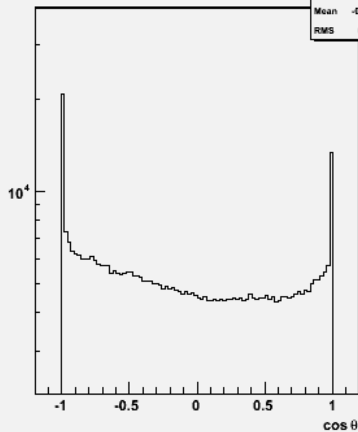
Particle cosθ : w101699 ccn1e1e2n2_o
