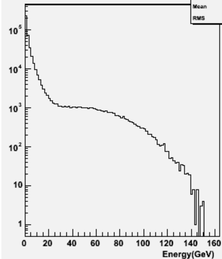
Particle Energy : w101699 ccn1e1e2n2_o
