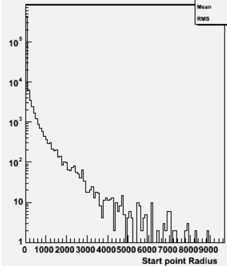
Start point R : w101699 ccn1e1e2n2_o
