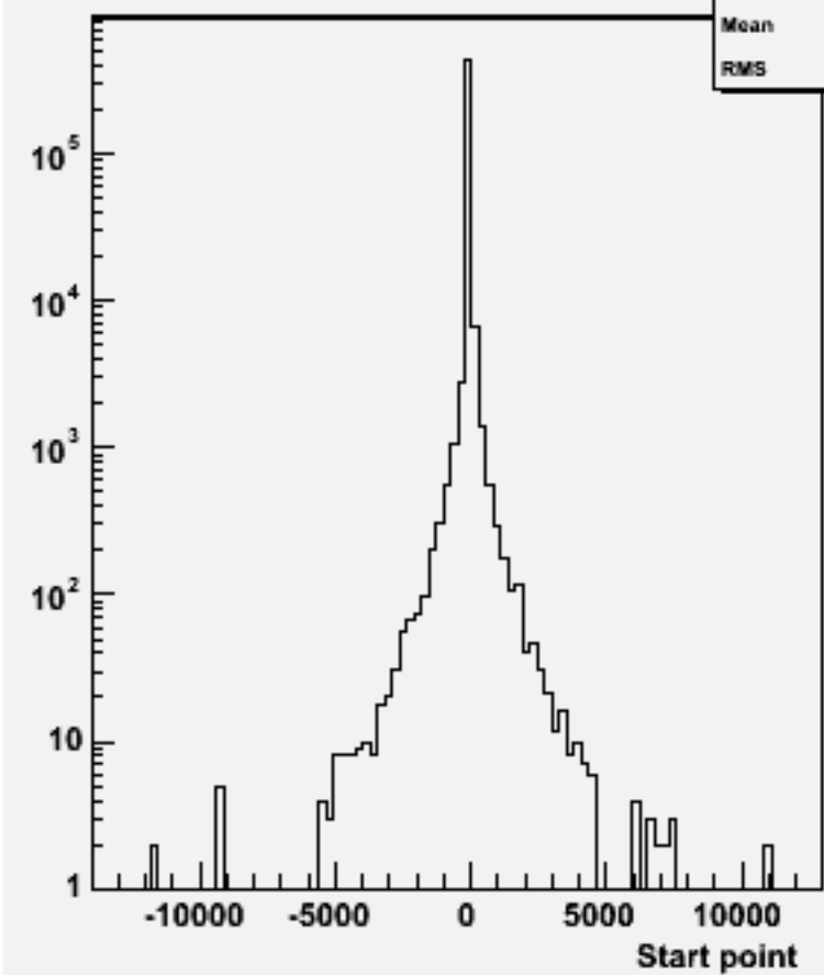
Start point Z : w101699 ccn1e1e2n2_o
