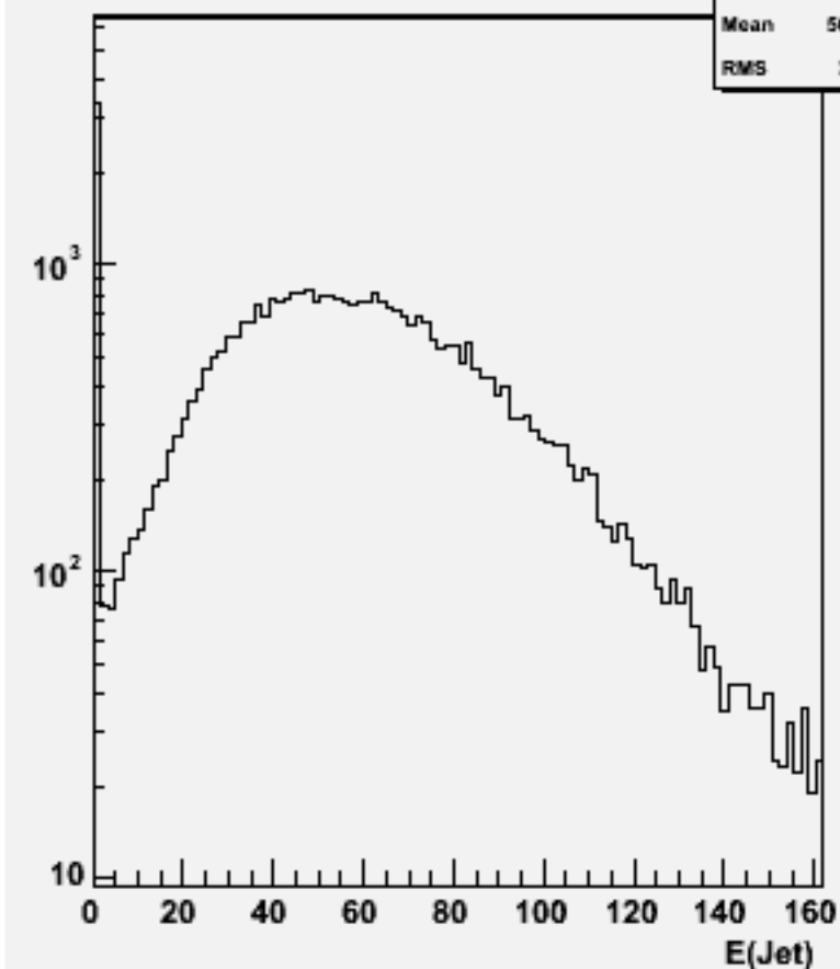
Jet energies(All jets)w101699 ccn1e1e2n2_o
