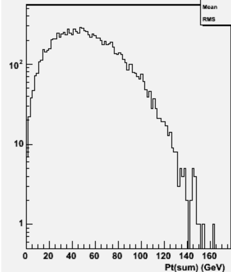
Pt Sum: w101699 ccn1e1e2n2_o
