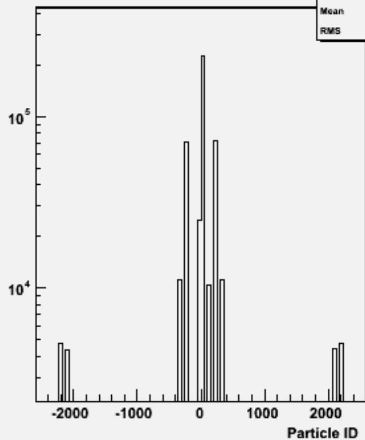
Particle ID : w101699 ccn1e1e2n2_o
