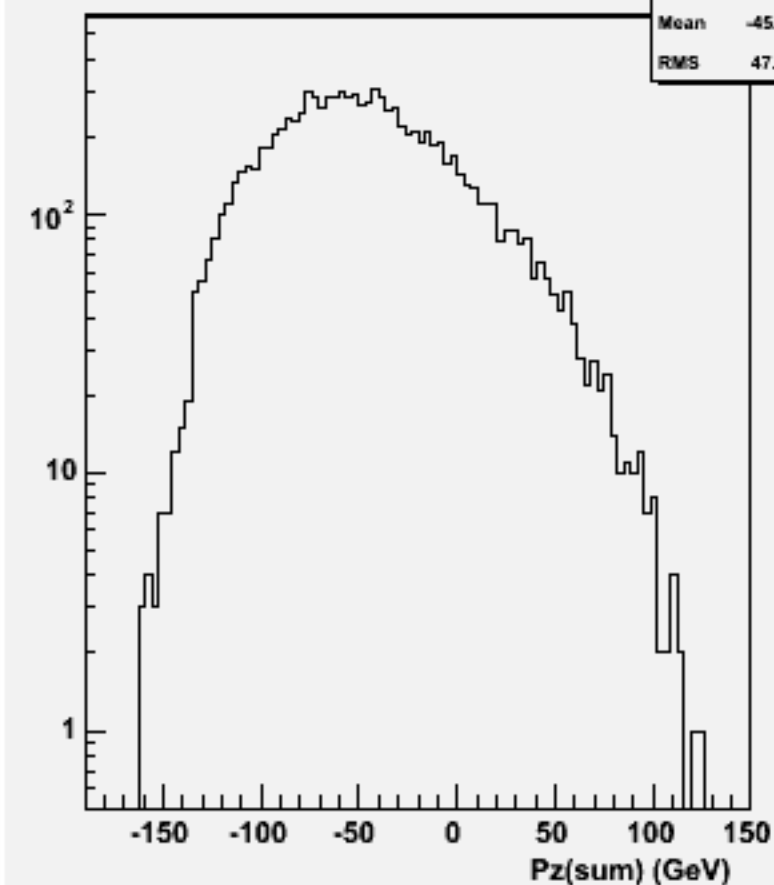
Pz Sum: w101699 ccn1e1e2n2_o
