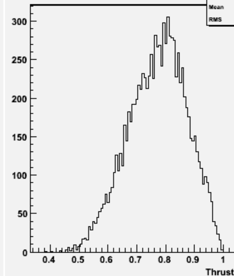
Thrust w101699 ccn1e1e2n2_o
