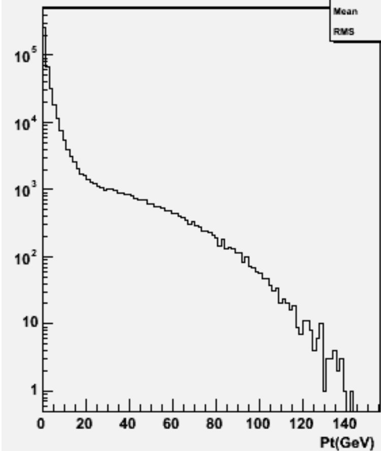
Particle Pt : w101699 ccn1e1e2n2_o
