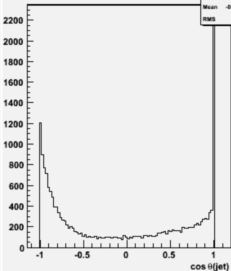
cos \theta for 2-jets :w101699 ccn1e1e2n2_o
