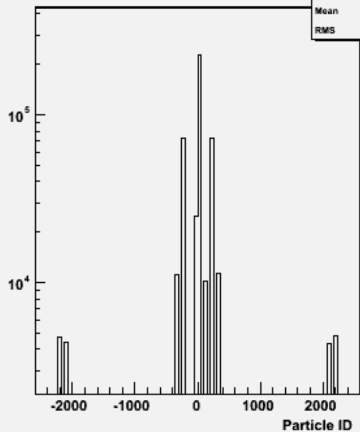
Particle ID : w101698 ccn1e1e1n1_o
