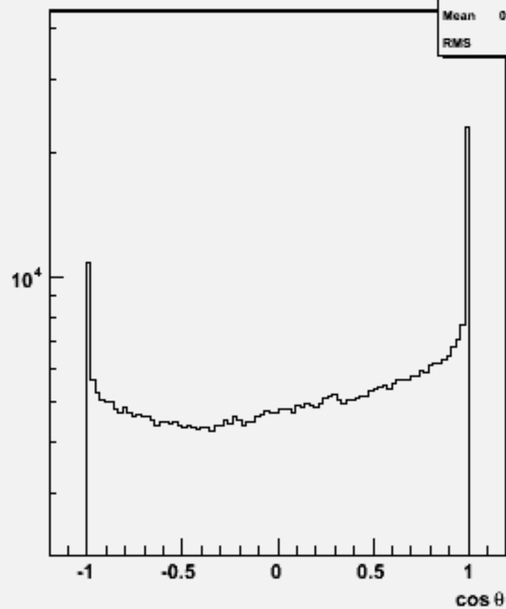
Particle cos \theta : w101698 ccn1e1e1n1_o
