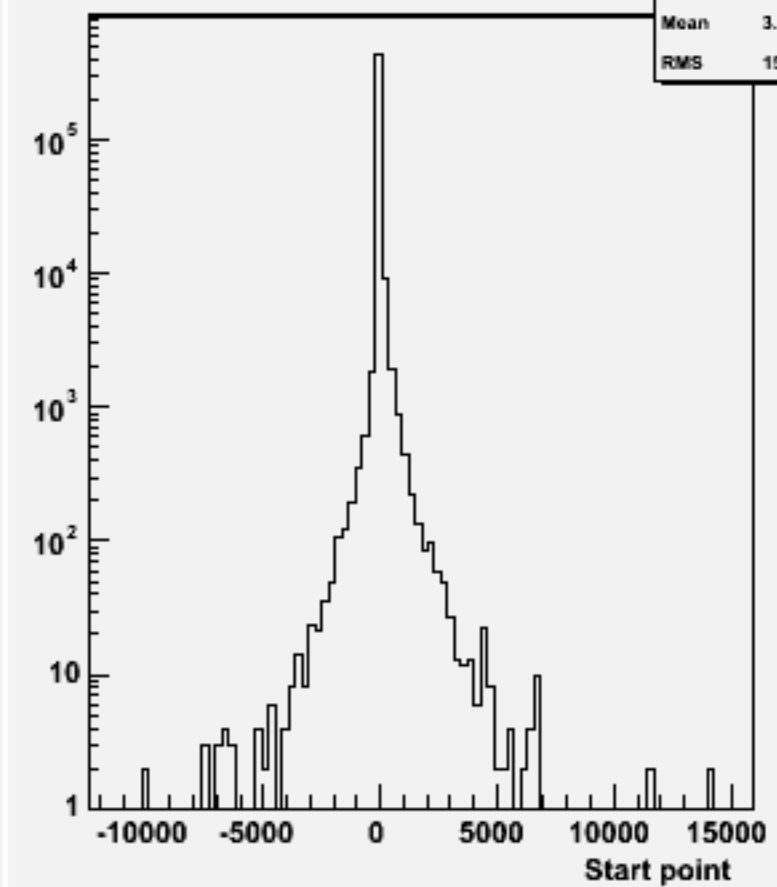
Start point Z : w101698 ccn1e1e1n1_o
