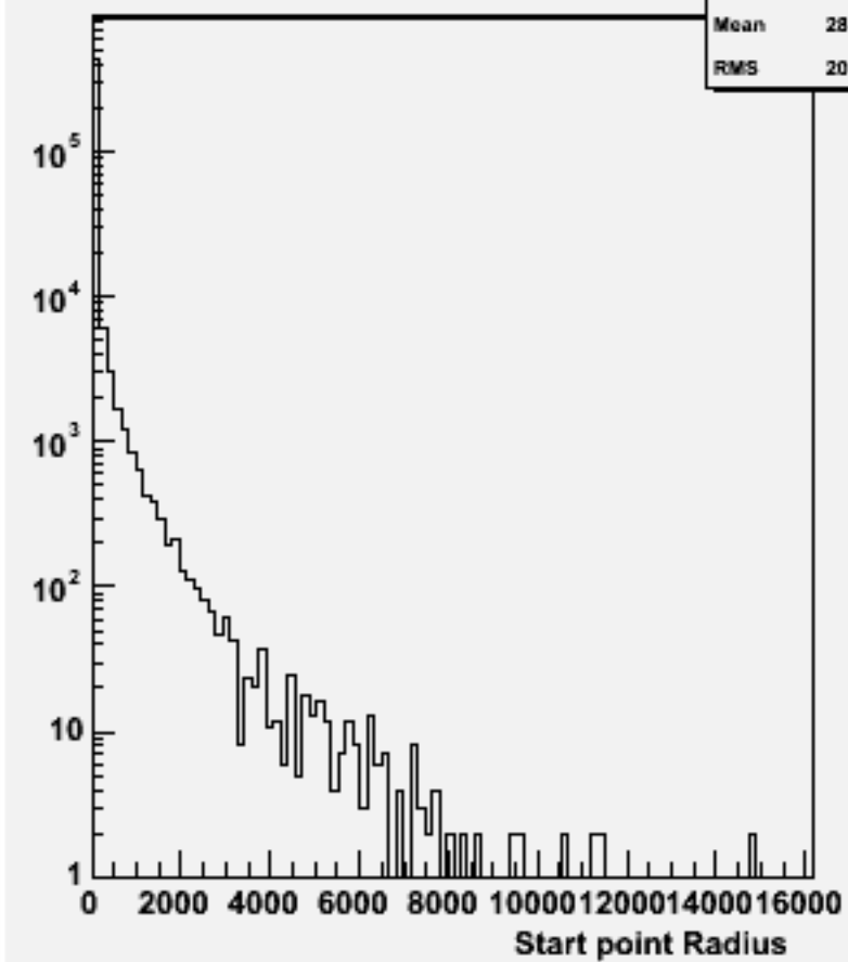
Start point R : w101698 ccn1e1e1n1_o
