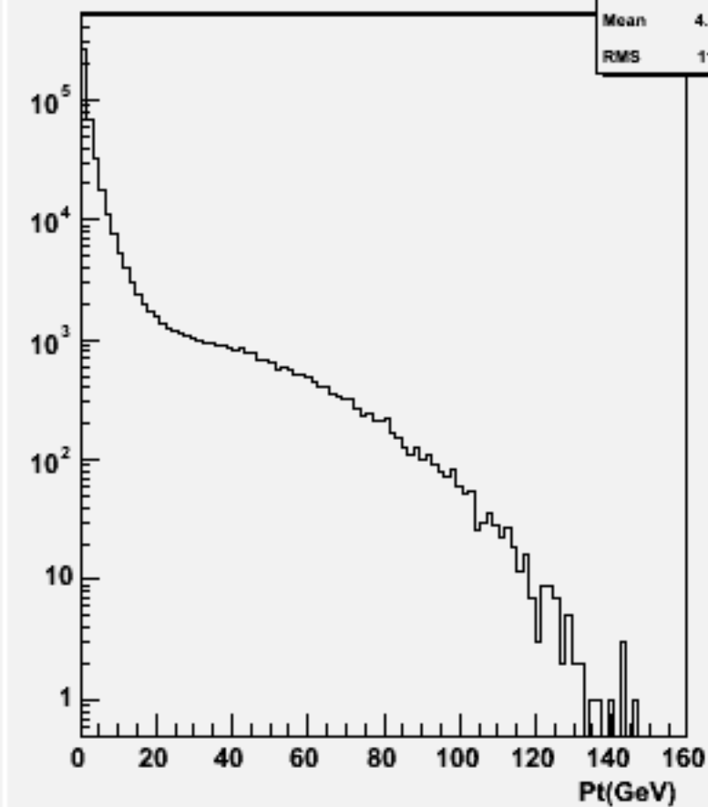
Particle Pt : w101698 ccn1e1e1n1_o
