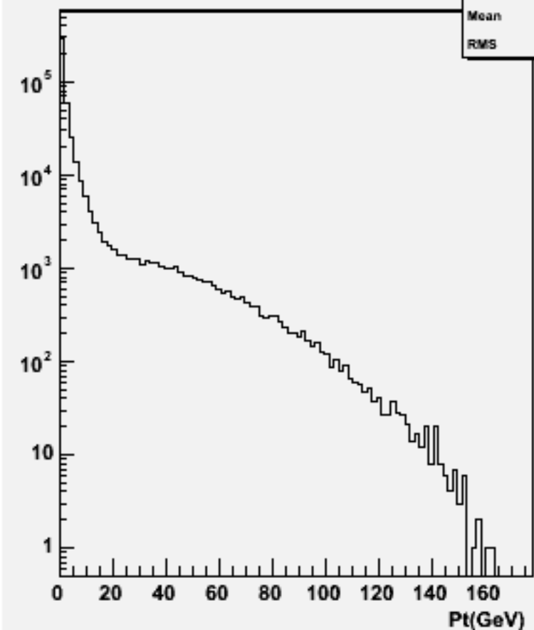
Particle Pt : w101697 ccn1e1e1n1_o
