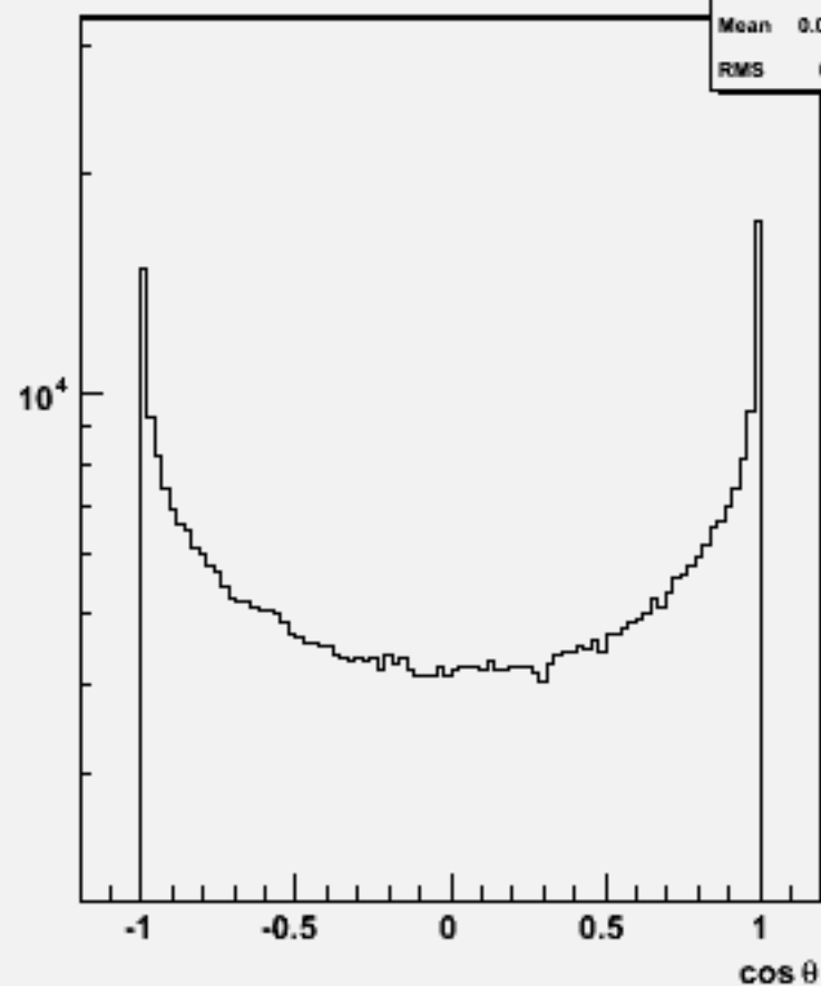
Particle cosθ : w101697 ccn1e1e1n1_o
