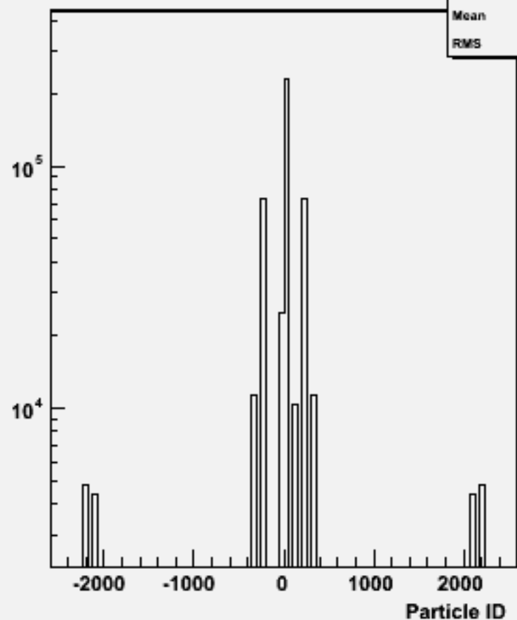
Particle ID : w101697 ccn1e1e1n1_o
