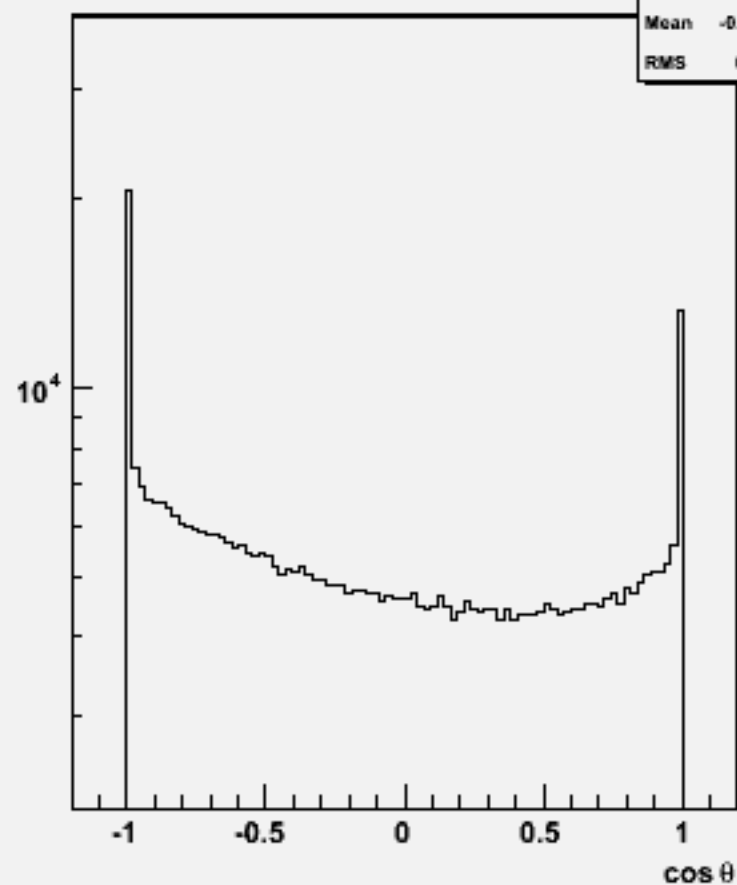
Particle cosθ : w101695 ccn1e1e1n1_o
