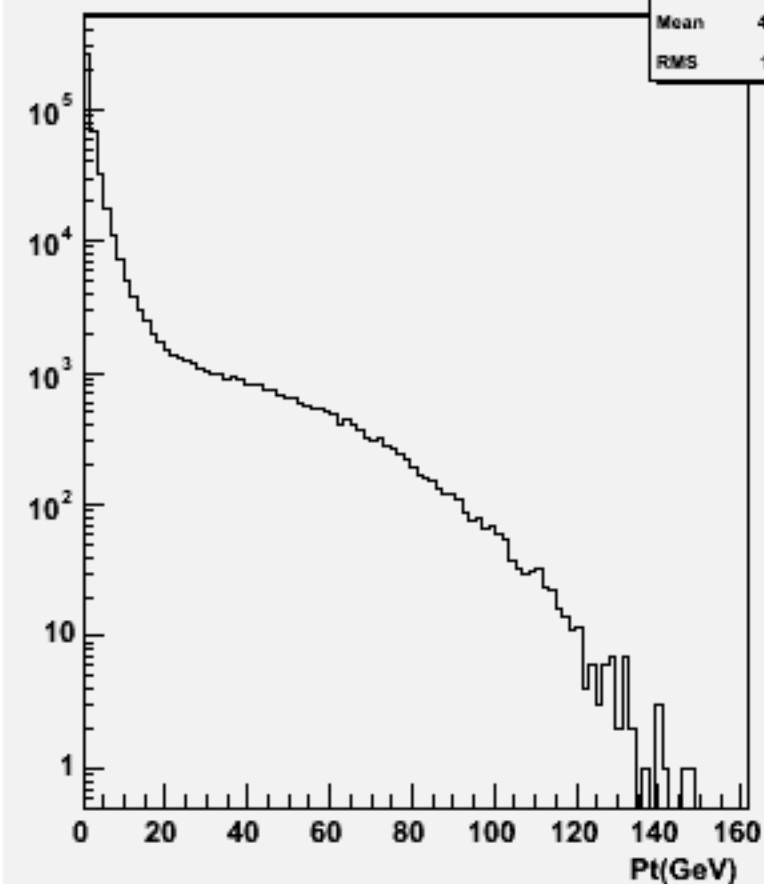
Particle Pt : w101695 ccn1e1e1n1_o
