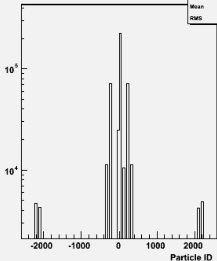
Particle ID : w101695 ccn1e1e1n1_o
