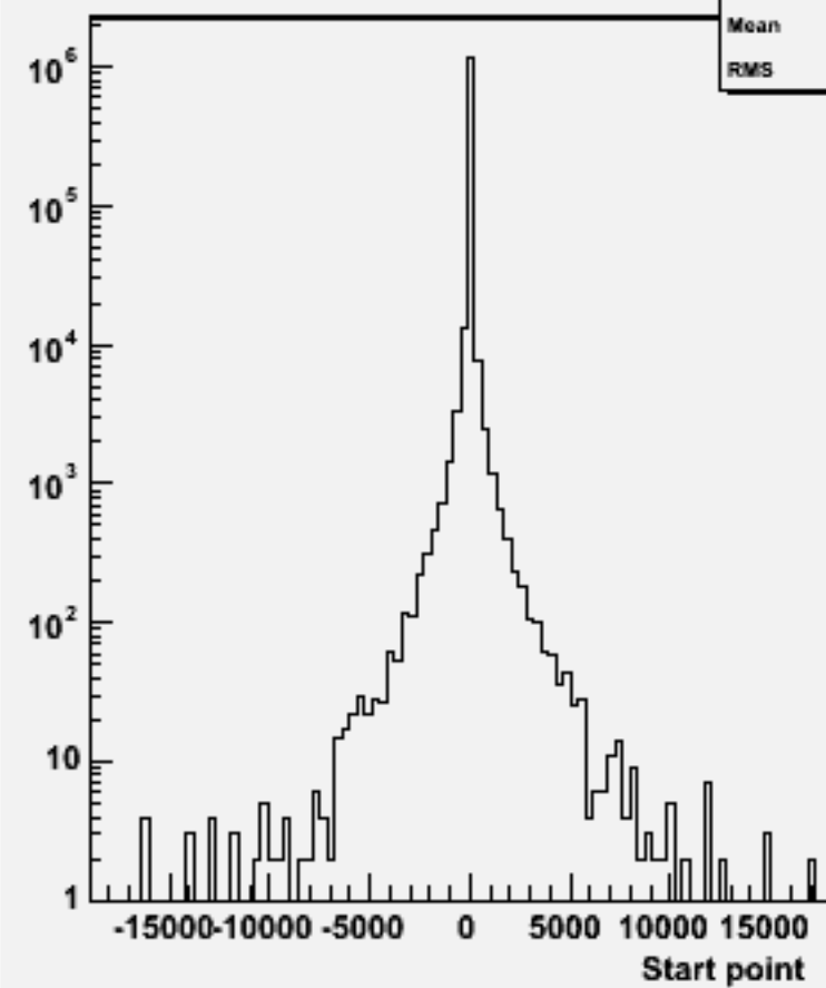
Start point Z : w101693 uucssc_o
