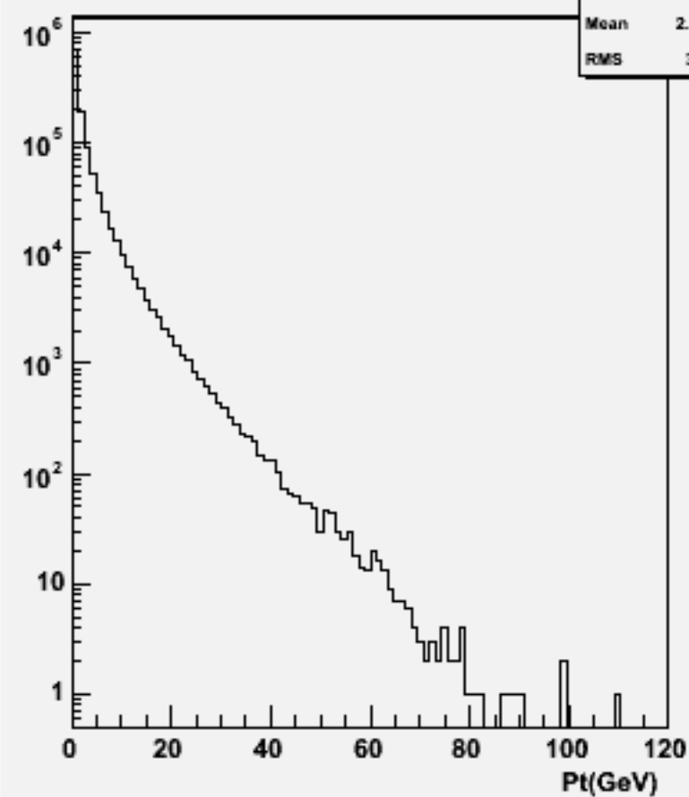
Particle Pt : w101693 uucssc_o
