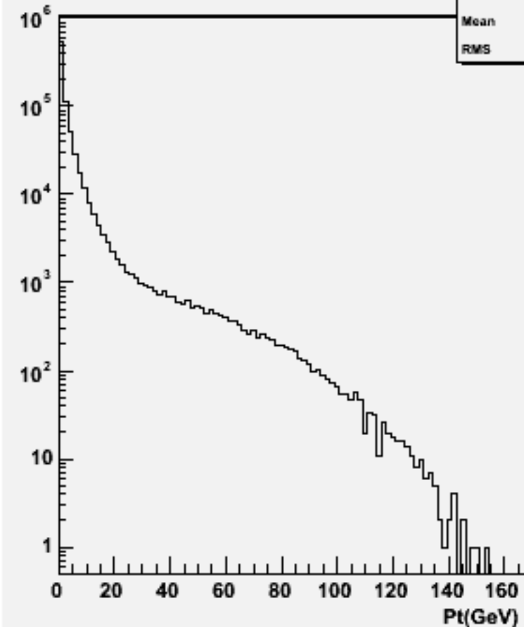
Particle Pt : w101681 uucse2n2_o
