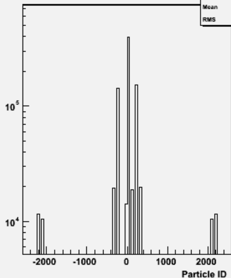
Particle ID : w101681 uucse2n2_o
