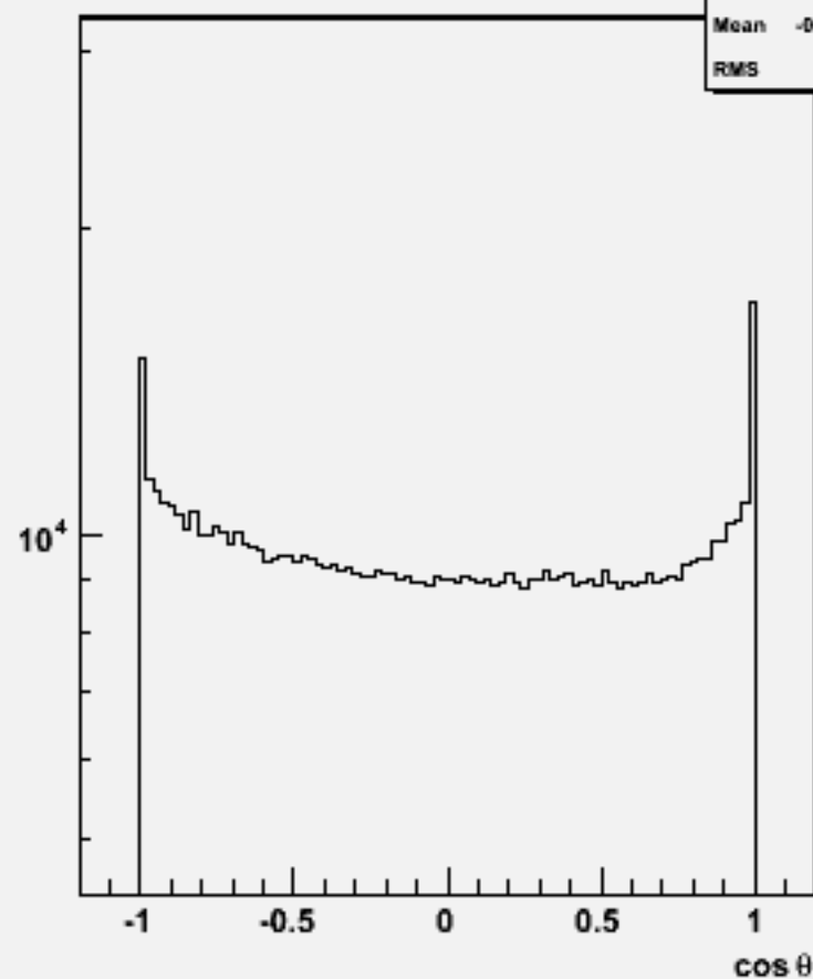
Particle cos \theta : w101681 uucse2n2_o
