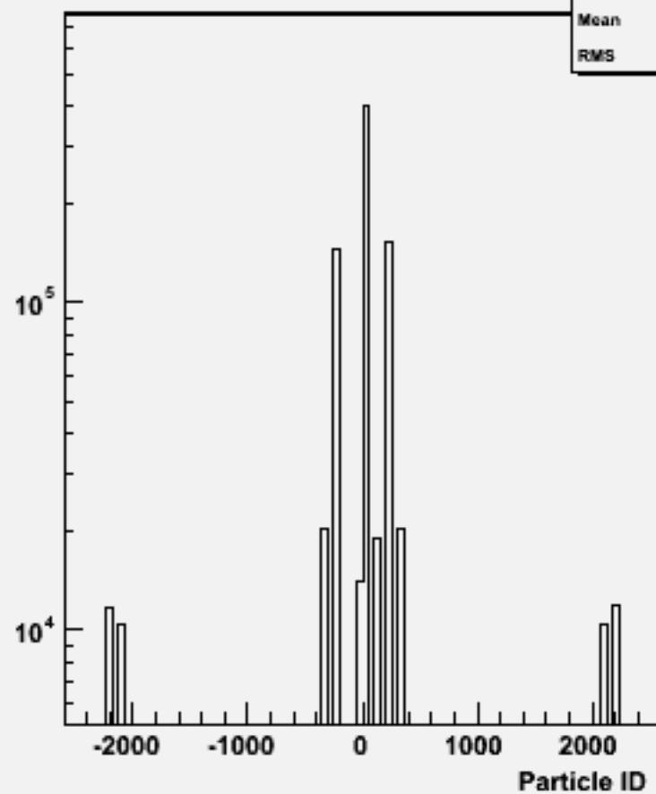
Particle ID : w101680 uucse2n2_o
