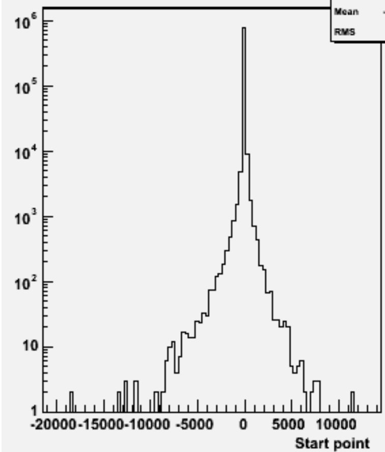
Start point Z : w101680 uucse2n2_o
