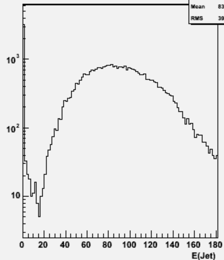
Jet energies(All jets)w101673 uuudsc_o
