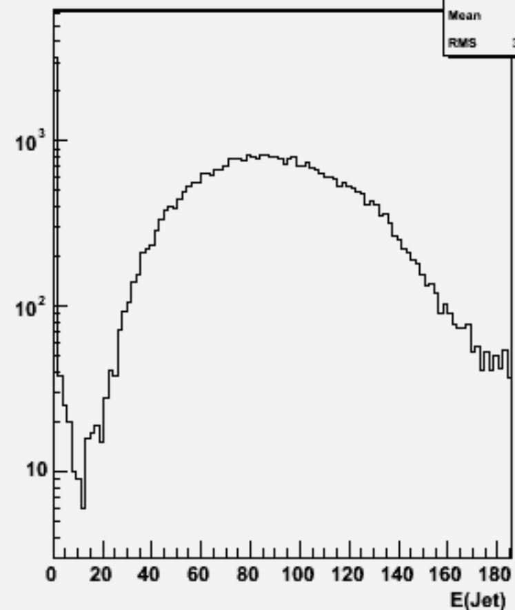
Jet energies(All jets)w101672 uuudsc_o
