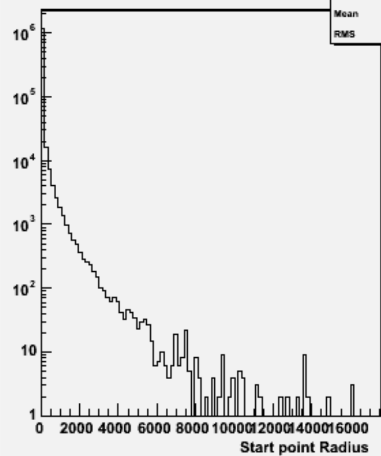
Start point R : w101672 uuudsc_o
