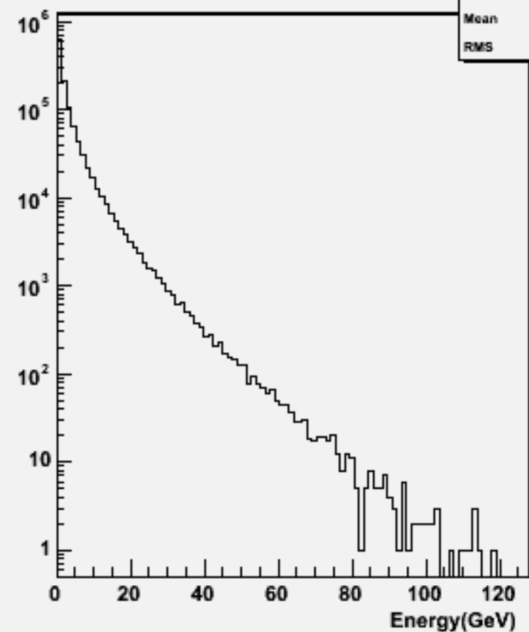
Particle Energy : w101672 uuudsc_o
