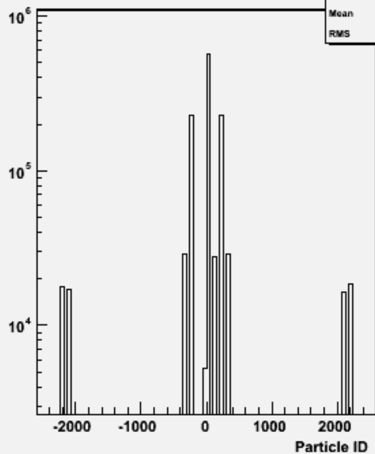
Particle ID : w101672 uuudsc_o
