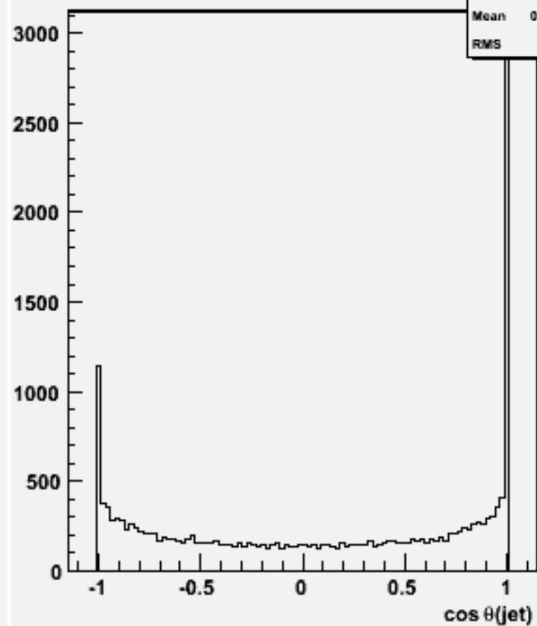
cos \theta for 2-jets :w101672 uuudsc_o
