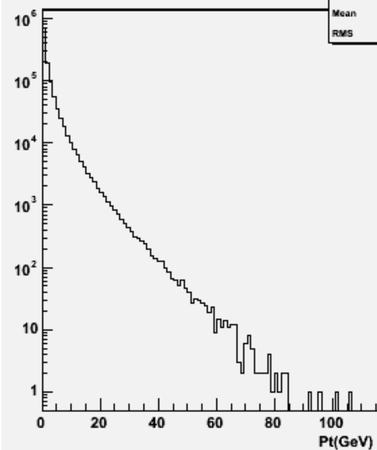
Particle Pt : w101672 uuudsc_o
