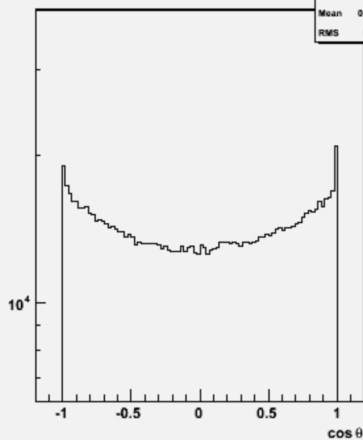
Particle cos \theta : w101672 uuudsc_o
