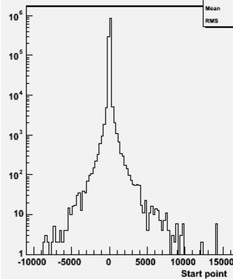
Start point Z : w101672 uuudsc_o
