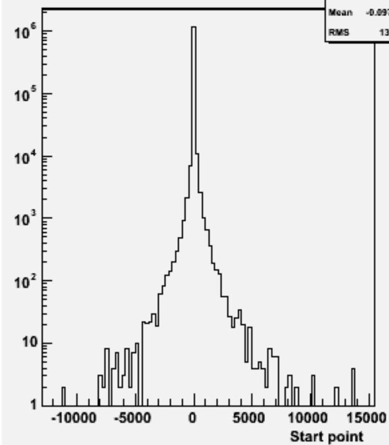
Start point Z : w101668 uuuddu_o
