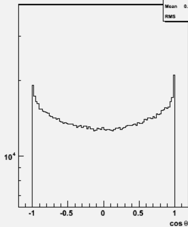
Particle cosθ : w101668 uuuddu_o
