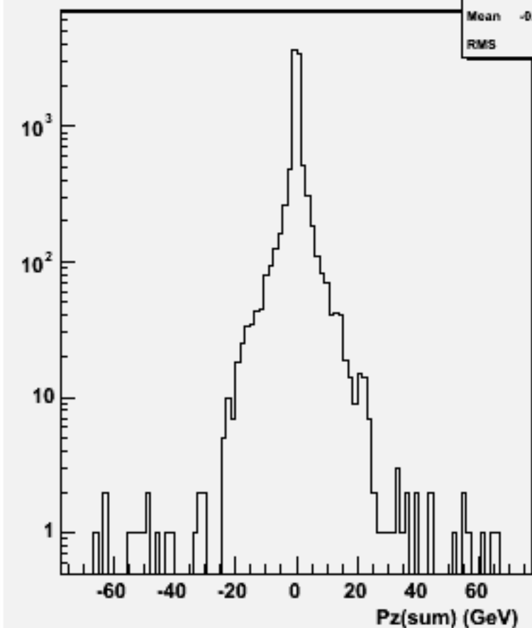
Pz Sum: w101668 uuuddu_o
