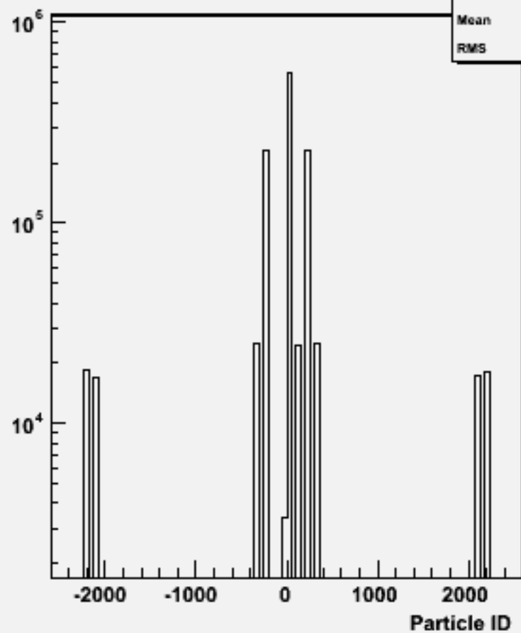
Particle ID : w101668 uuuddu_o
