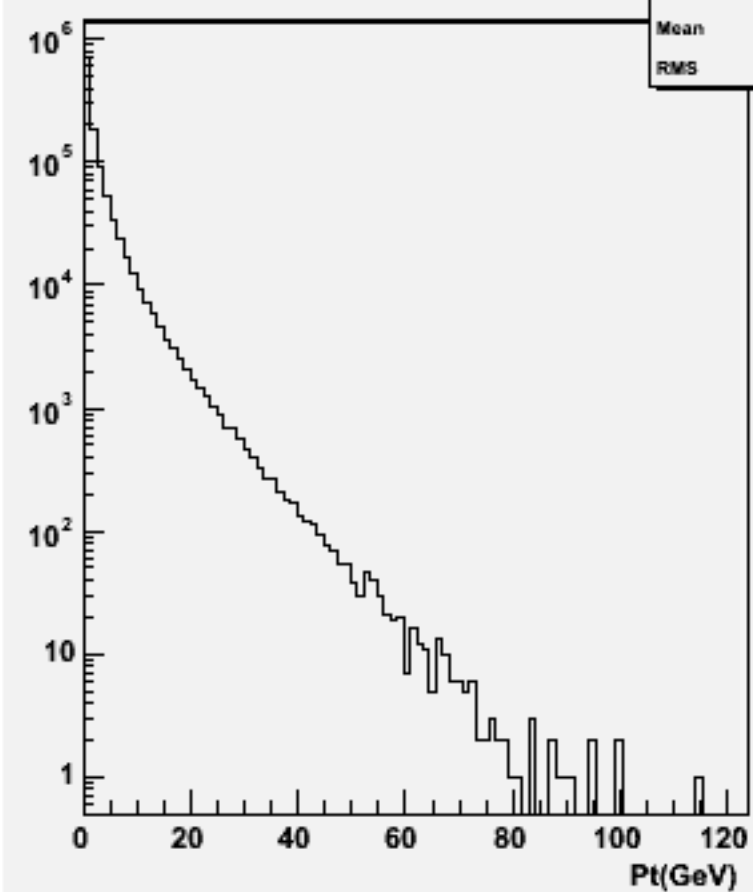
Particle Pt : w101668 uuuddu_o
