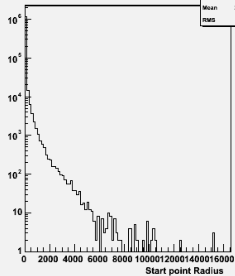
Start point R : w101668 uuuddu_o
