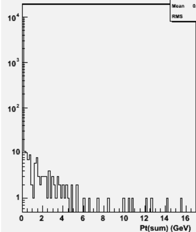
Pt Sum: w101668 uuuddu_o
