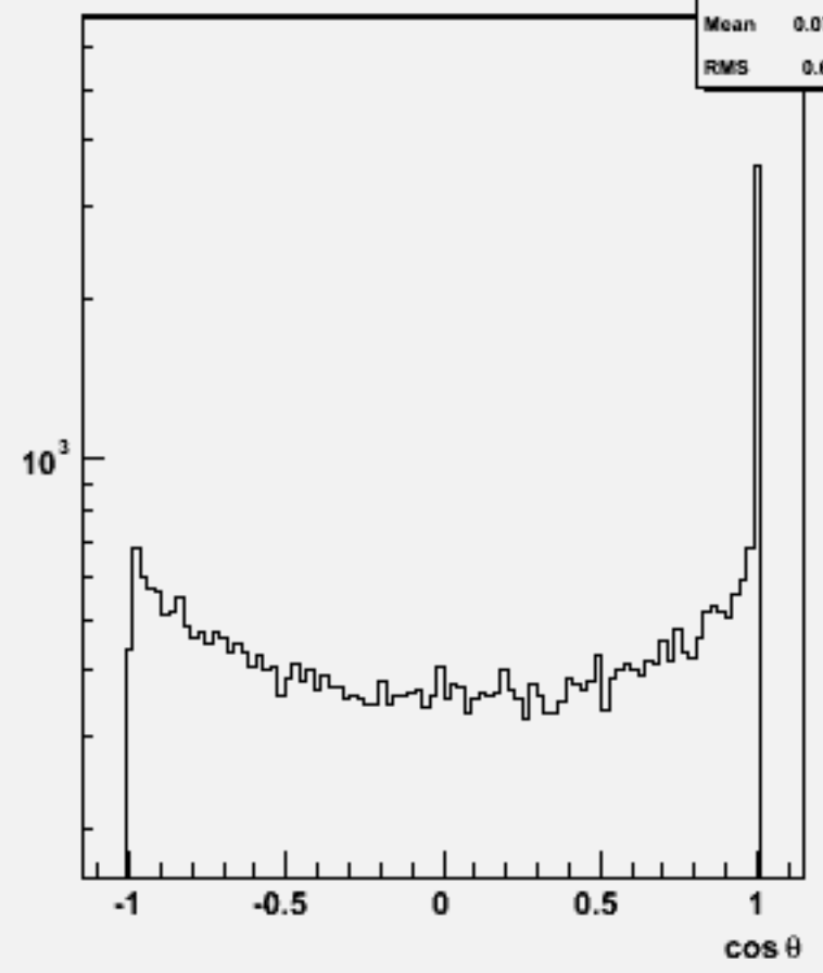
Jet cosθ (All jets)w101664 uuude3n3_o
