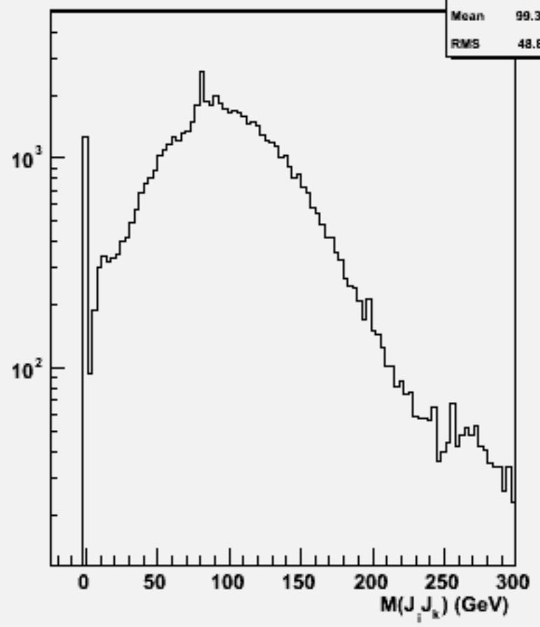
2jets mass(All comb)w101664 uuude3n3_o
