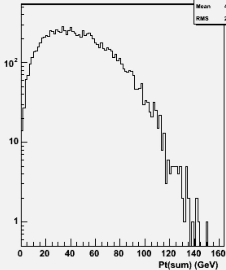
Pt Sum: w101664 uuude3n3_o
