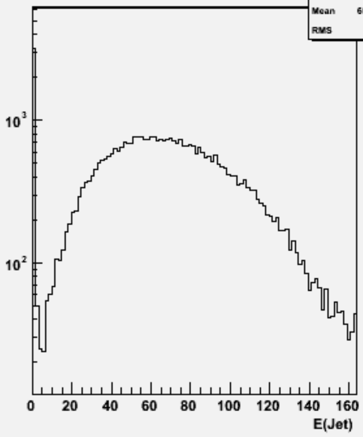
Jet energies(All jets)w101664 uuude3n3_o
