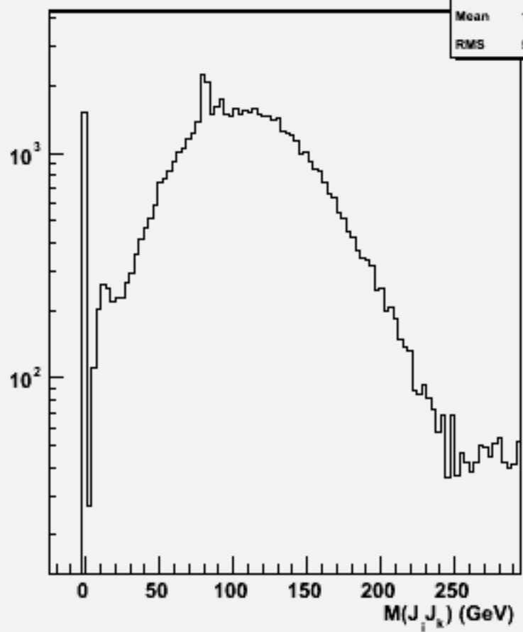
2jets mass(All comb)w101657 uuude1n1_o
