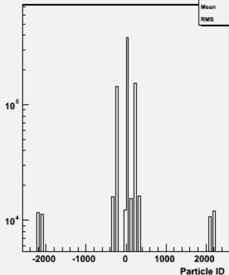
Particle ID : w101657 uuude1n1_o
