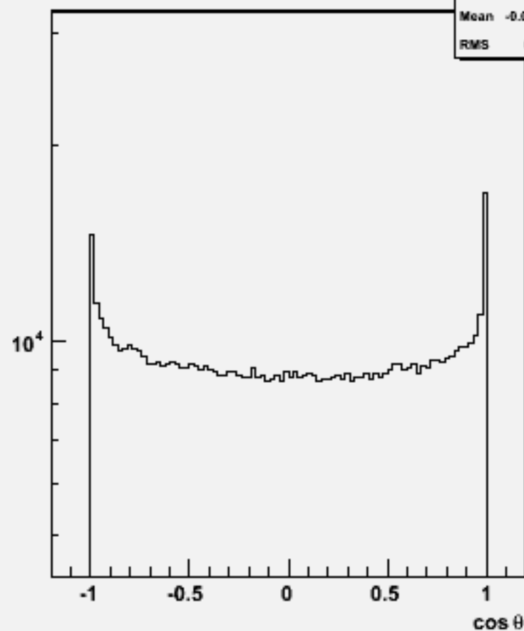
Particle cos \theta : w101657 uuude1n1_o
