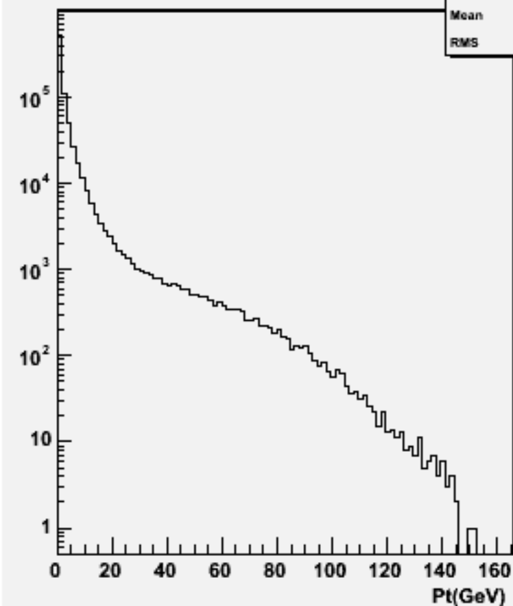
Particle Pt : w101657 uuude1n1_o
