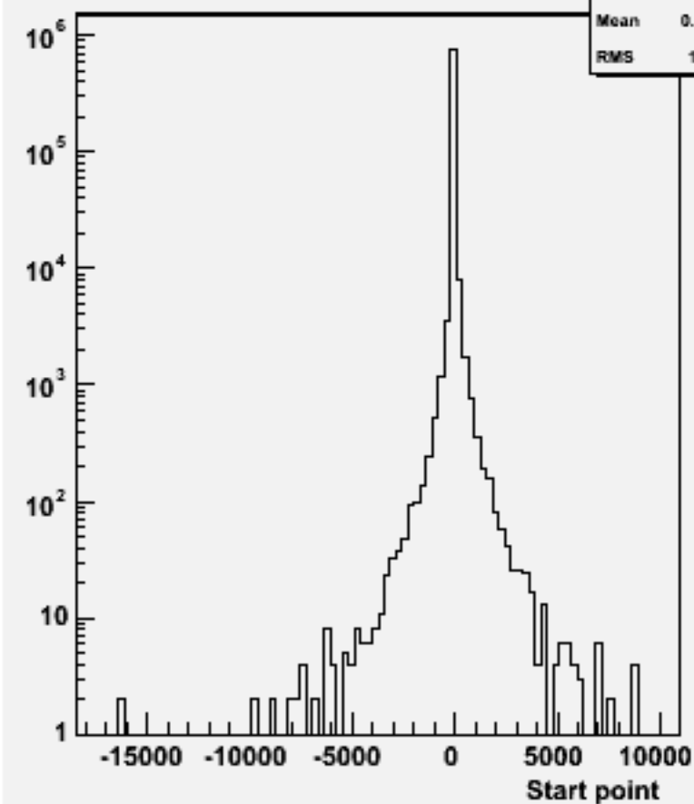
Start point Z : w101657 uuude1n1_o
