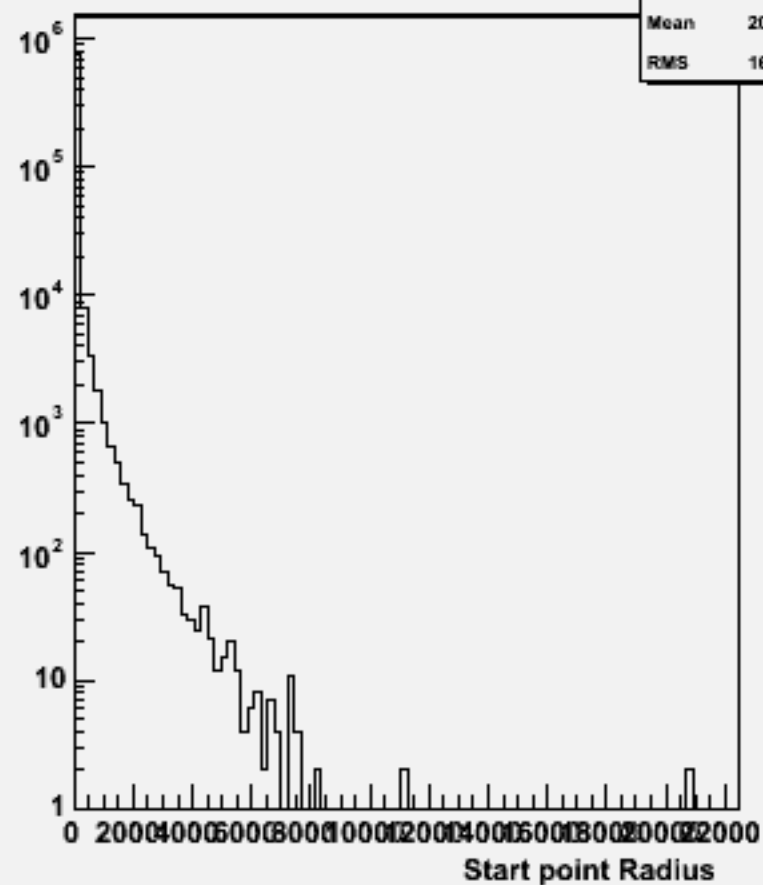
Start point R : w101657 uuude1n1_o
