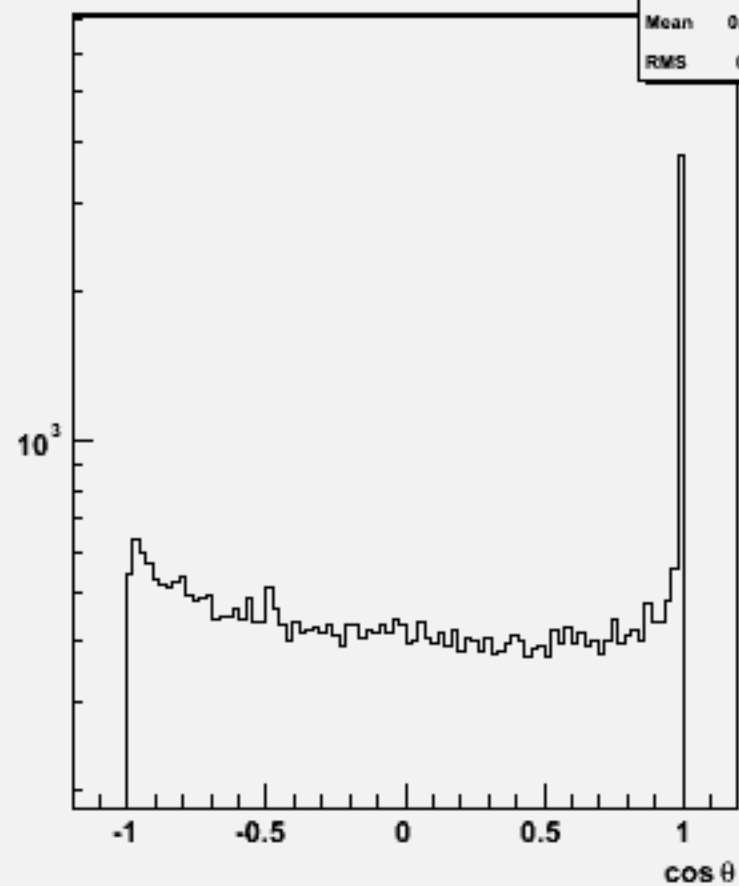
Jet cos \theta (All jets)w101657 uuude1n1_o
