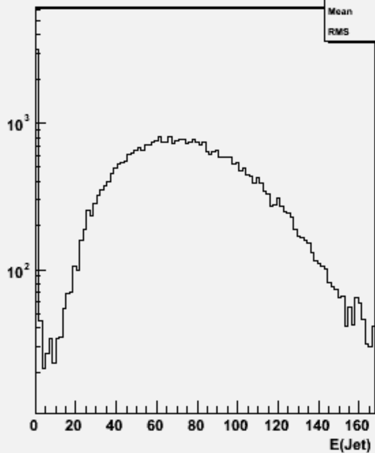
Jet energies(All jets)w101657 uuude1n1_o
