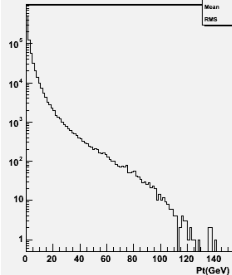
Particle Pt : w101656 uuude1n1_o
