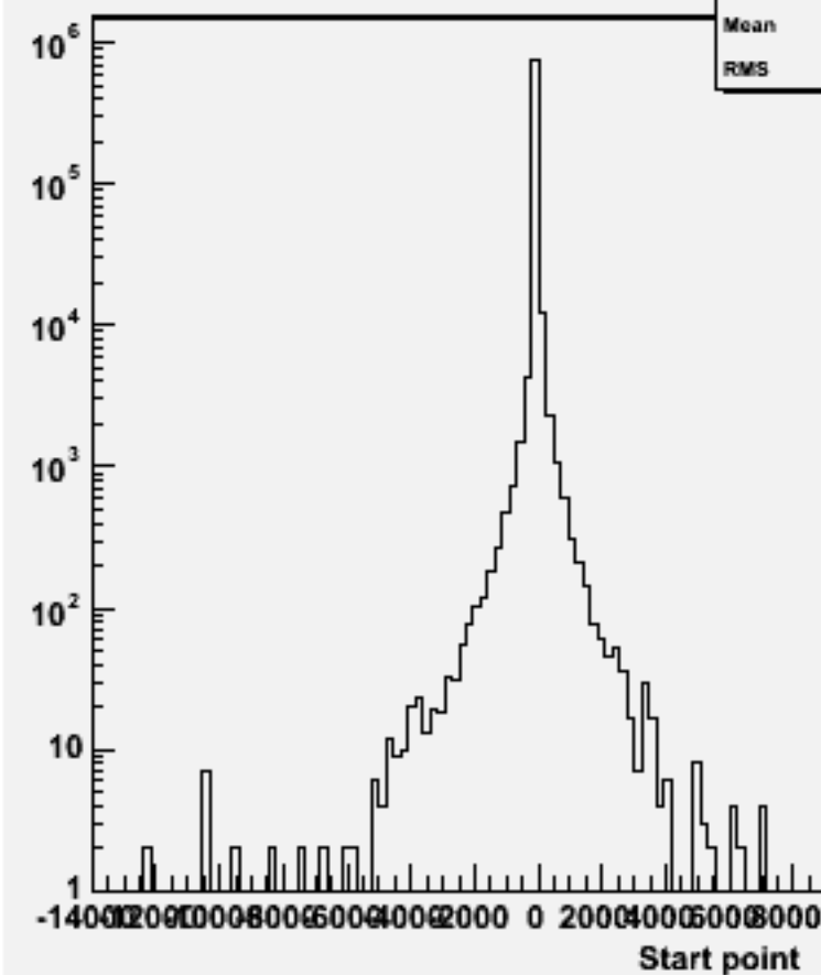
Start point Z : w101656 uuude1n1_o
