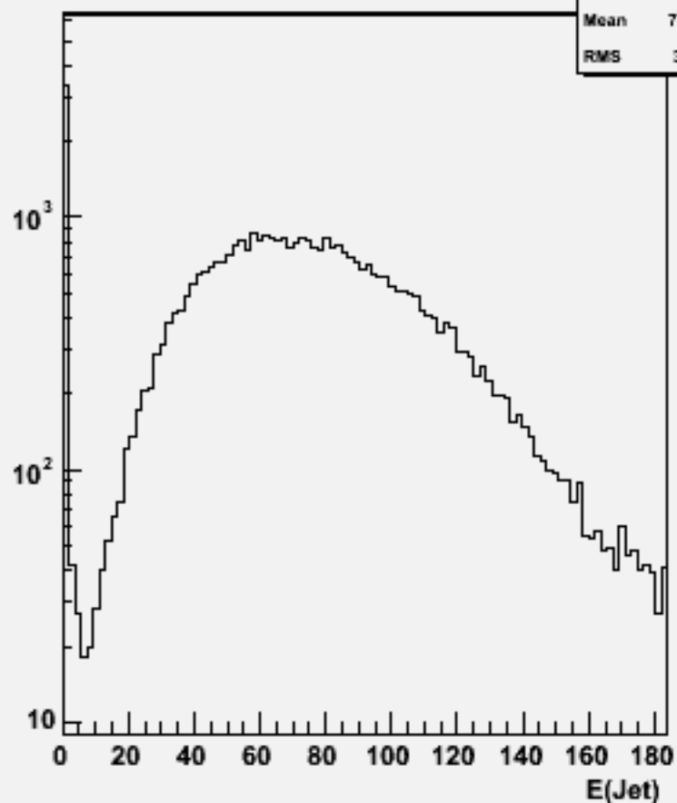
Jet energies(All jets)w101656 uuude1n1_o
