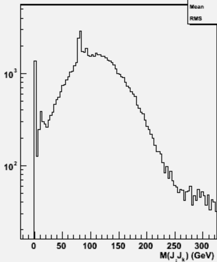
2jets mass(All comb)w101656 uuude1n1_o
