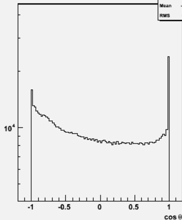
Particle cos \theta : w101656 uuude1n1_o
