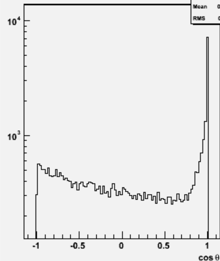
Jet cos \theta (All jets)w101656 uuude1n1_o
