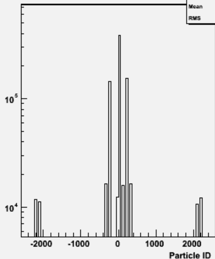
Particle ID : w101656 uuude1n1_o
