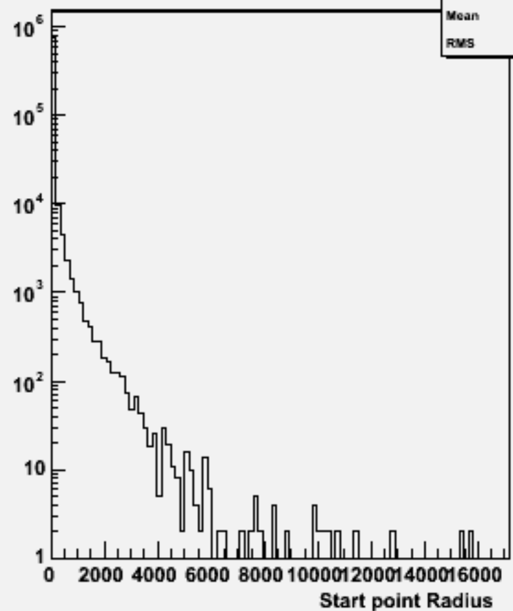
Start point R : w101656 uuude1n1_o
