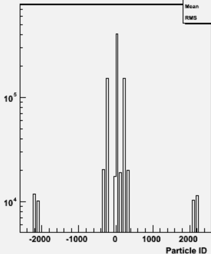
Particle ID : w101653 uun3e3sc_o
