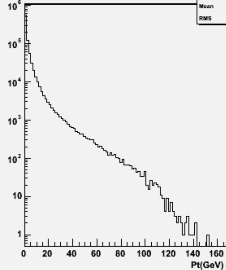
Particle Pt : w101652 uun3e3sc_o
