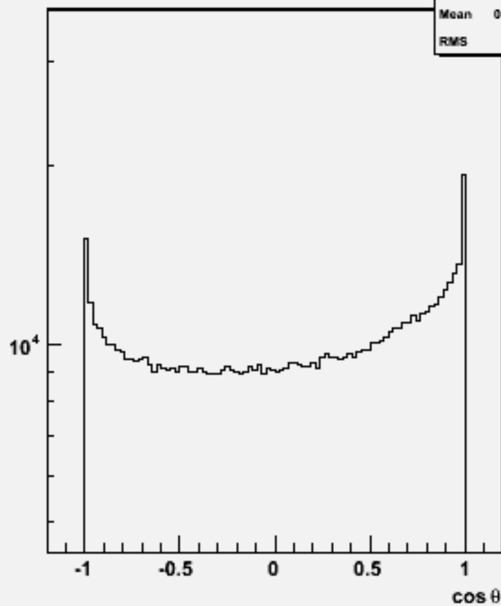
Particle cos \theta : w101652 uun3e3sc_o
