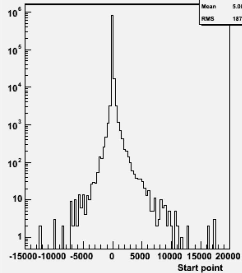
Start point Z : w101652 uun3e3sc_o
