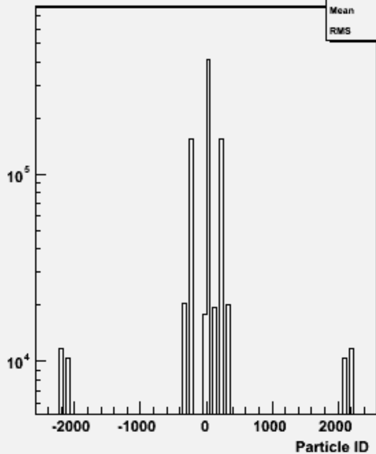
Particle ID : w101652 uun3e3sc_o
