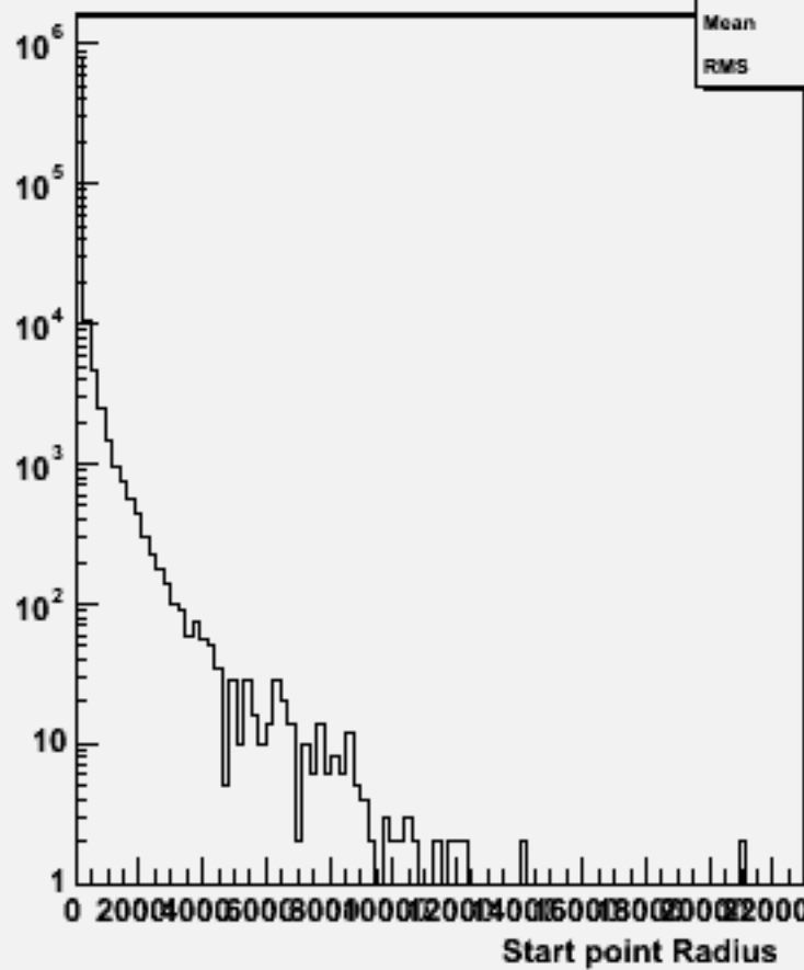
Start point R : w101652 uun3e3sc_o
