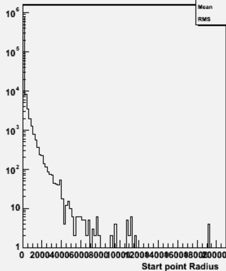
Start point R : w101648 uun3e3du_o
