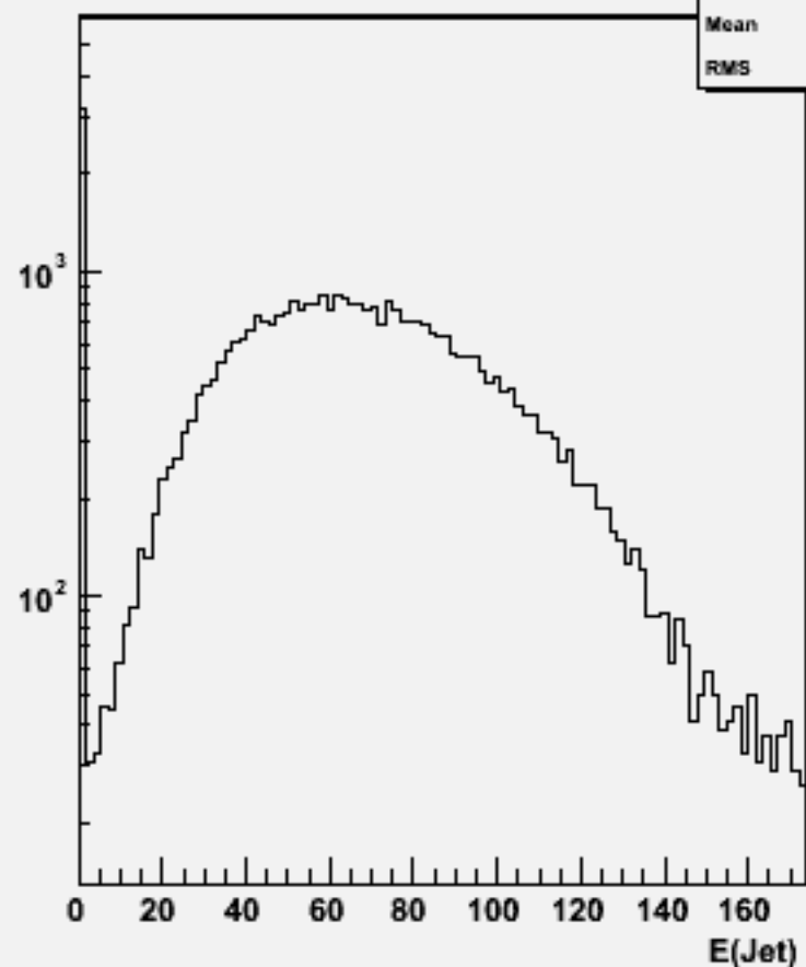
Jet energies(All jets)w101648 uun3e3du_o
