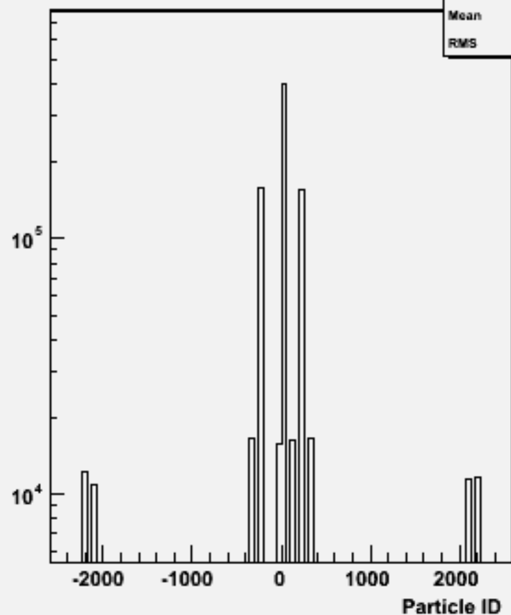
Particle ID : w101648 uun3e3du_o
