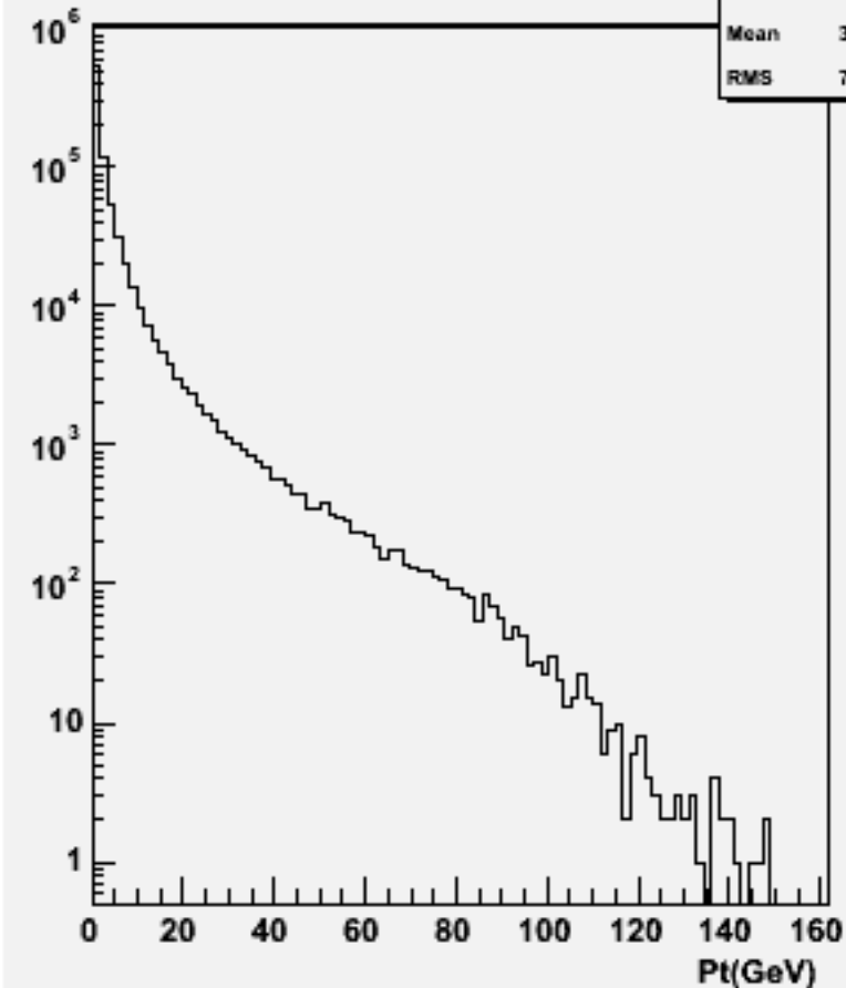
Particle Pt : w101648 uun3e3du_o
