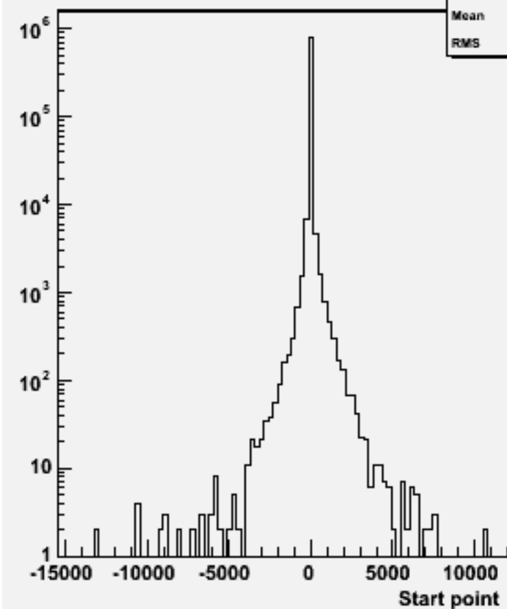
Start point Z : w101648 uun3e3du_o
