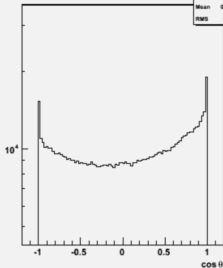
Particle cos \theta : w101648 uun3e3du_o
