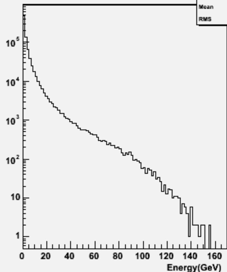
Particle Energy : w101648 uun3e3du_o
