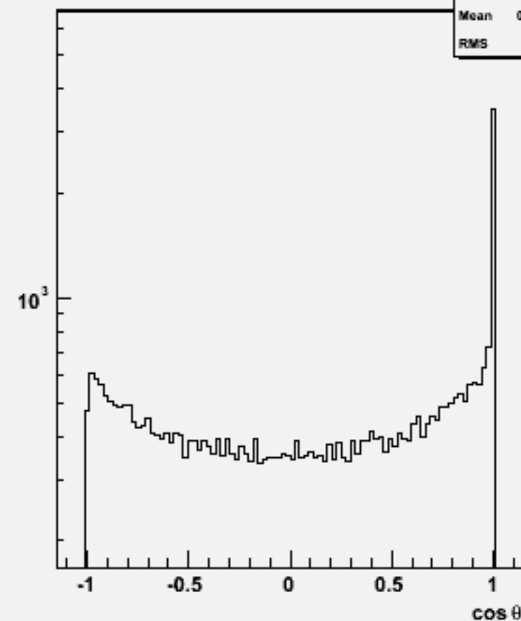
Jet cosθ (All jets)w101648 uun3e3du_o
