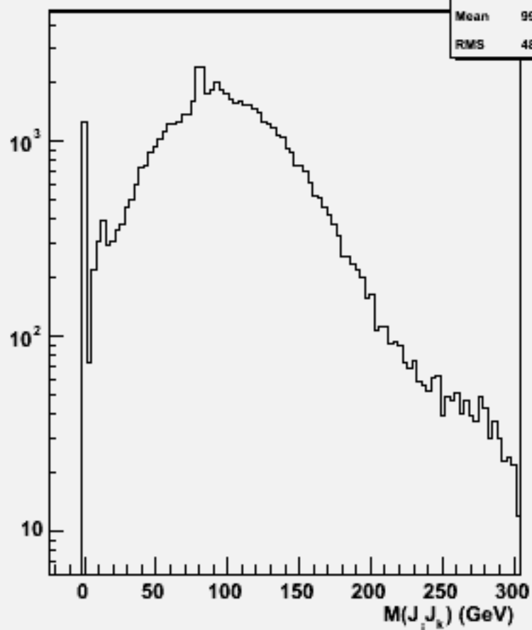
2jets mass(All comb)w101648 uun3e3du_o
