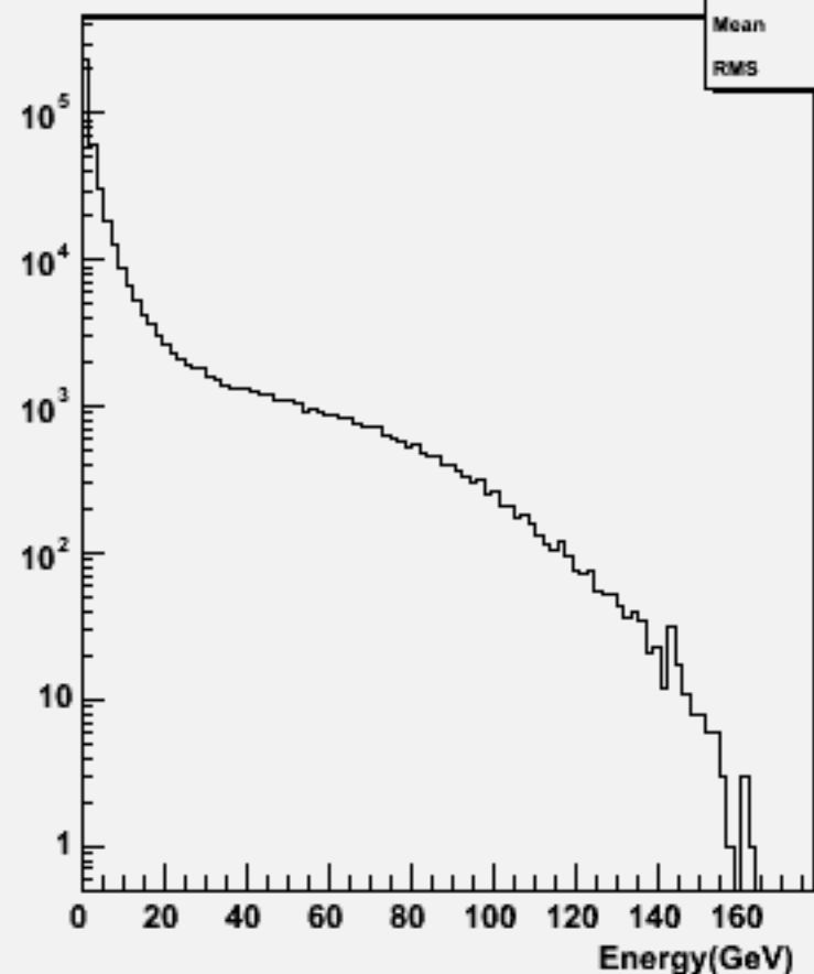
Start point R : w101641 uun3e3e2n2_o
