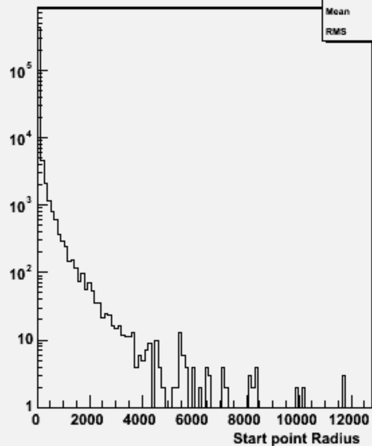
Start point R : w101641 uun3e3e2n2_o
