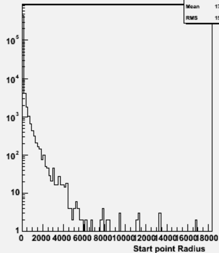
Start point R : w101640 uun3e3e2n2_o
