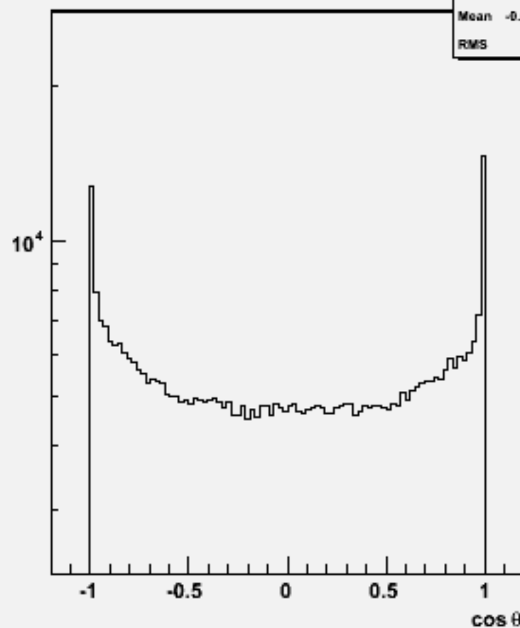
Particle cosθ : w101640 uun3e3e2n2_o
