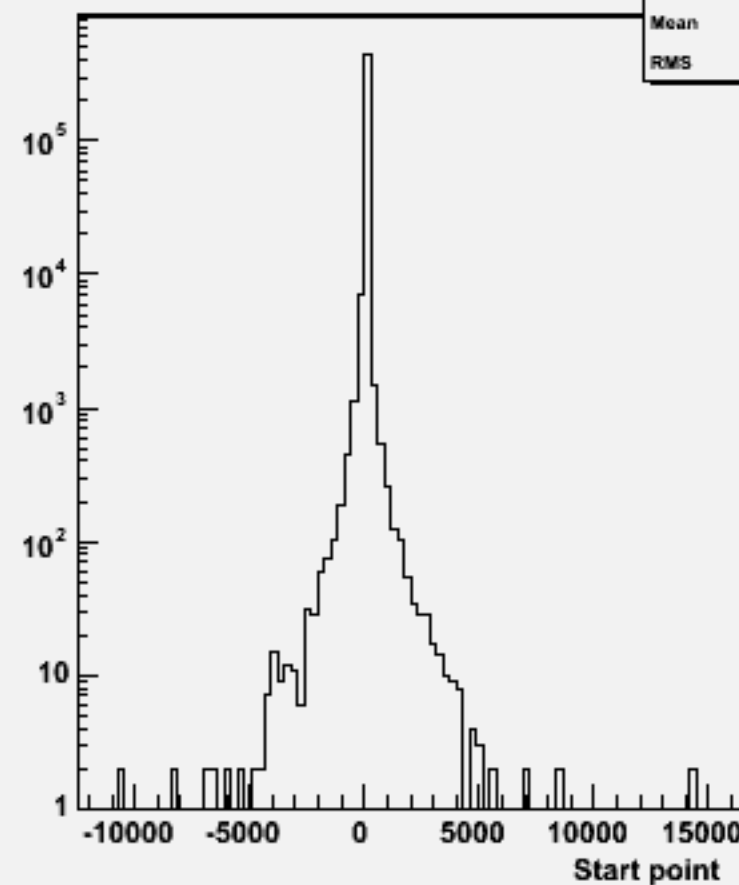
Start point Z : w101640 uun3e3e2n2_o
