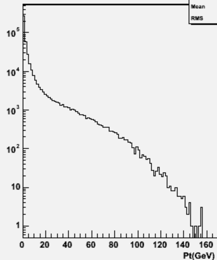
Start point Z : w101640 uun3e3e2n2_o
