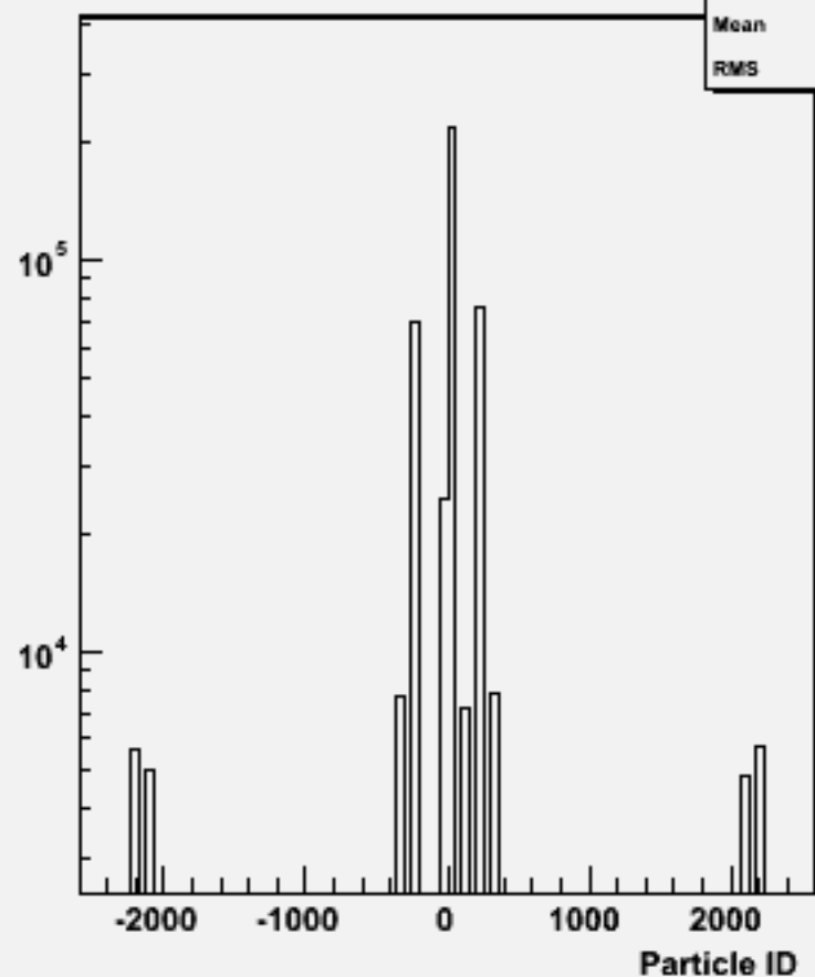
Particle ID : w101637 uun3e3e1n1_o
