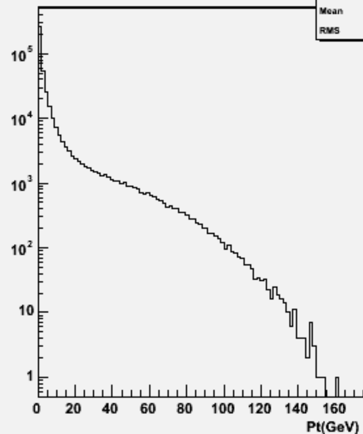
Particle Pt : w101637 uun3e3e1n1_o
