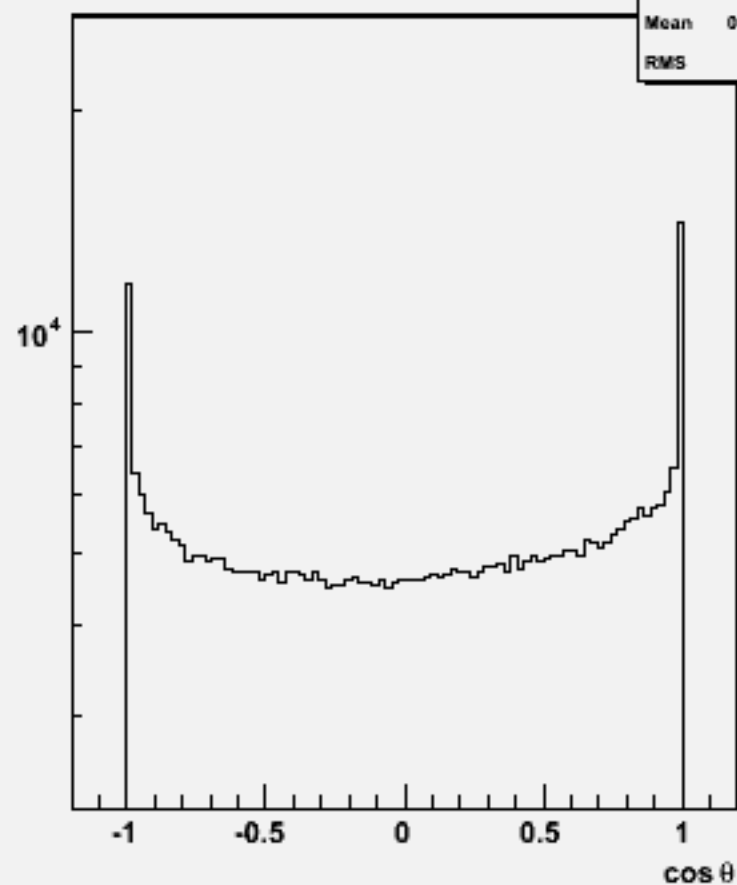
Particle cos \theta : w101637 uun3e3e1n1_o
