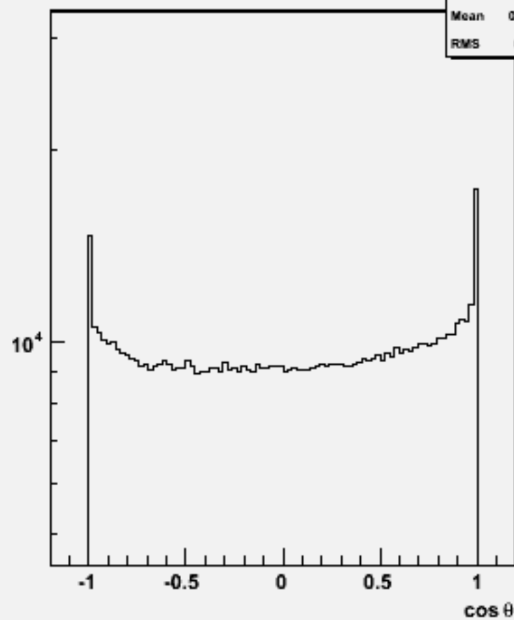
Particle cos \theta : w101633 uun2e2sc_o
