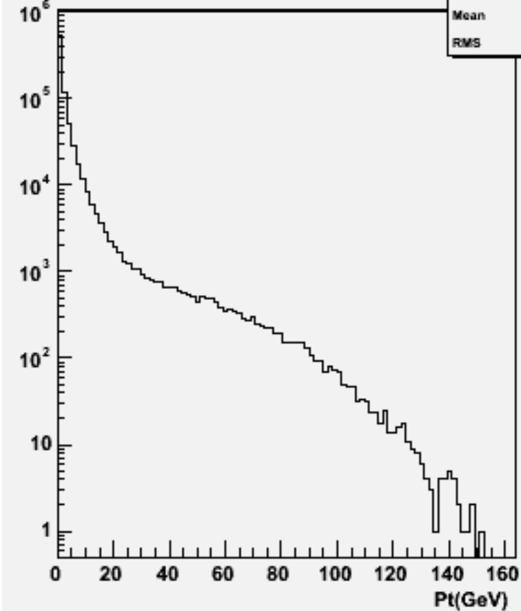
Particle Pt : w101633 uun2e2sc_o
