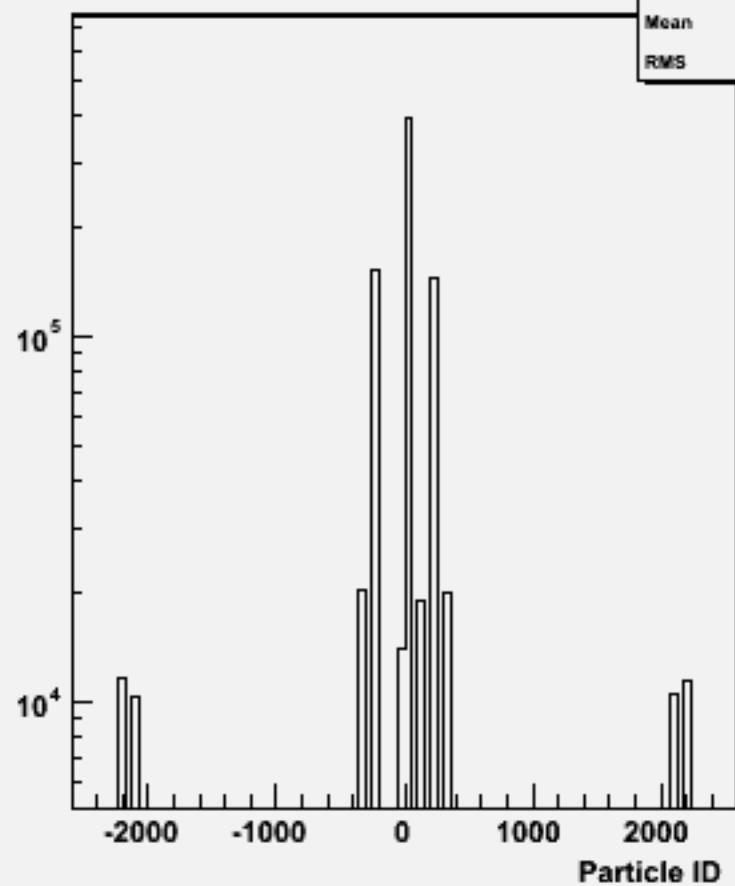
Particle ID : w101633 uun2e2sc_o
