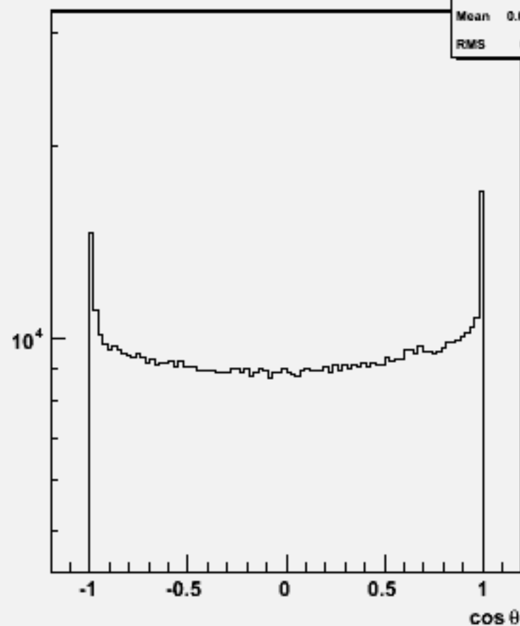
Particle cos \theta : w101629 uun2e2du_o
