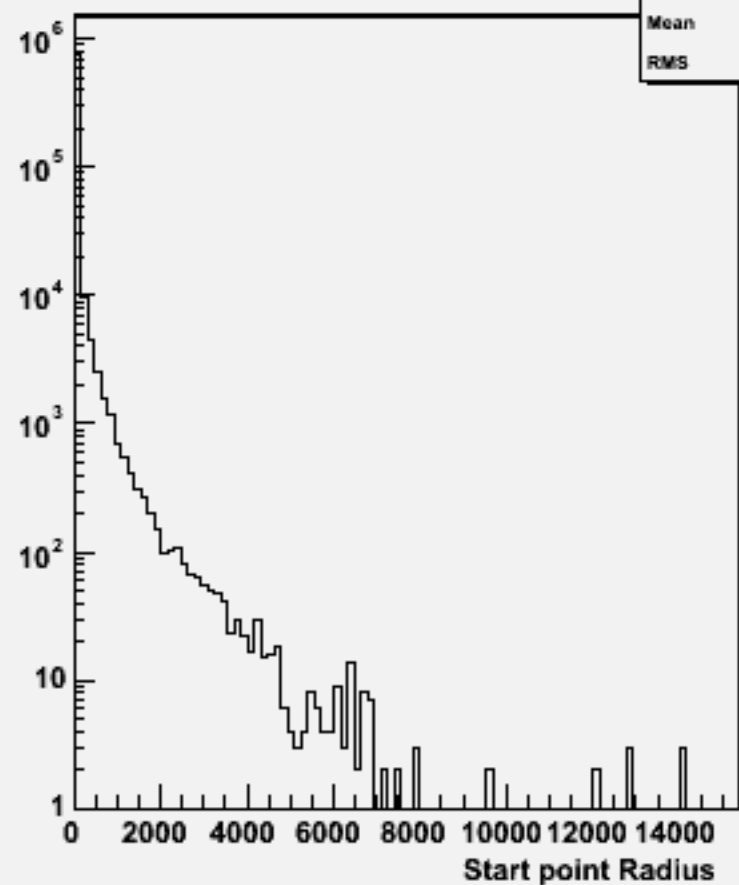
Start point R : w101629 uun2e2du_o
