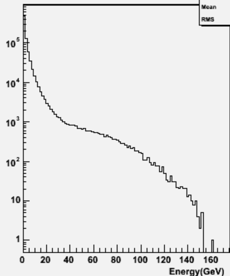
Particle Energy : w101629 uun2e2du_o
