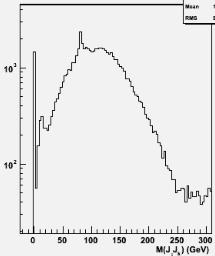
2jets mass(All comb)w101628 uun2e2du_o
