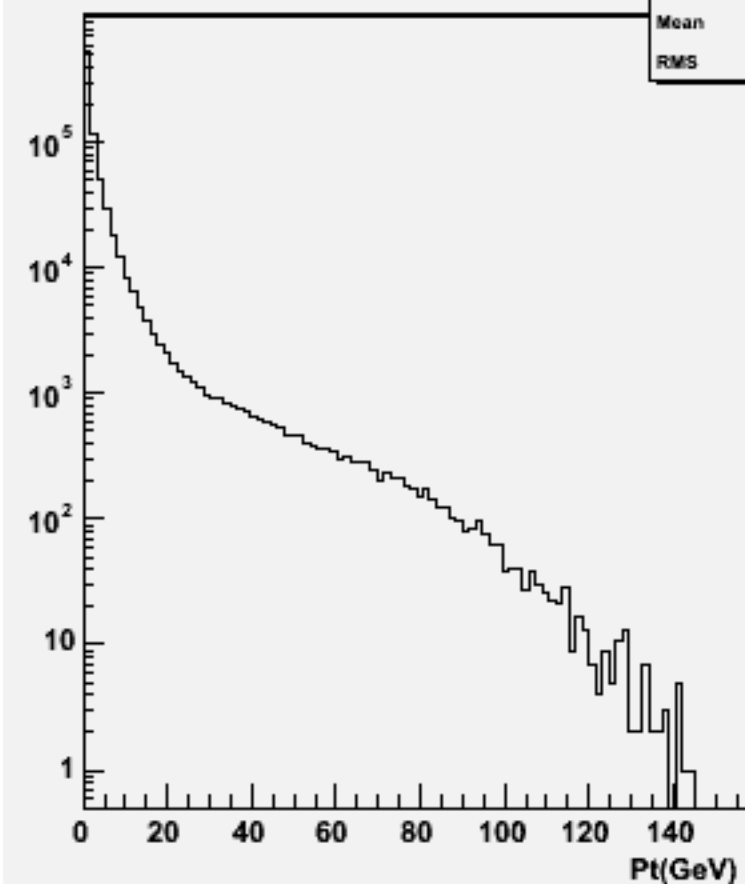
Particle Pt : w101628 uun2e2du_o
