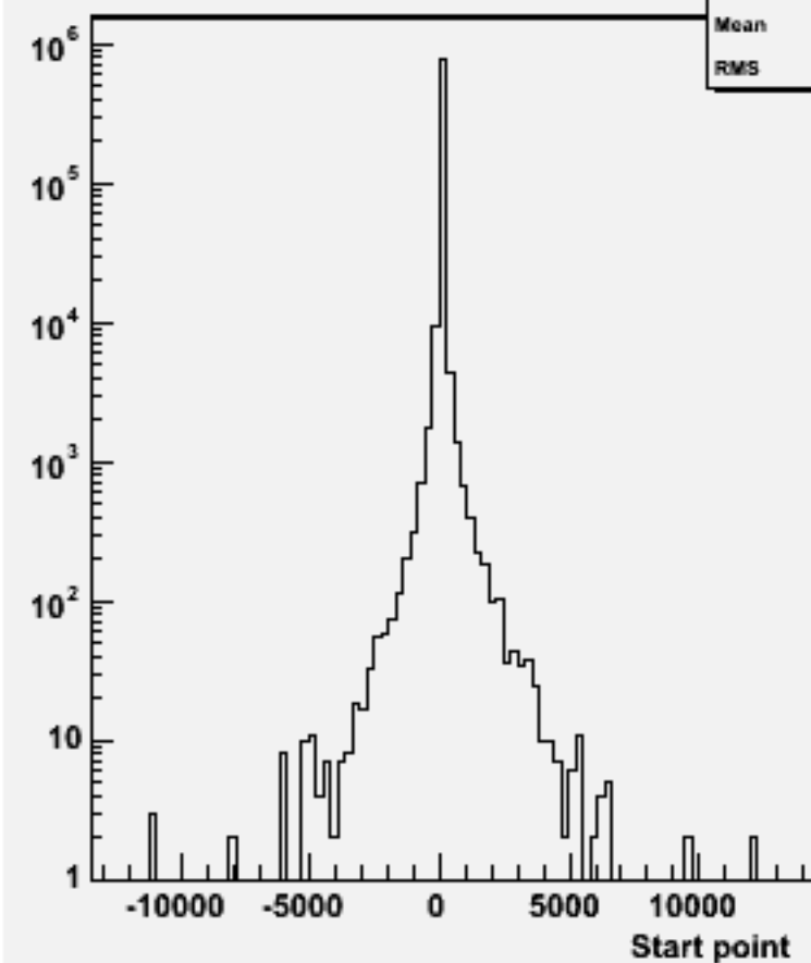
Start point Z : w101628 uun2e2du_o
