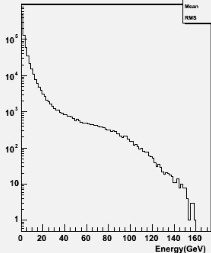
Particle Energy : w101628 uun2e2du_o
