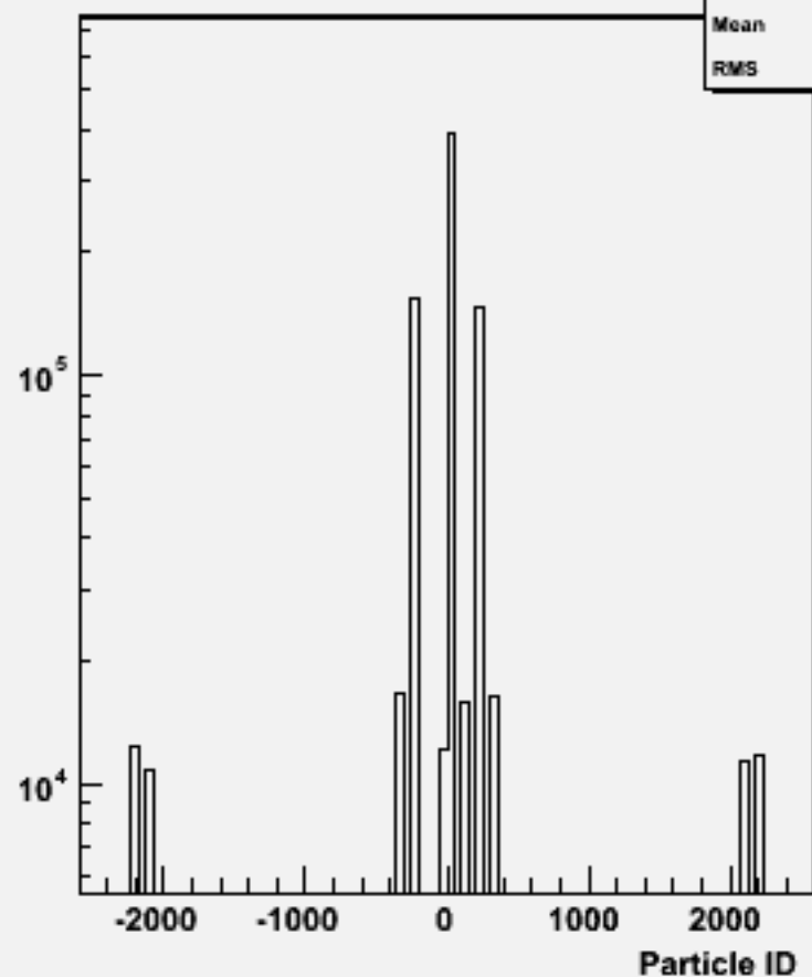
Particle ID : w101628 uun2e2du_o
