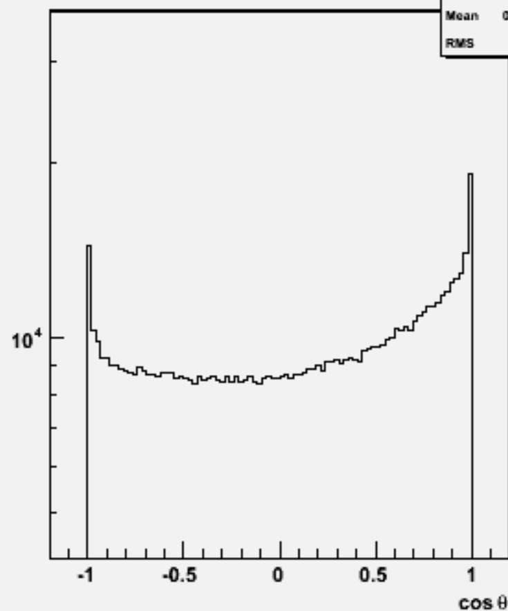
Particle cos \theta : w101628 uun2e2du_o
