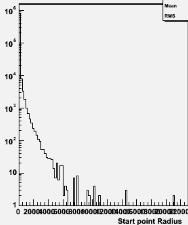
Start point R : w101628 uun2e2du_o
