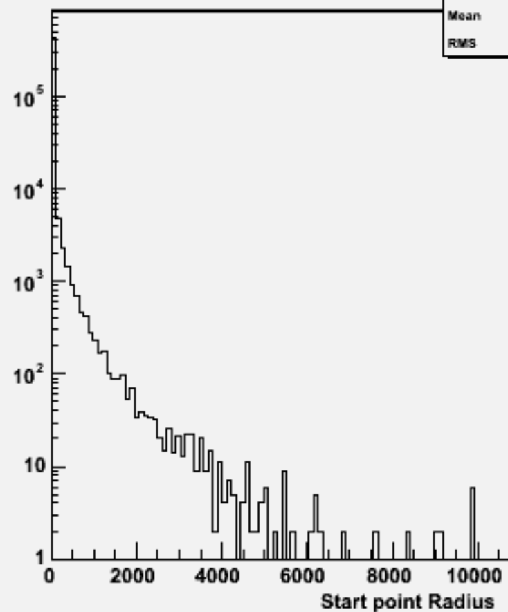
Start point R : w101625 uun2e2e3n3_o
