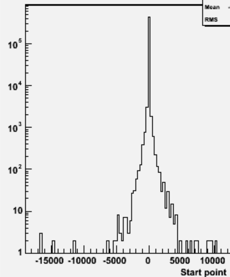
Start point Z : w101625 uun2e2e3n3_o
