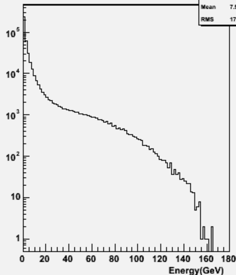
Start point R : w101625 uun2e2e3n3_o
