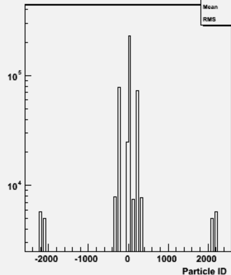
Particle ID : w101624 uun2e2e3n3_o
