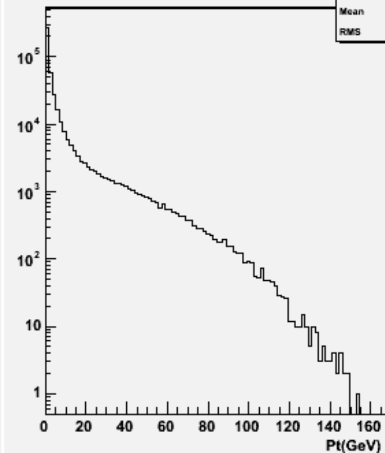
Particle Pt : w101624 uun2e2e3n3_o
