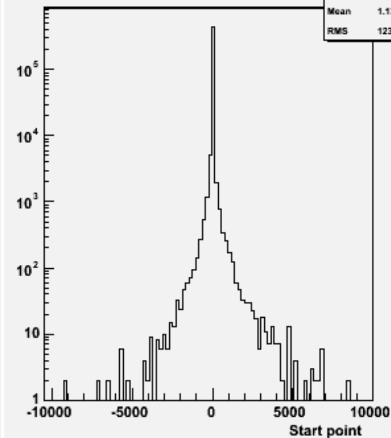
Start point Z : w101624 uun2e2e3n3_o
