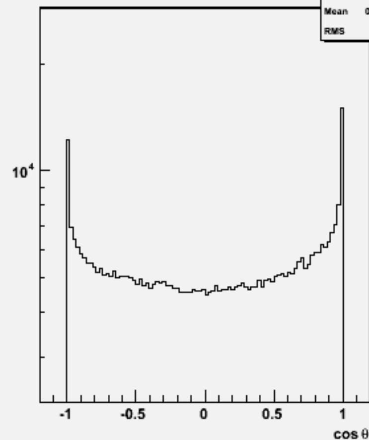
Particle cos \theta : w101624 uun2e2e3n3_o
