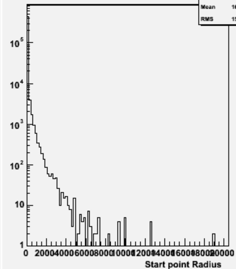
Start point R : w101624 uun2e2e3n3_o
