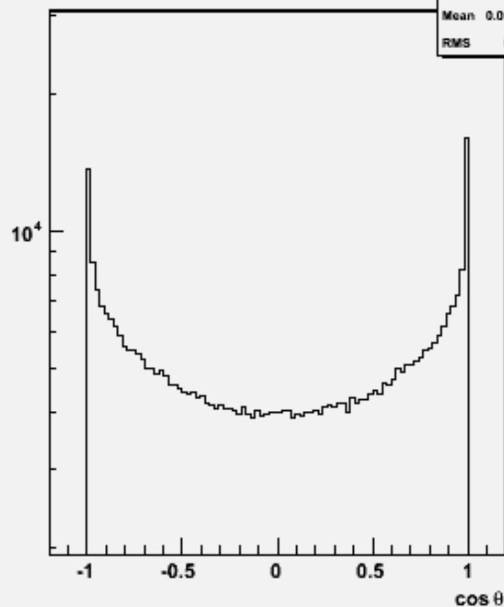
Particle \cos\theta : w101621 uun2e2e2n2_o
