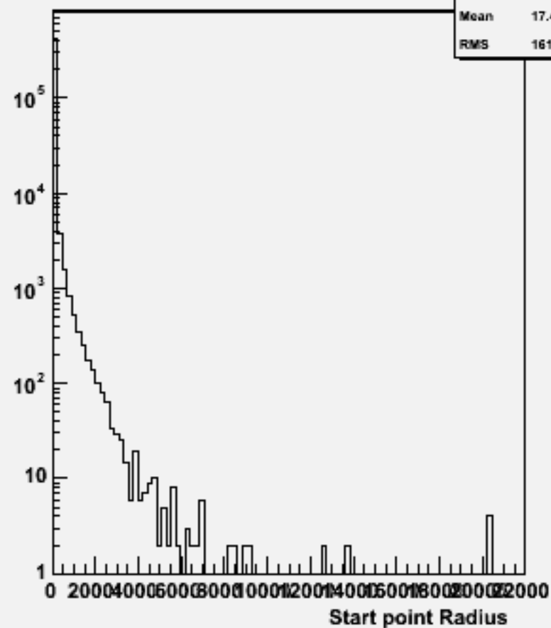
Start point R : w101621 uun2e2e2n2_o
