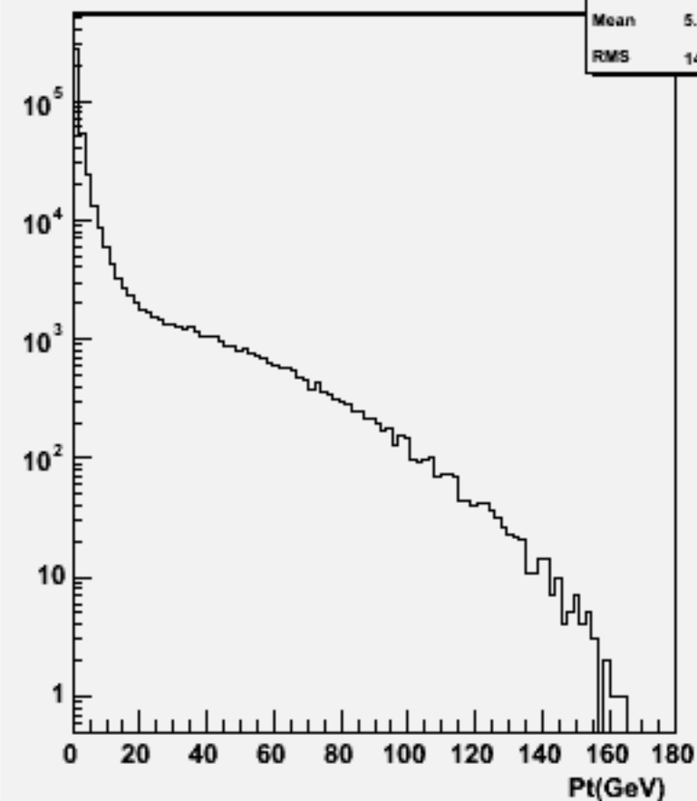
Particle Pt : w101621 uun2e2e2n2_o
