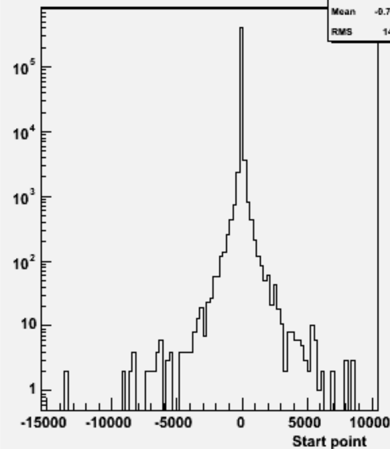
Start point Z : w101621 uun2e2e2n2_o
