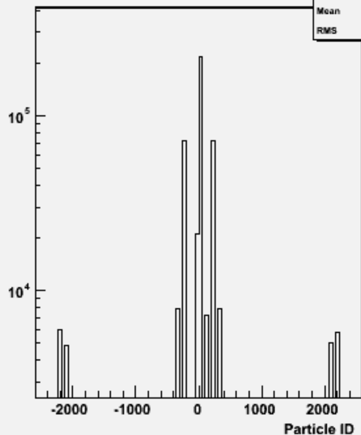
Particle ID : w101621 uun2e2e2n2_o
