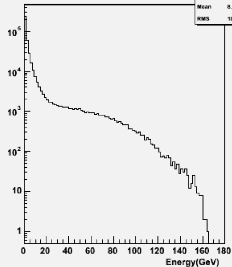
Start point R : w101620 uun2e2e2n2_o
