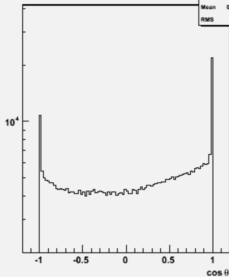
Particle cos \theta : w101616 uun2e2e1n1_o
