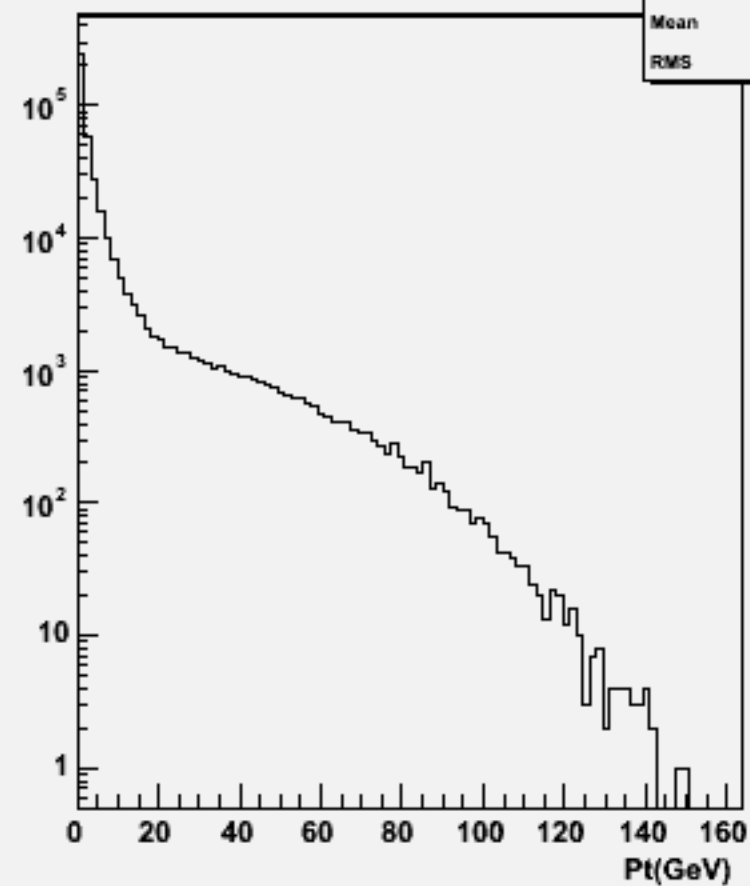
Particle Pt : w101616 uun2e2e1n1_o
