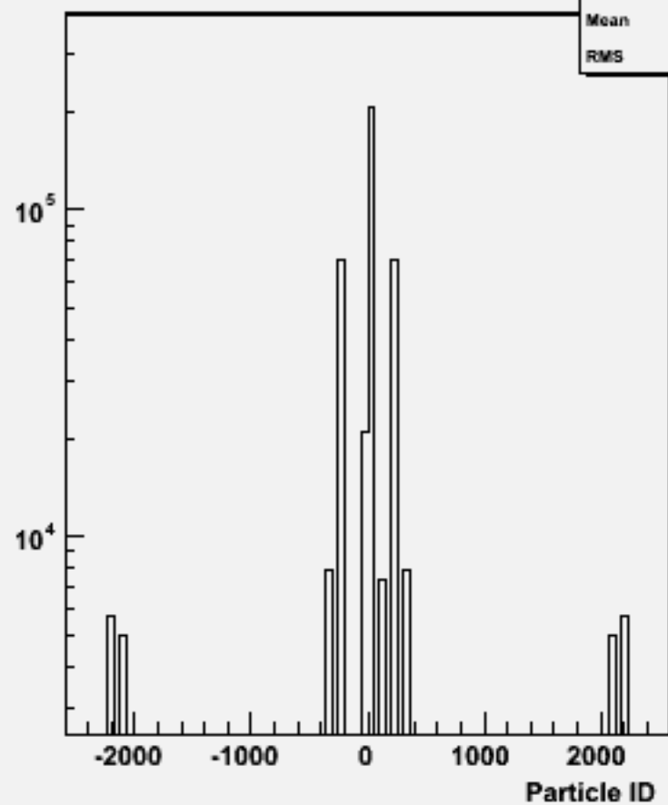
Particle ID : w101616 uun2e2e1n1_o
