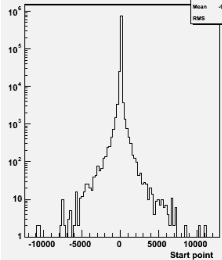
Start point Z : w101613 uun1e1sc_o
