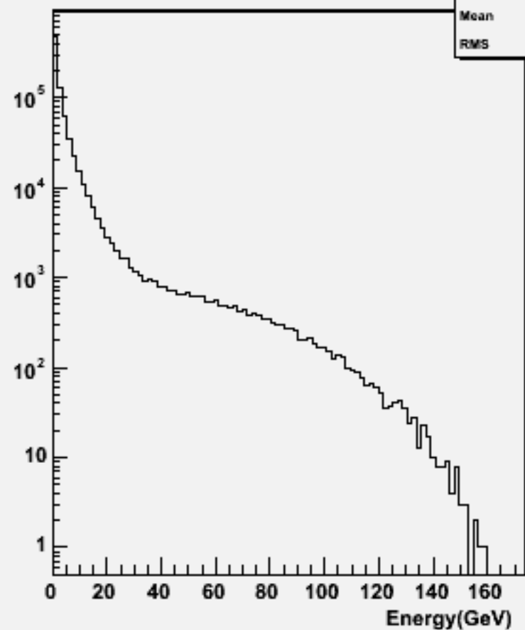
Particle Energy : w101613 uun1e1sc_o
