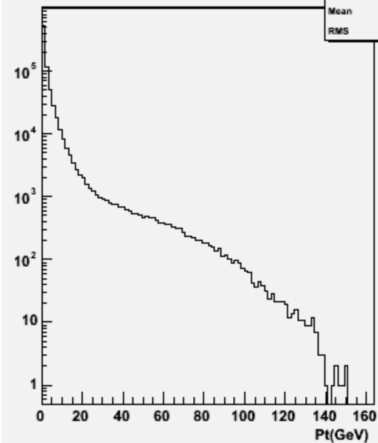
Particle Pt : w101613 uun1e1sc_o
