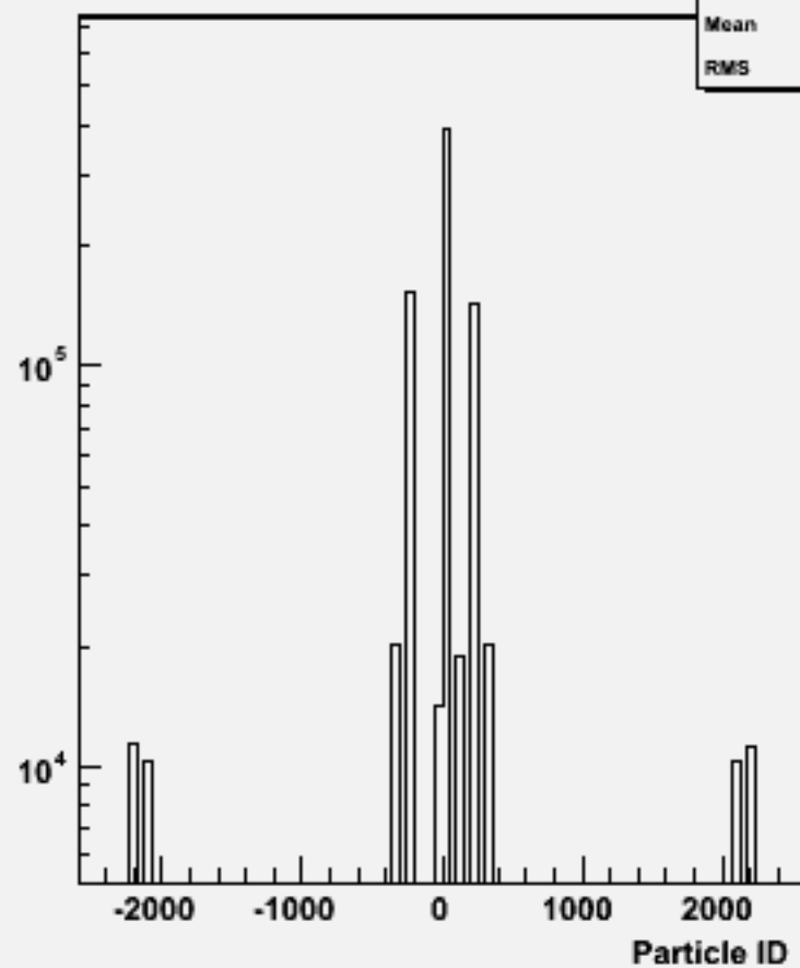
Particle ID : w101613 uun1e1sc_o
