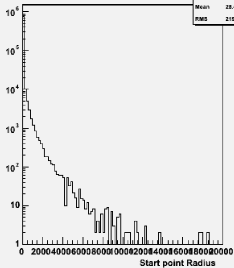
Start point R : w101613 uun1e1sc_o
