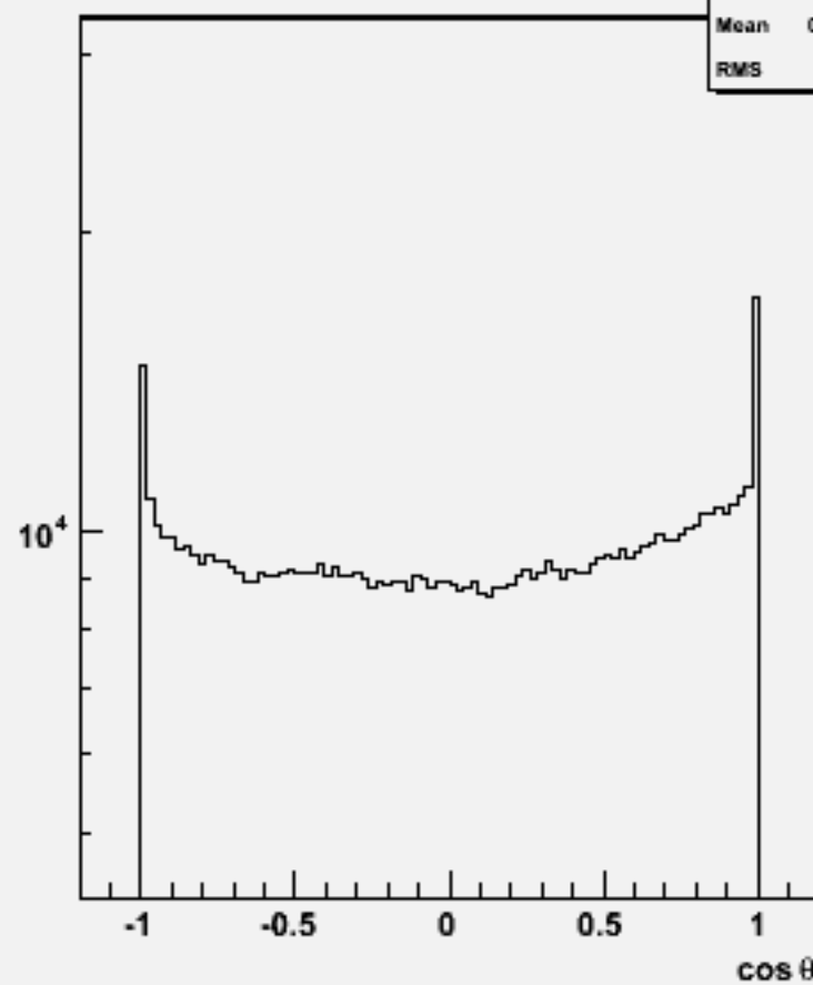
Particle cos \theta : w101613 uun1e1sc_o
