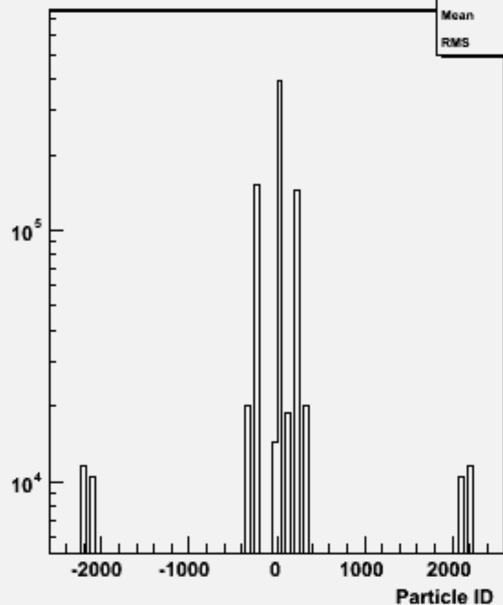
Particle ID : w101612 uun1e1sc_o
