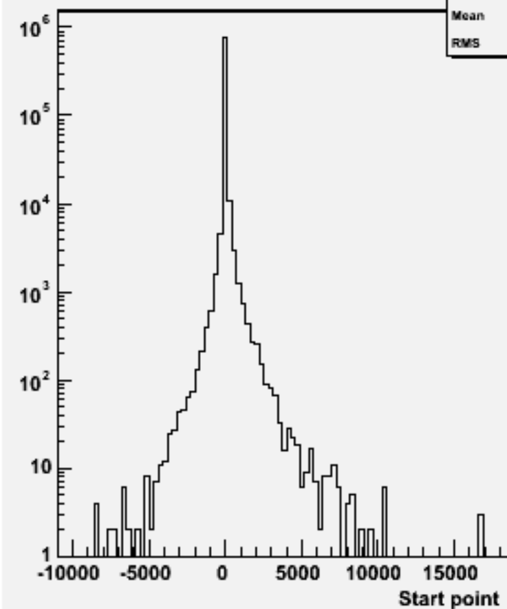
Start point Z : w101612 uun1e1sc_o
