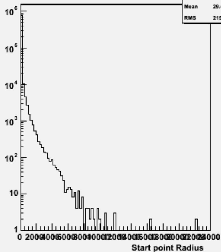
Start point R : w101612 uun1e1sc_o
