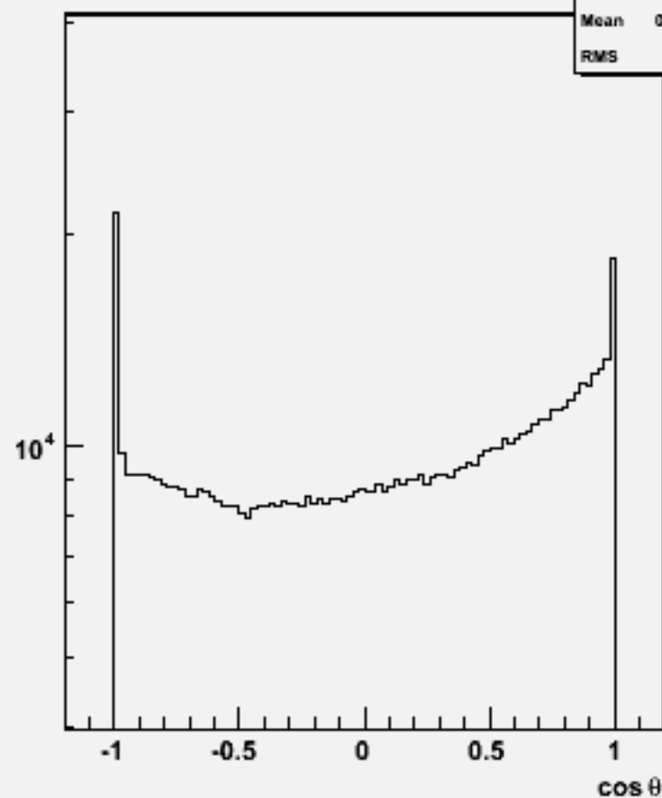
Particle cos \theta : w101612 uun1e1sc_o
