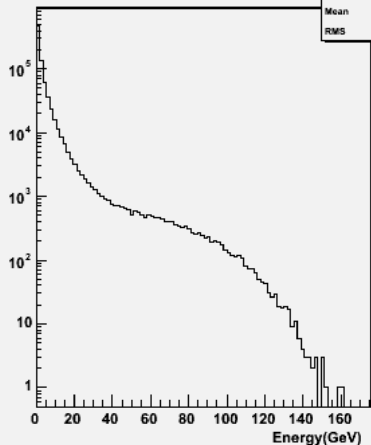
Particle Energy : w101612 uun1e1sc_o
