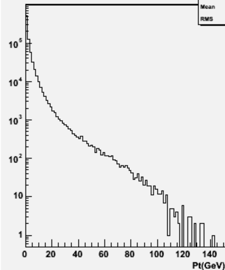
Particle Pt : w101612 uun1e1sc_o
