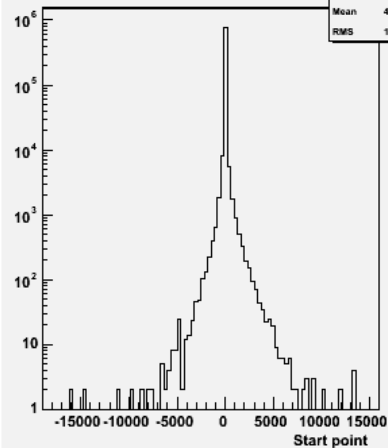
Start point Z : w101611 uun1e1sc_o
