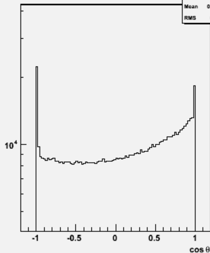
Particle cos \theta : w101611 uun1e1sc_o
