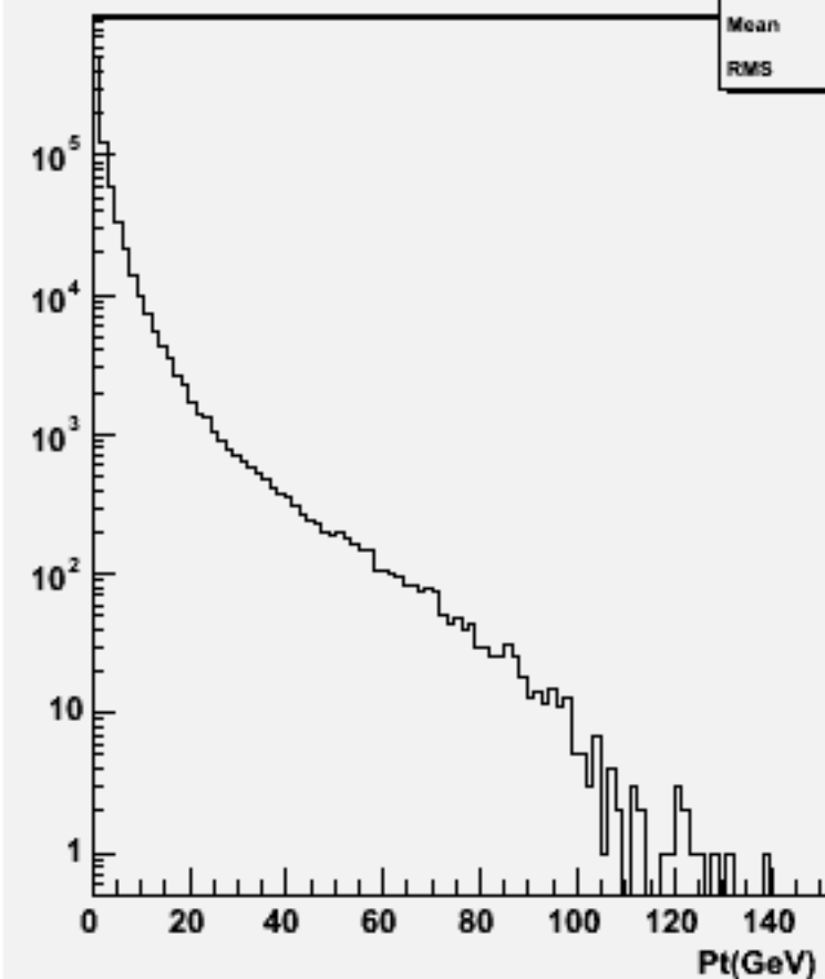
Particle Pt : w101611 uun1e1sc_o
