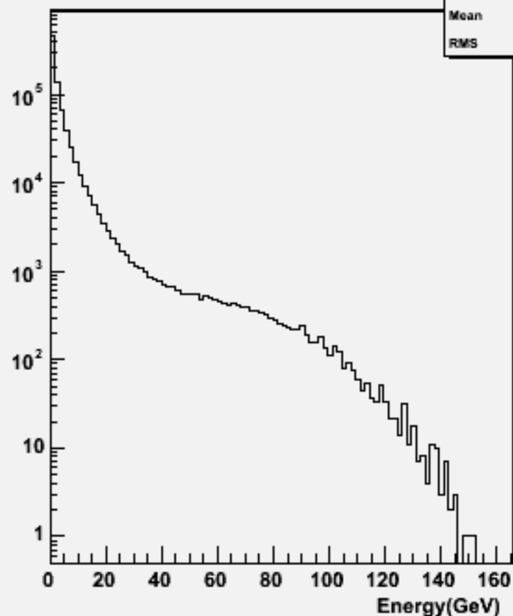
Particle Energy : w101611 uun1e1sc_o
