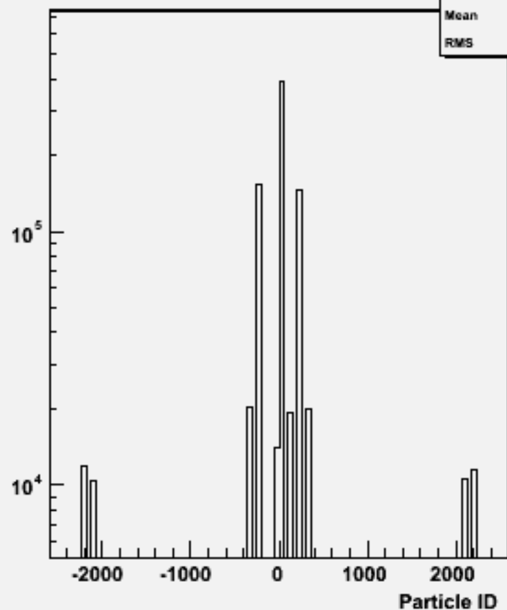
Particle ID : w101611 uun1e1sc_o
