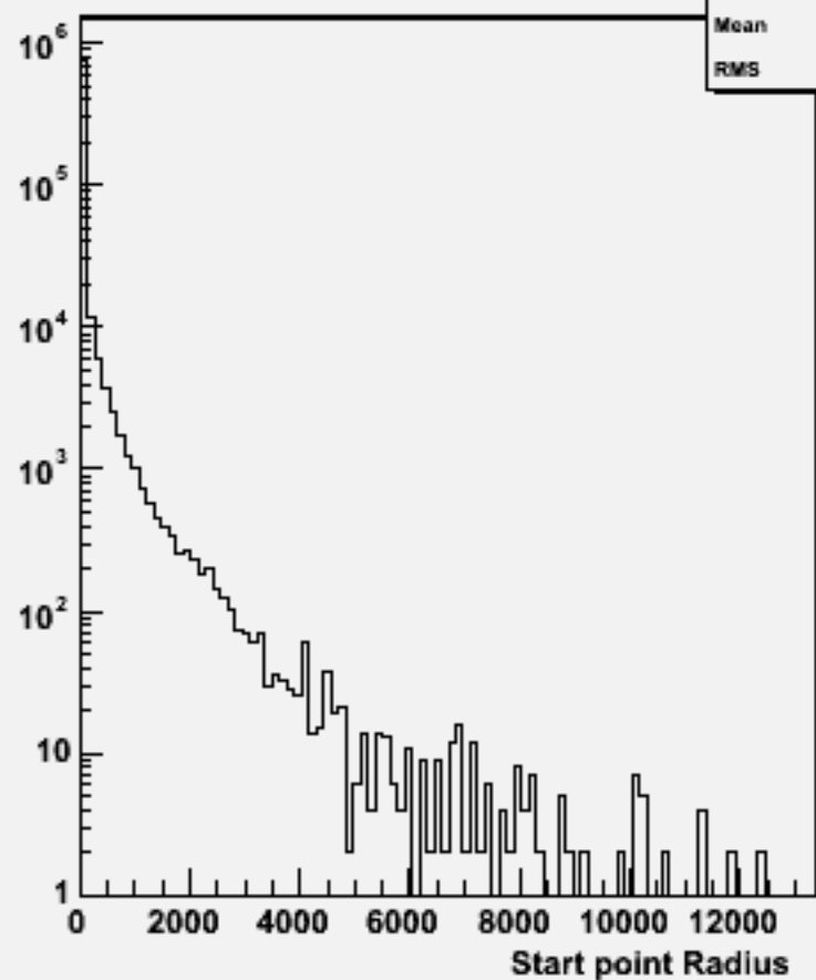
Start point R : w101611 uun1e1sc_o
