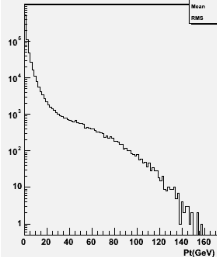
Particle Pt : w101609 uun1e1du_o
