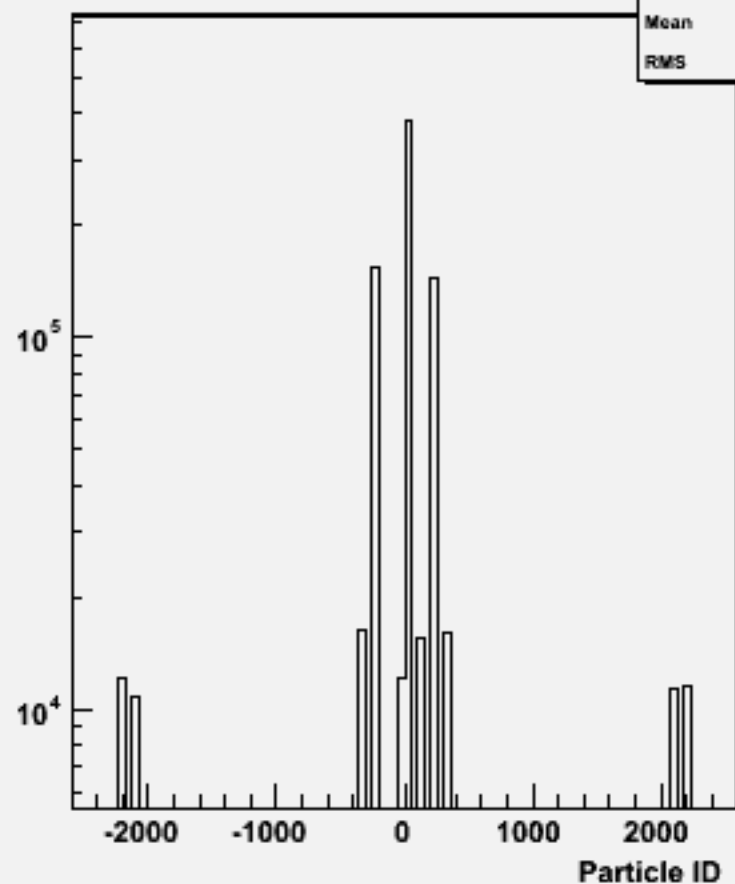
Particle ID : w101609 uun1e1du_o
