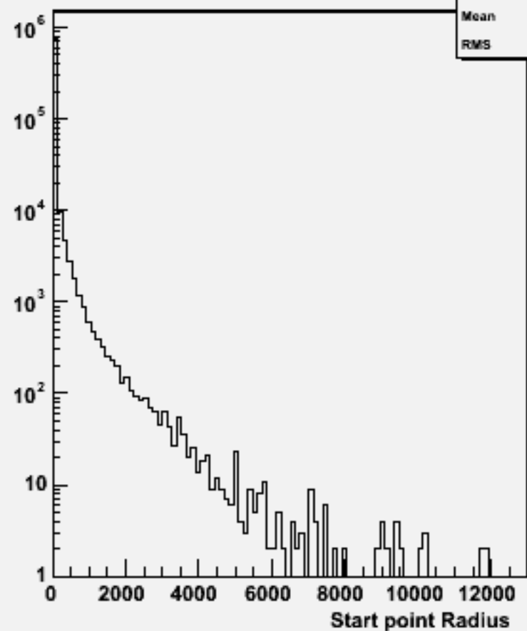
Start point R : w101609 uun1e1du_o
