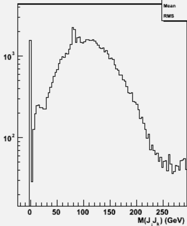
2jets mass(All comb)w101609 uun1e1du_o
