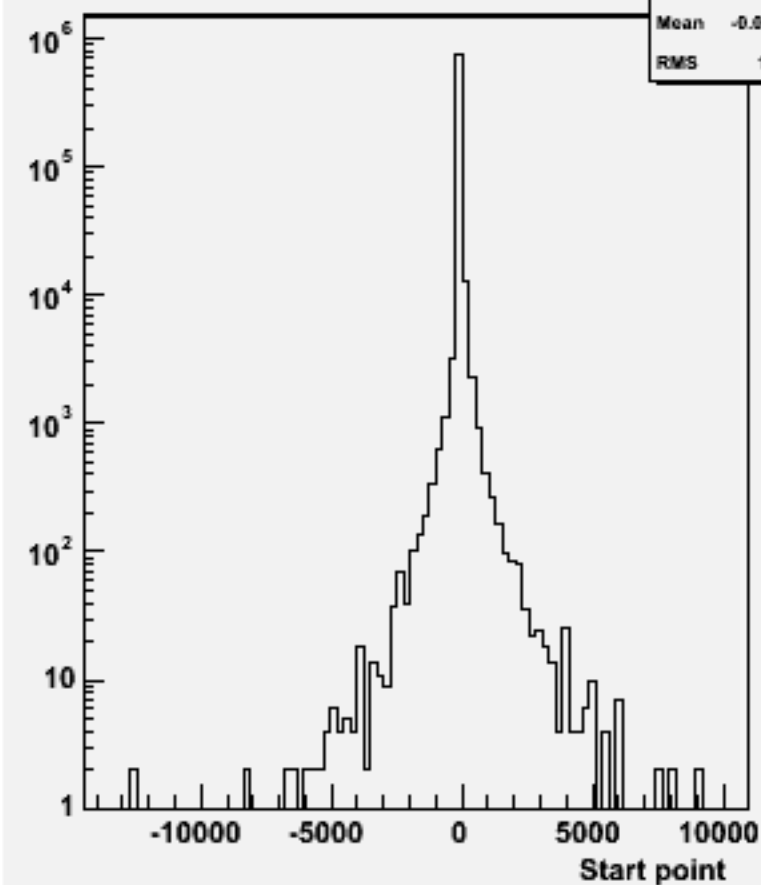
Start point Z : w101609 uun1e1du_o
