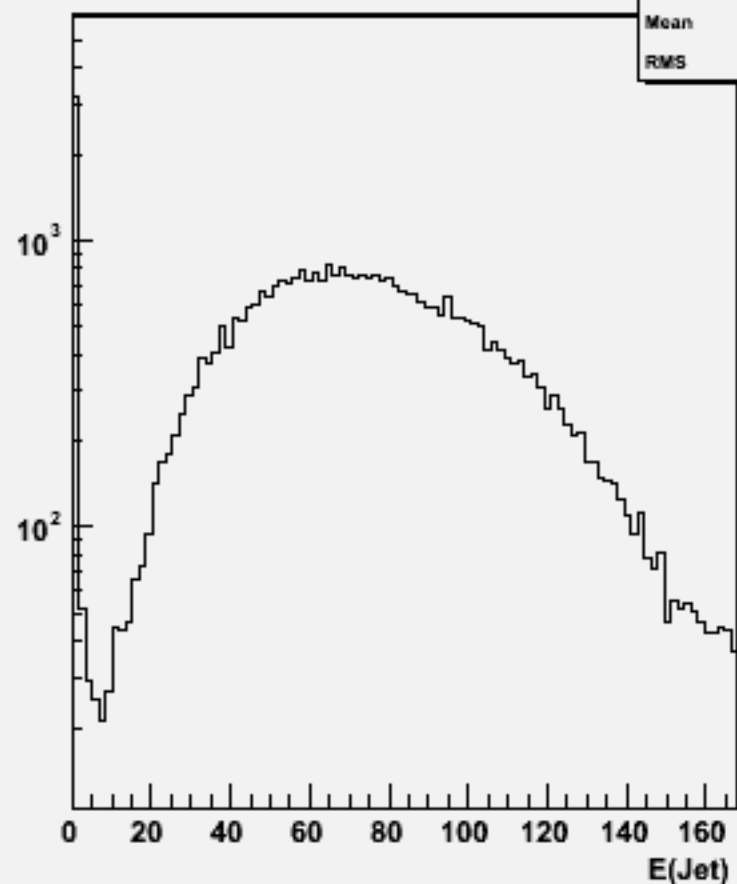
Jet energies(All jets)w101609 uun1e1du_o
