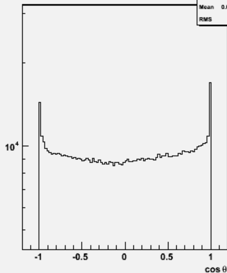
Particle cos \theta : w101609 uun1e1du_o
