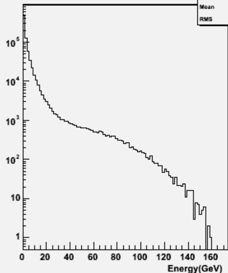
Particle Energy : w101609 uun1e1du_o
