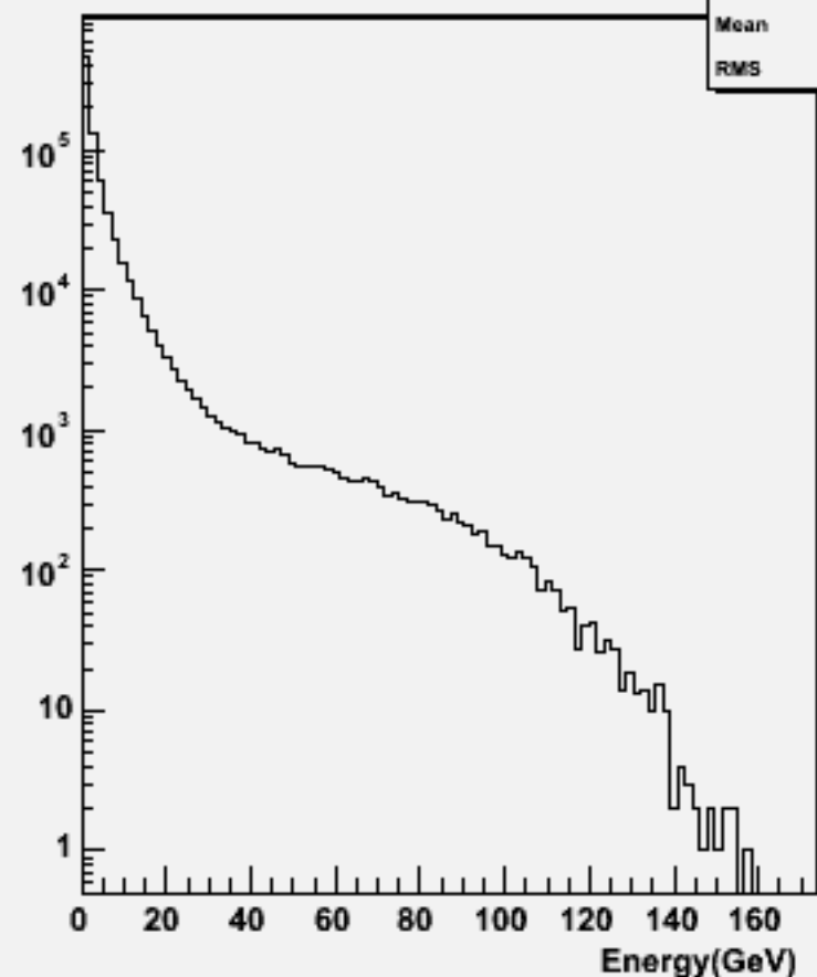
Particle Energy : w101608 uun1e1du_o
