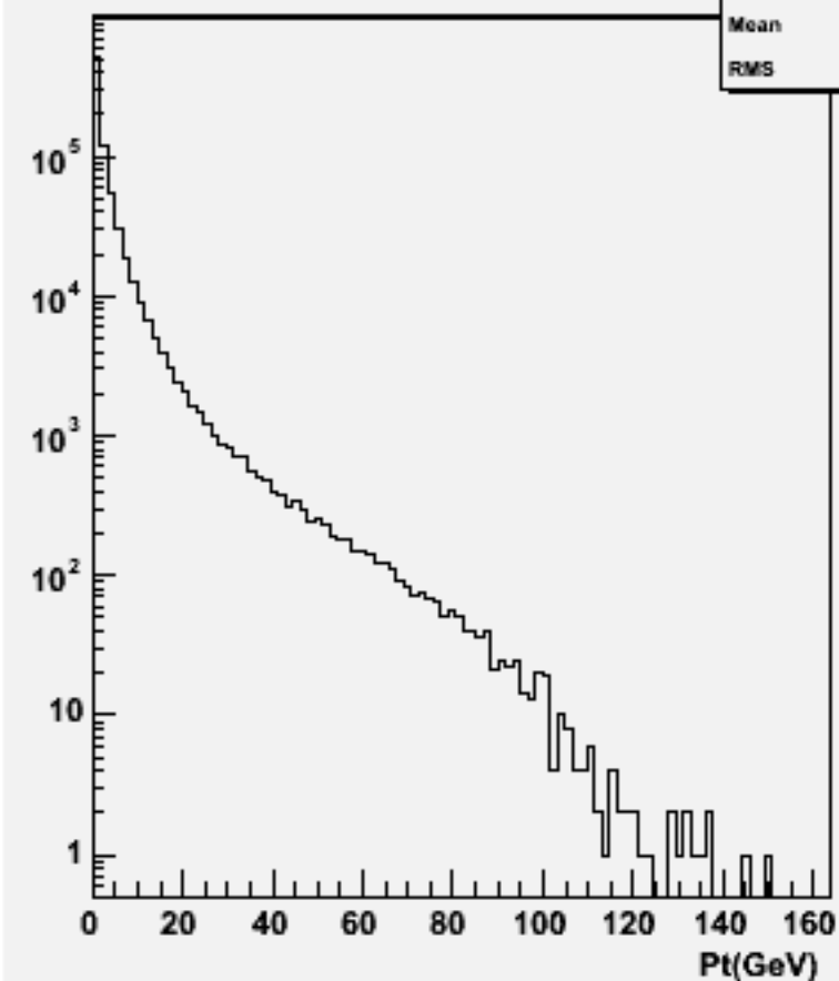
Particle Pt : w101608 uun1e1du_o
