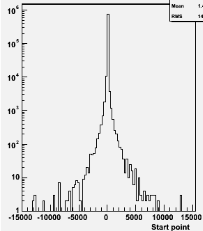
Start point Z : w101608 uun1e1du_o
