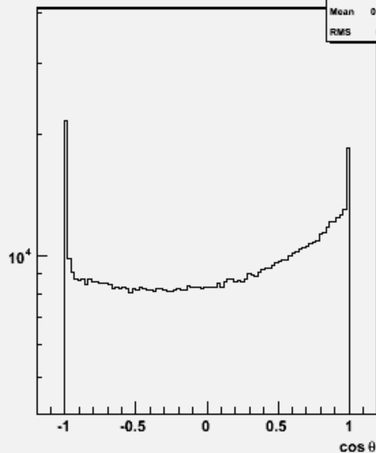
Particle cos \theta : w101608 uun1e1du_o
