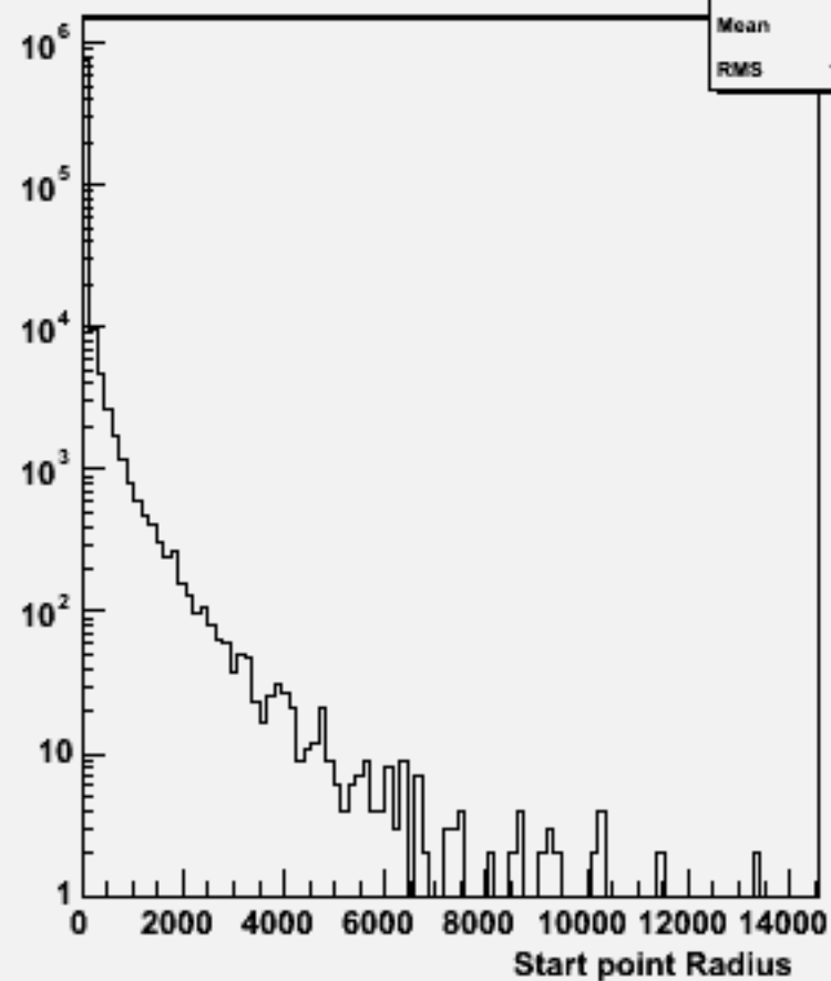
Start point R : w101608 uun1e1du_o
