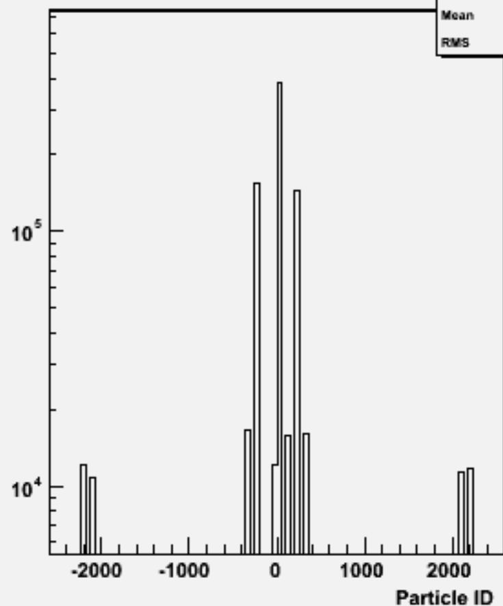
Particle ID : w101608 uun1e1du_o
