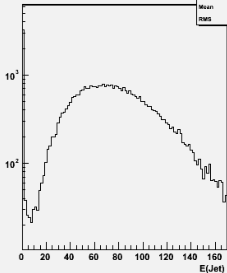
Jet energies(All jets)w101608 uun1e1du_o
