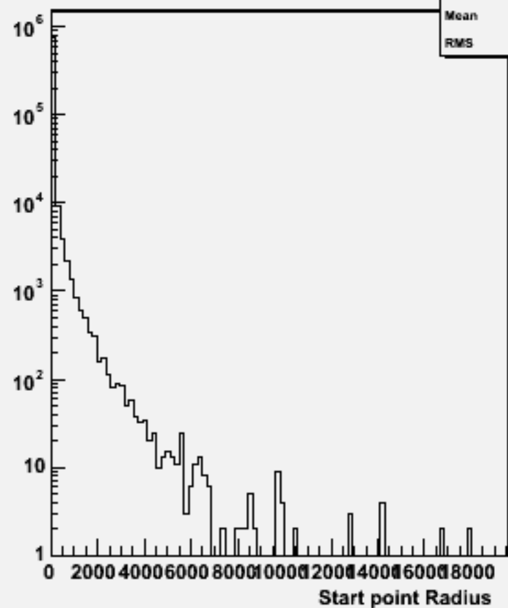
Start point R : w101607 uun1e1du_o
