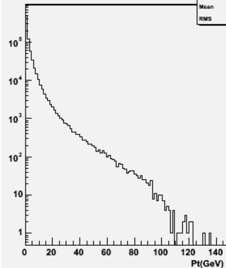
Particle Pt : w101607 uun1e1du_o
