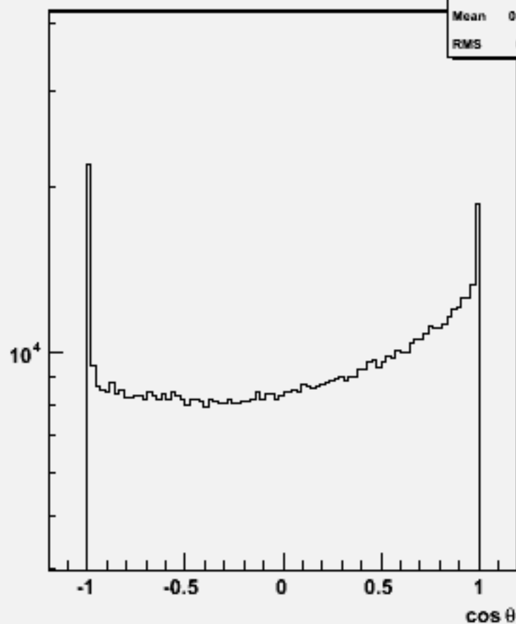
Particle cos \theta : w101607 uun1e1du_o
