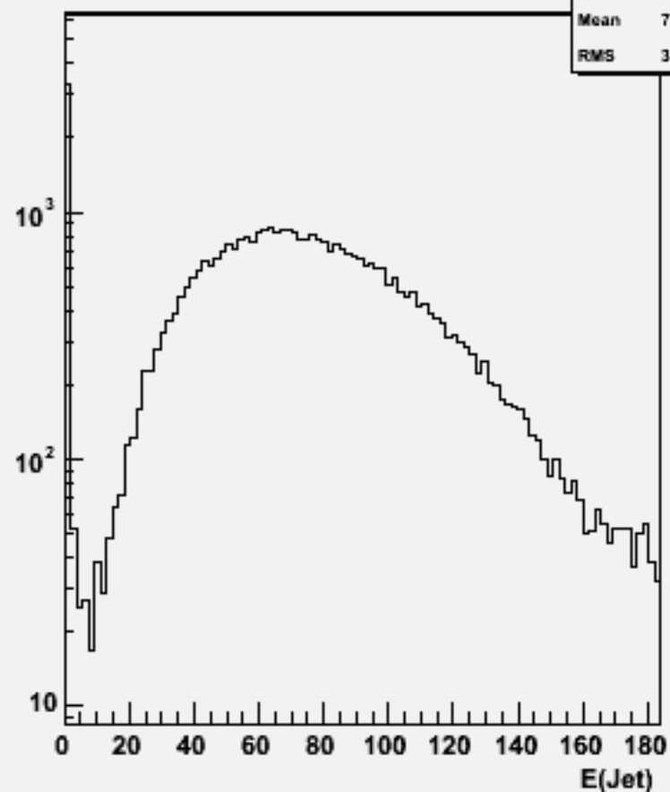
Jet energies(All jets)w101607 uun1e1du_o
