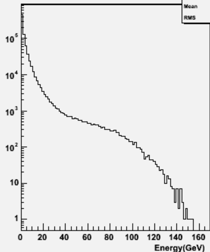
Particle Energy : w101607 uun1e1du_o
