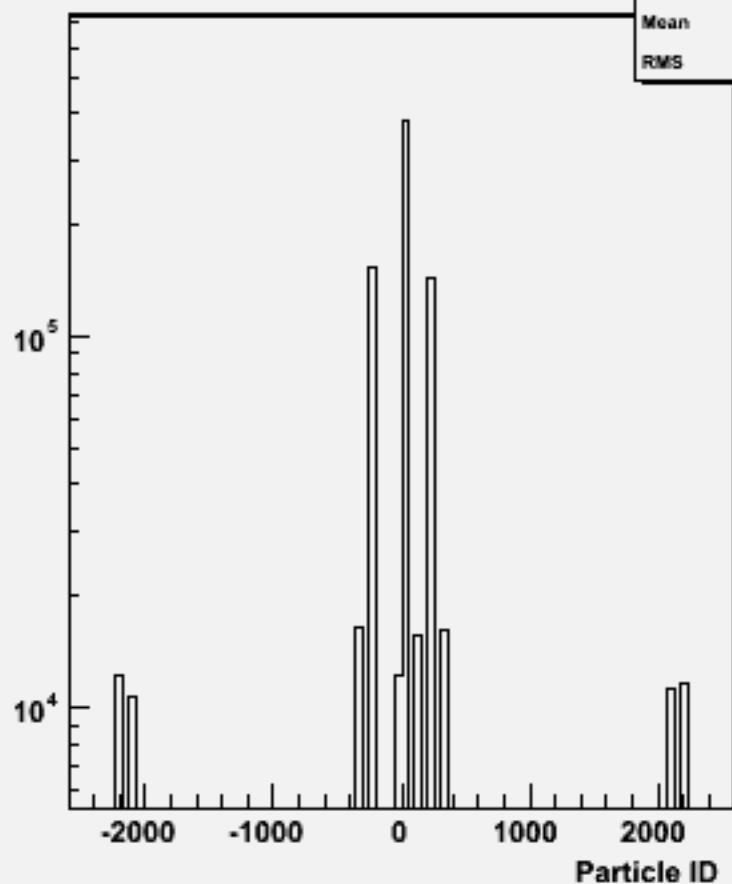
Particle ID : w101607 uun1e1du_o
