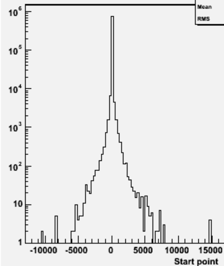
Start point Z : w101607 uun1e1du_o
