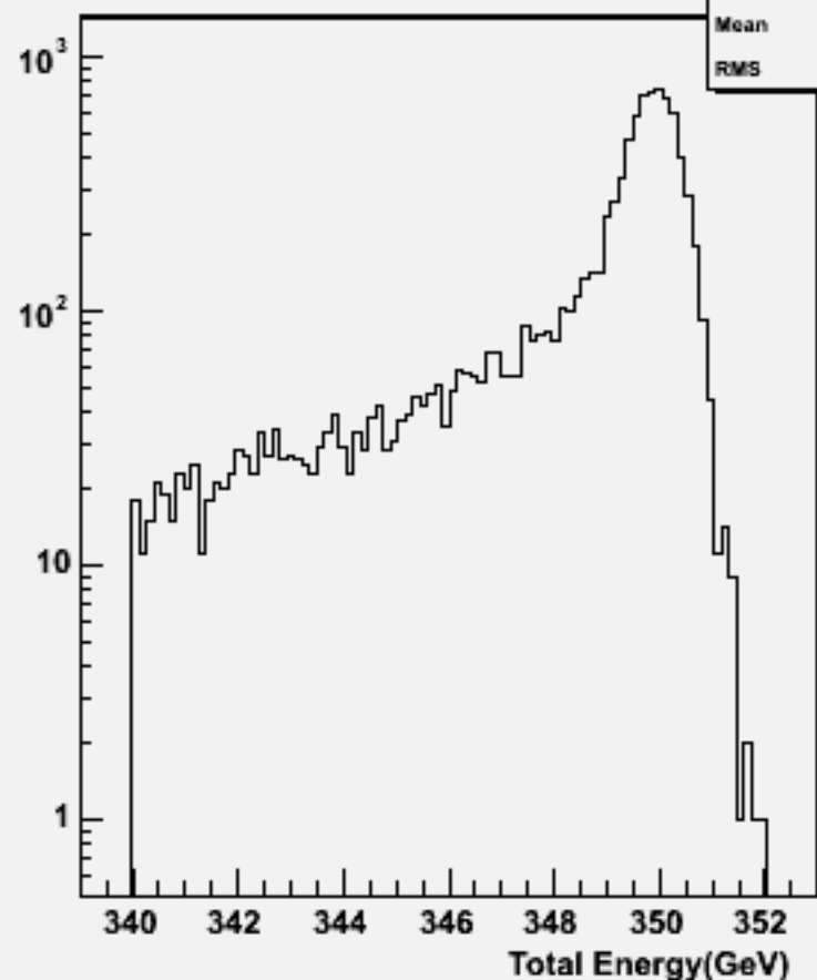
Pz Sum: w101605 uun1e1e3n3_o
