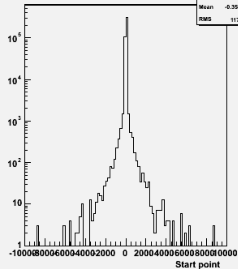
Start point Z : w101605 uun1e1e3n3_o
