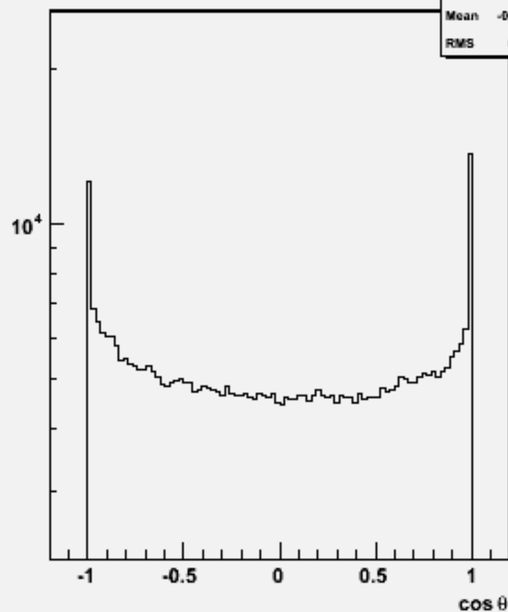
Particle cos \theta : w101605 uun1e1e3n3_o
