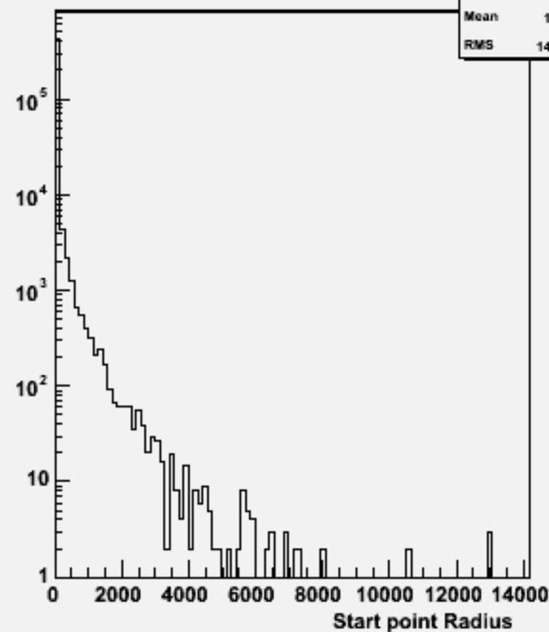
Start point R : w101605 uun1e1e3n3_o
