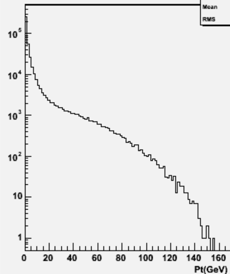
Start point Z : w101605 uun1e1e3n3_o
