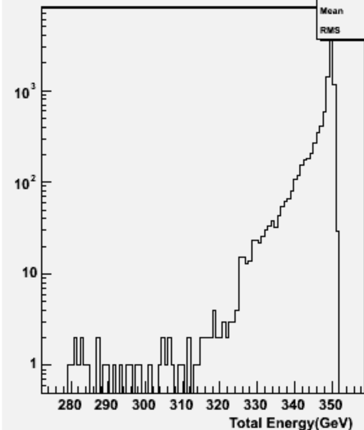
Pt Sum: w101605 uun1e1e3n3_o
