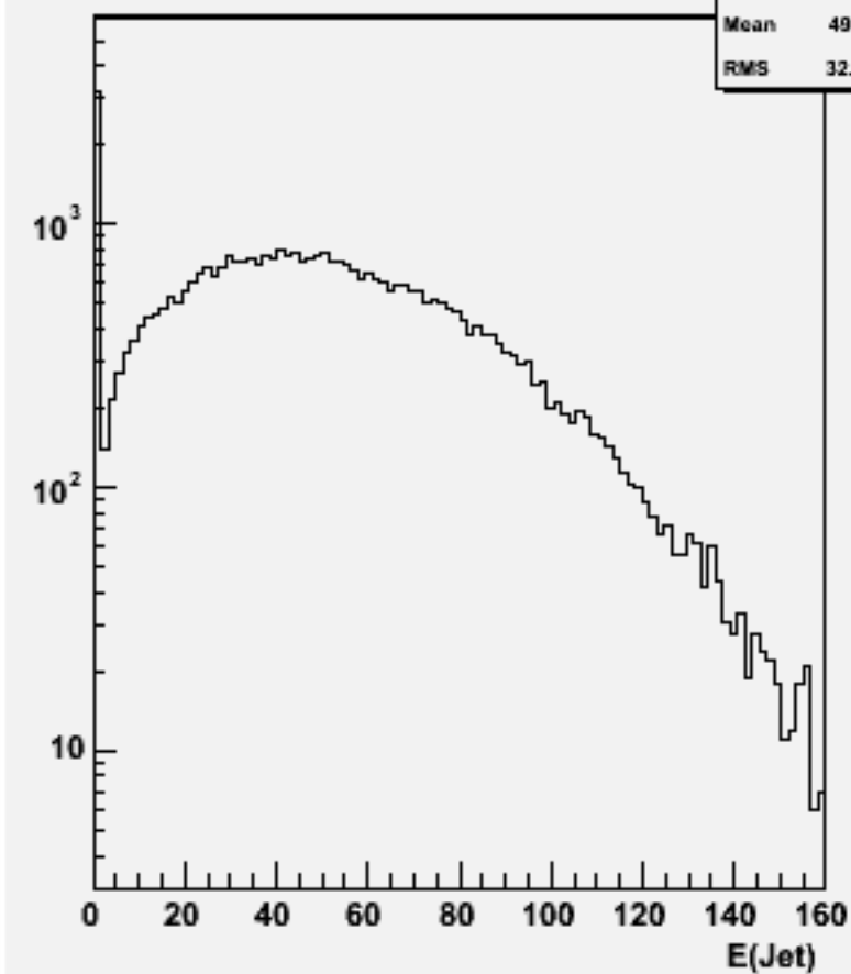
Jet energies(All jets)w101605 uun1e1e3n3_o
