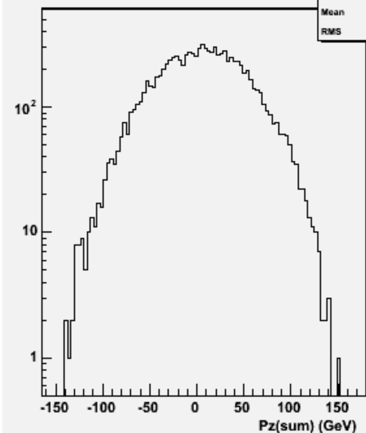
Pz Sum: w101605 uun1e1e3n3_o
