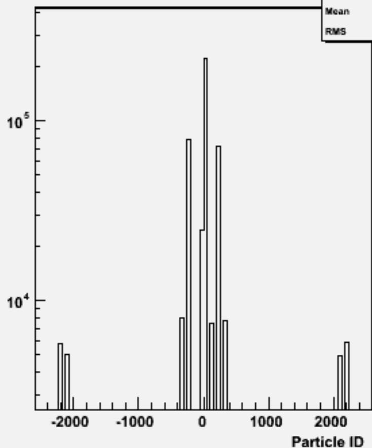
Particle ID : w101603 uun1e1e3n3_o
