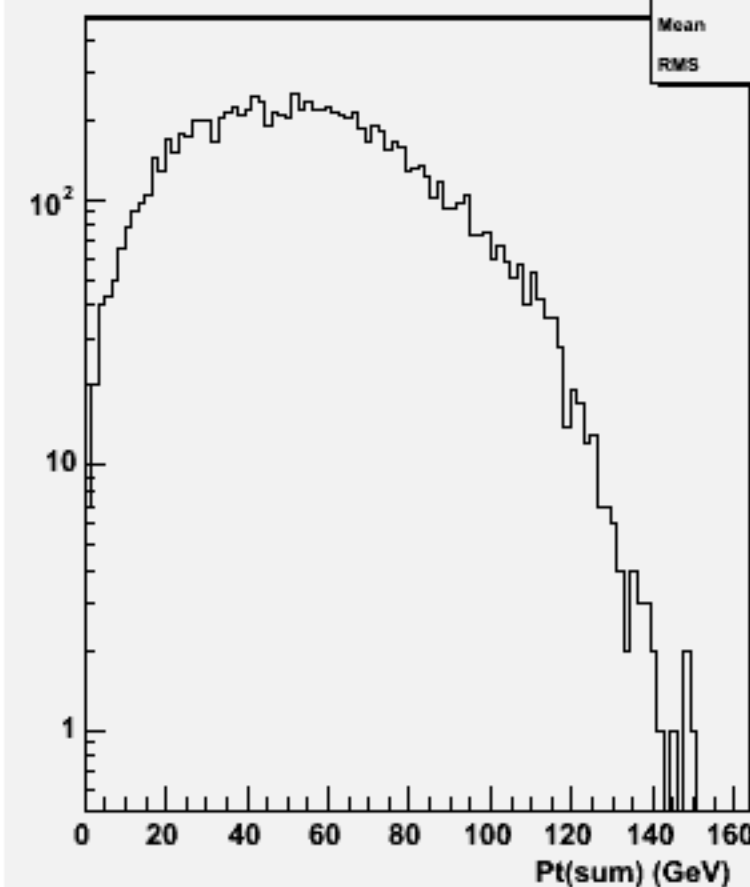
Pt Sum: w101603 uun1e1e3n3_o
