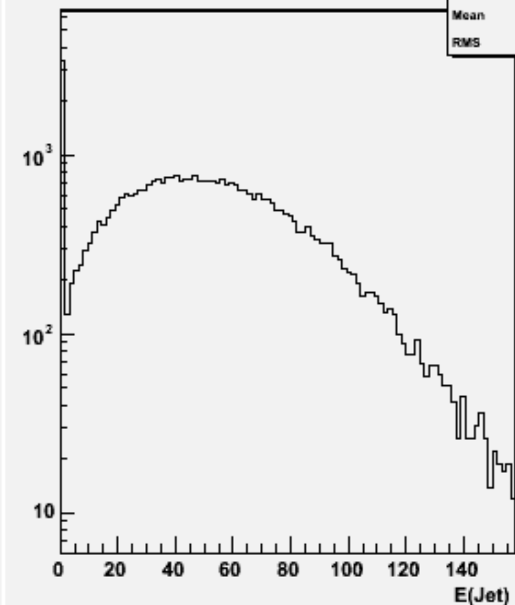
Jet energies(All jets)w101603 uun1e1e3n3_o
