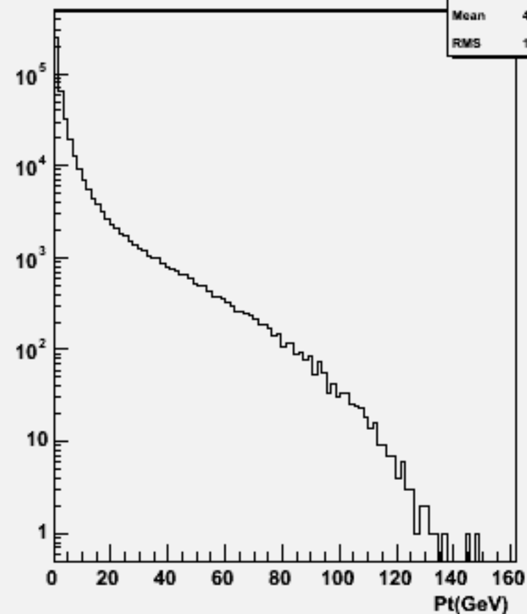
Particle Pt : w101603 uun1e1e3n3_o
