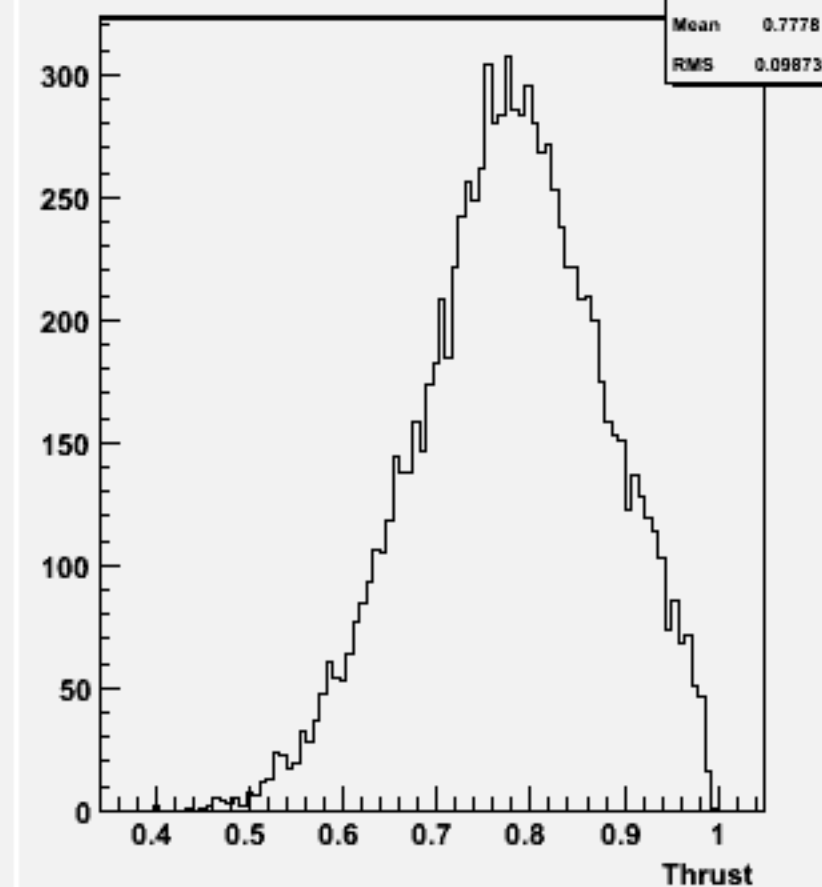
Thrust w101603 uun1e1e3n3_o
