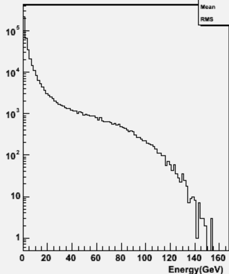
Particle Energy : w101603 uun1e1e3n3_o
