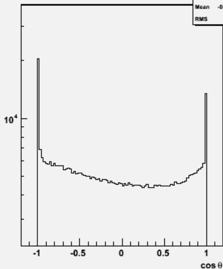
Particle cos \theta : w101603 uun1e1e3n3_o
