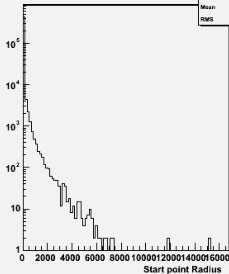
Start point R : w101603 uun1e1e3n3_o
