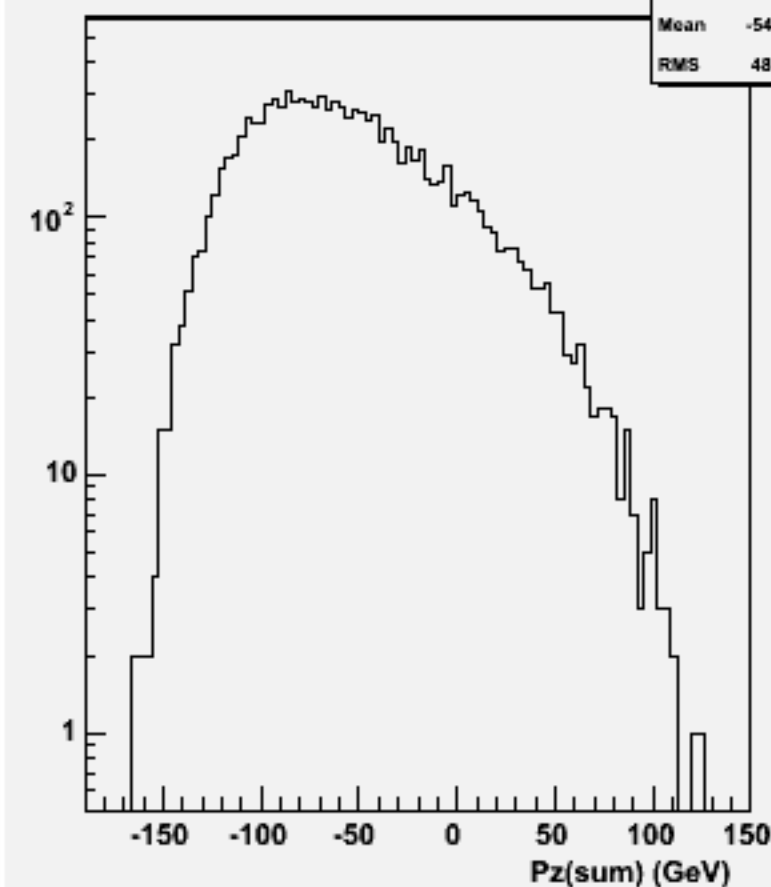
Pz Sum: w101603 uun1e1e3n3_o
