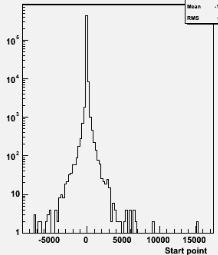
Start point Z : w101603 uun1e1e3n3_o
