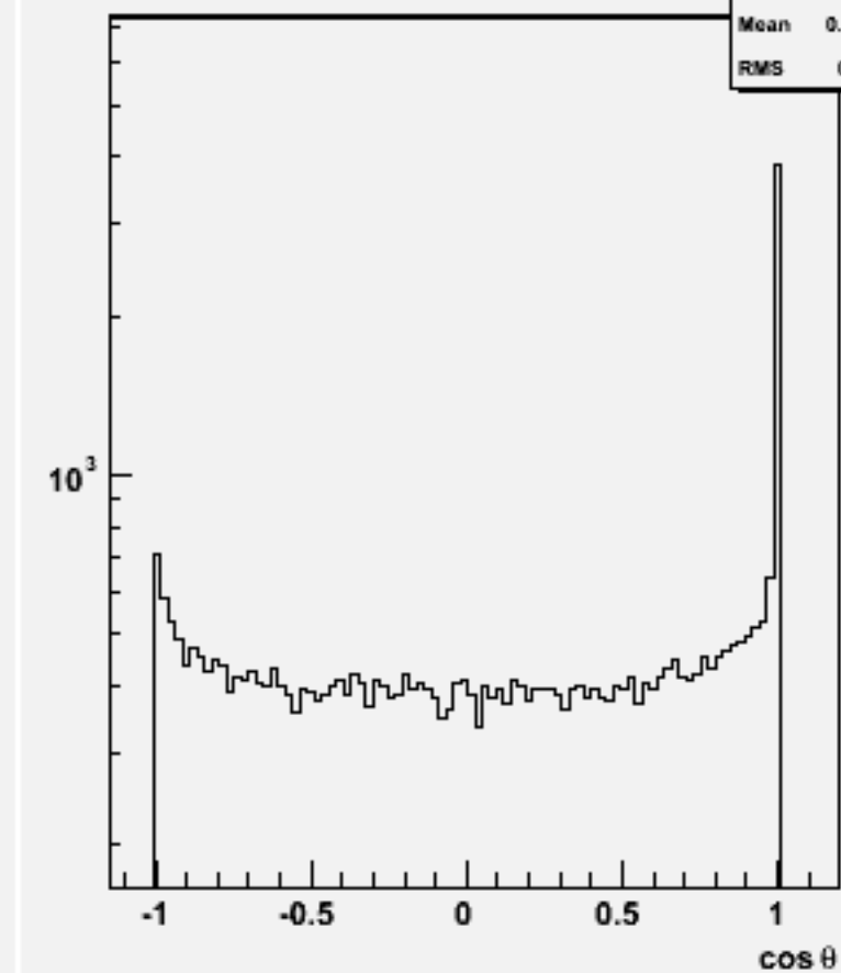
Jet cos \theta (All jets)w101601 uun1e1e2n2_o
