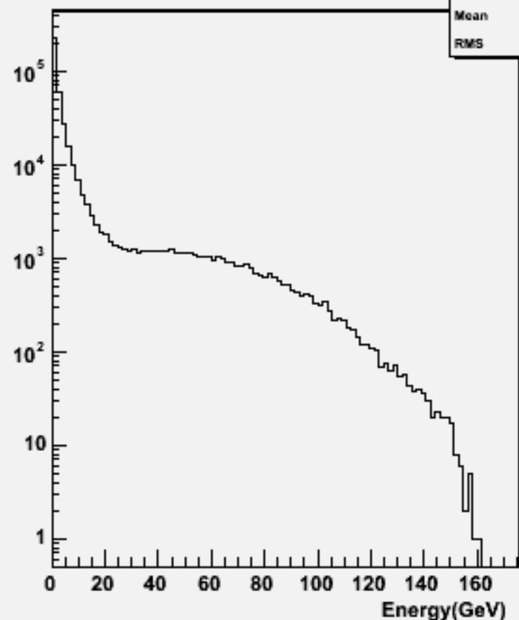
Start point R : w101601 uun1e1e2n2_o
