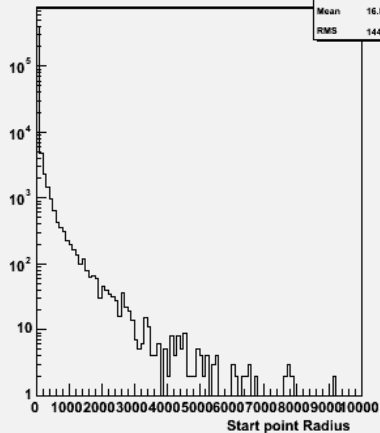
Start point R : w101601 uun1e1e2n2_o
