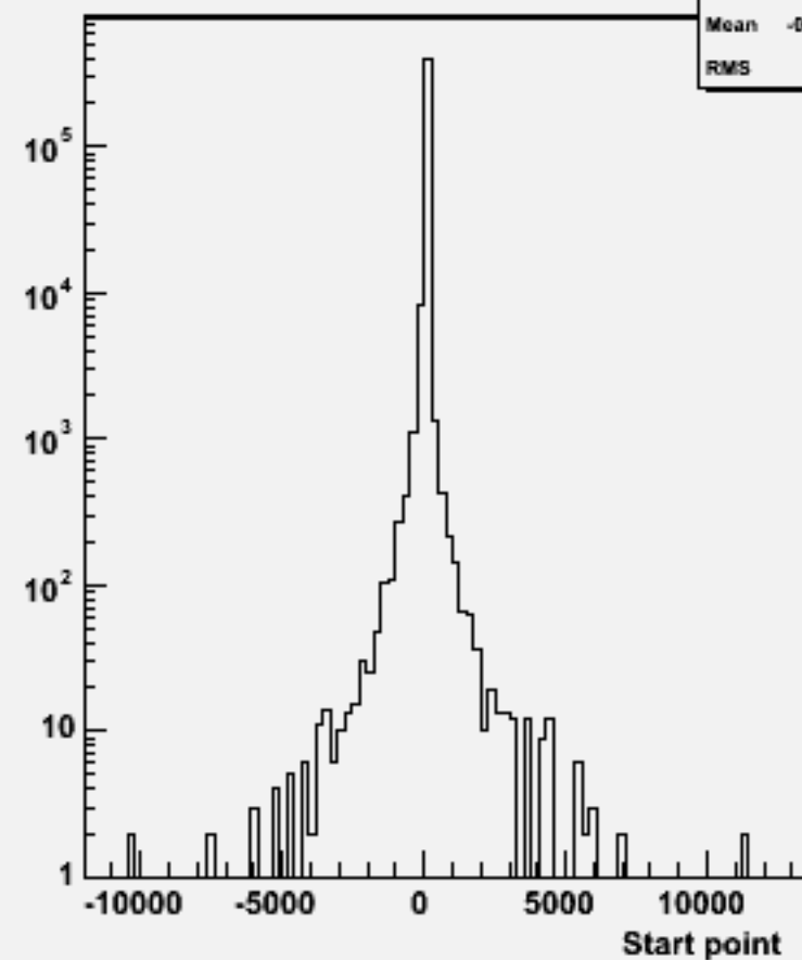
Start point Z : w101601 uun1e1e2n2_o
