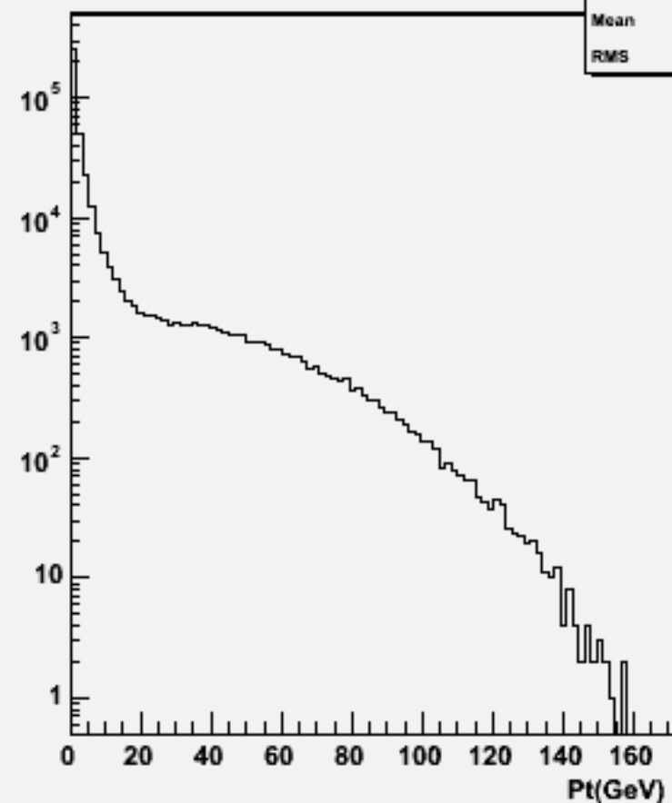
Start point Z : w101601 uun1e1e2n2_o
