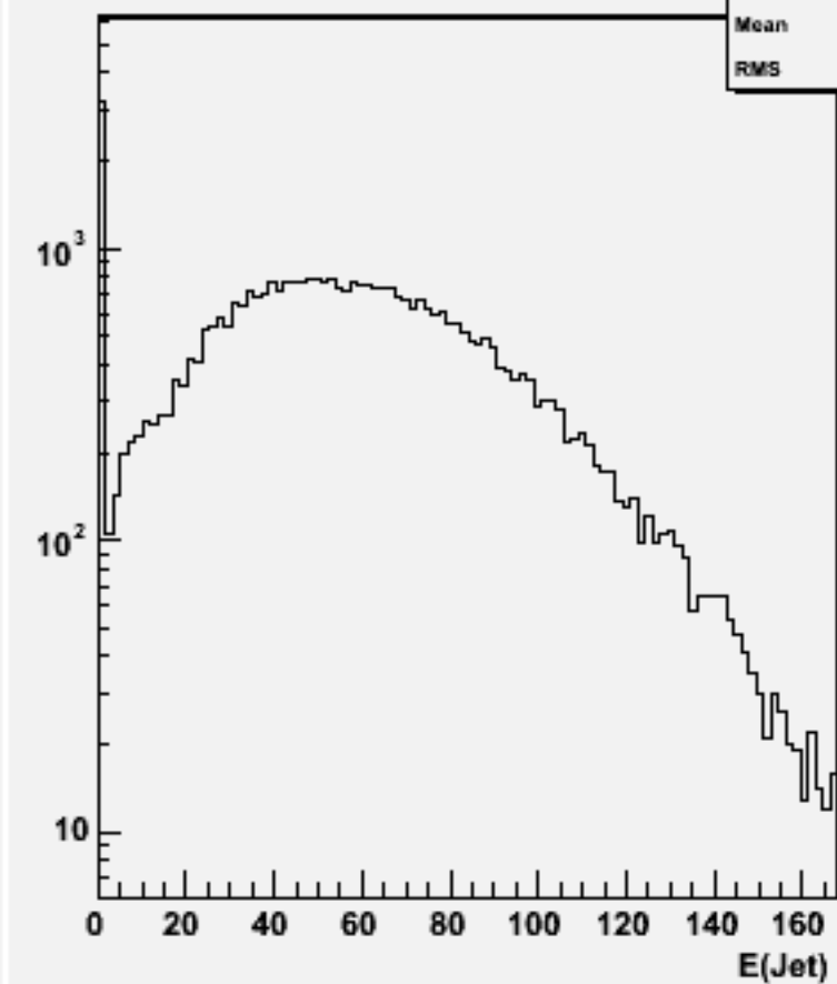
Jet energies(All jets)w101601 uun1e1e2n2_o
