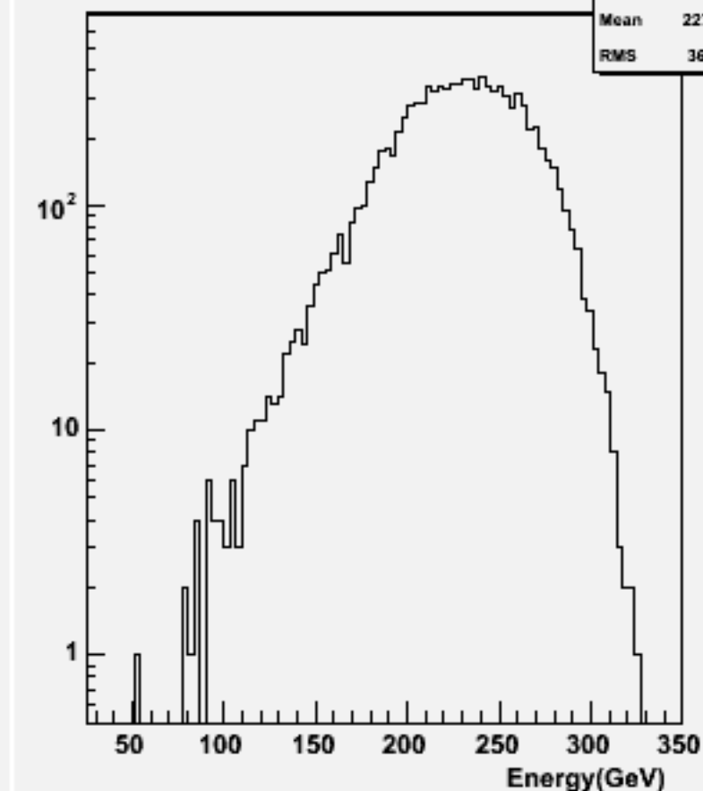
Thrust w101601 uun1e1e2n2_o
