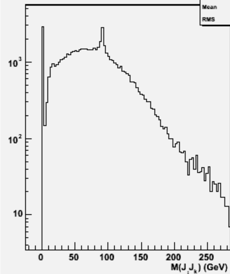
2jets mass(All comb)w101601 uun1e1e2n2_o
