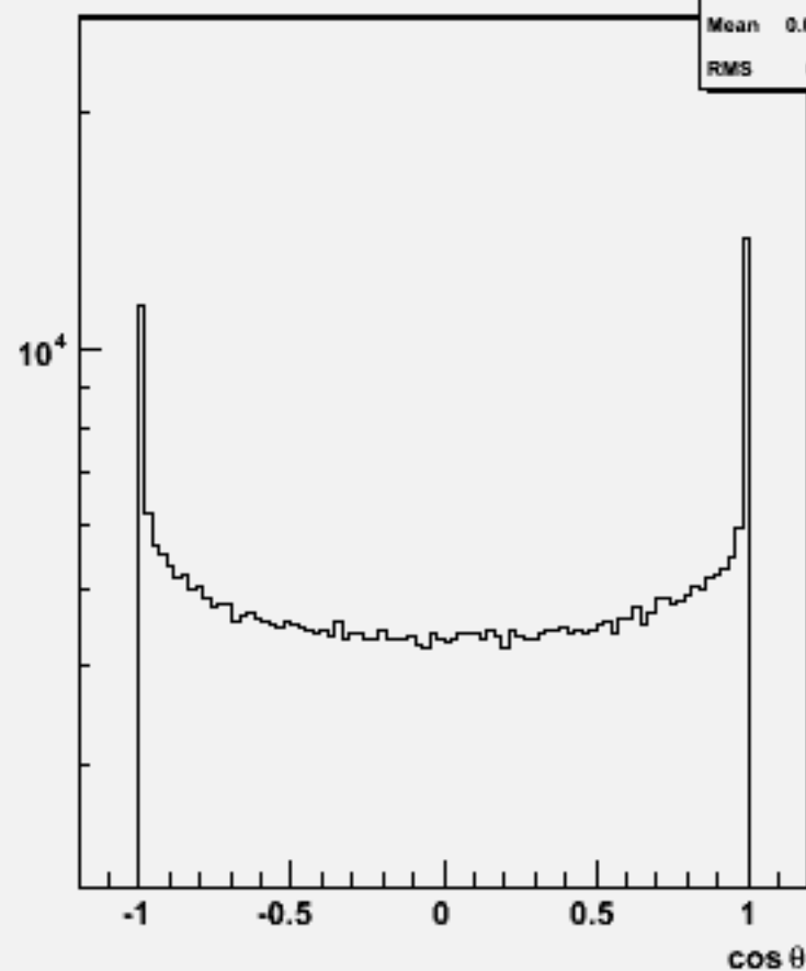
Particle cosθ : w101601 uun1e1e2n2_o
