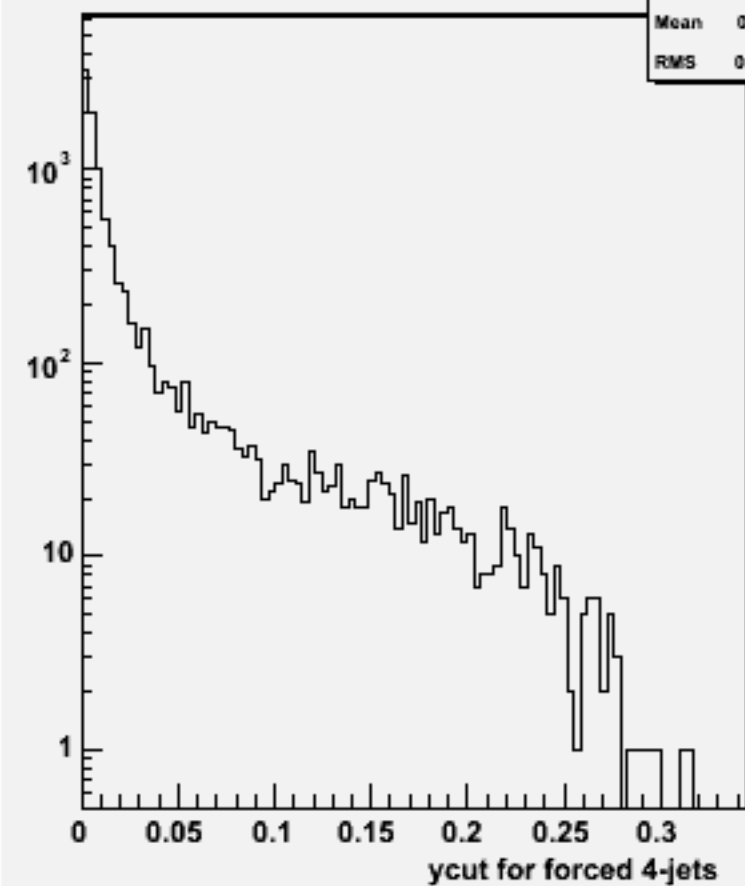
Ycut for 4-jets :w101601 uun1e1e2n2_o
