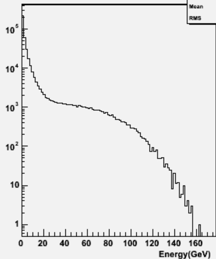
Start point R : w101600 uun1e1e2n2_o
