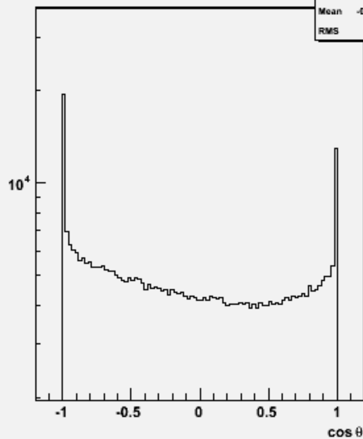
Particle cosθ : w101600 uun1e1e2n2_o
