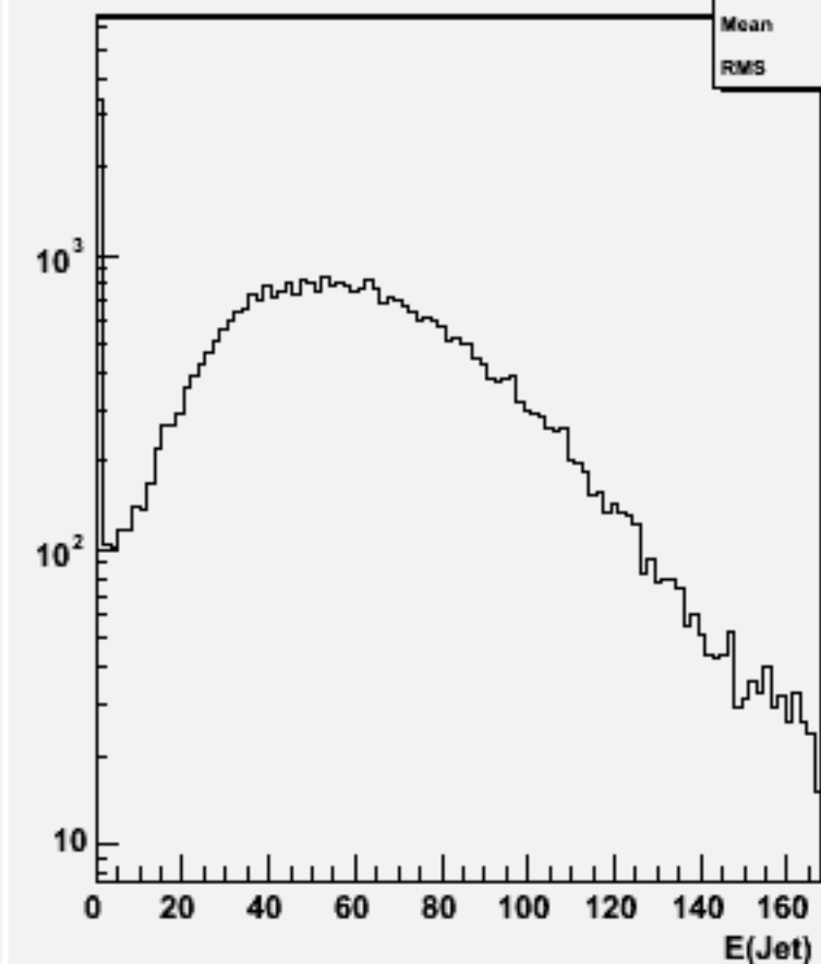
Jet energies(All jets)w101600 uun1e1e2n2_o
