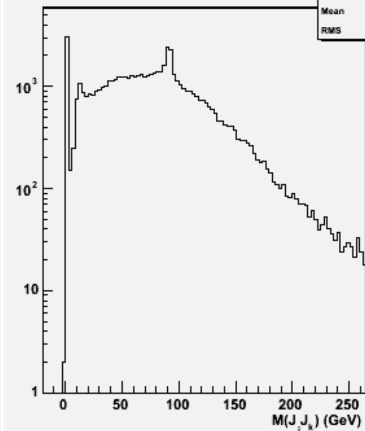
2jets mass(All comb)w101600 uun1e1e2n2_o
