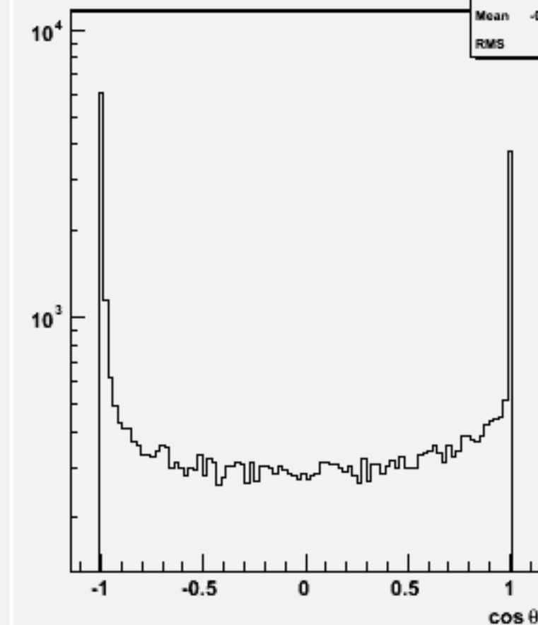
Jet cos \theta (All jets)w101600 uun1e1e2n2_o
