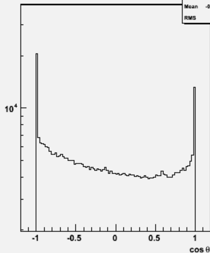
Particle cos \theta : w101599 uun1e1e2n2_o
