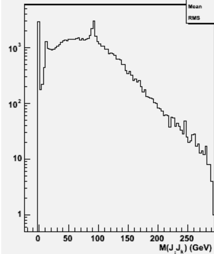
2jets mass(All comb)w101599 uun1e1e2n2_o
