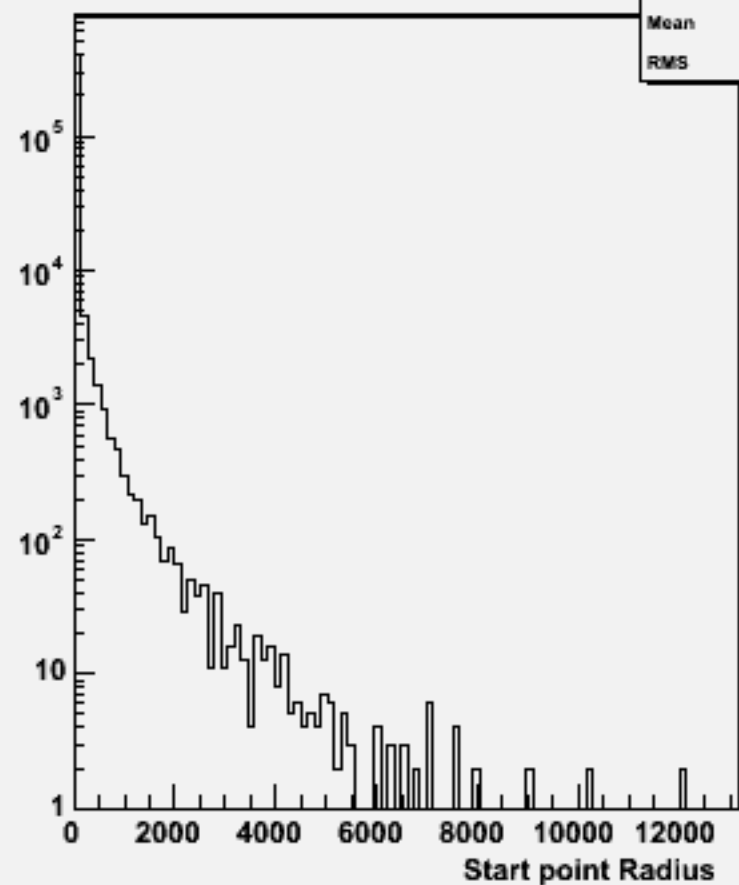
Start point R : w101599 uun1e1e2n2_o
