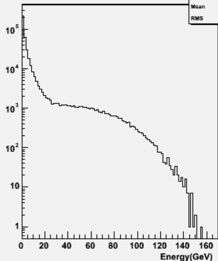
Start point R : w101599 uun1e1e2n2_o
