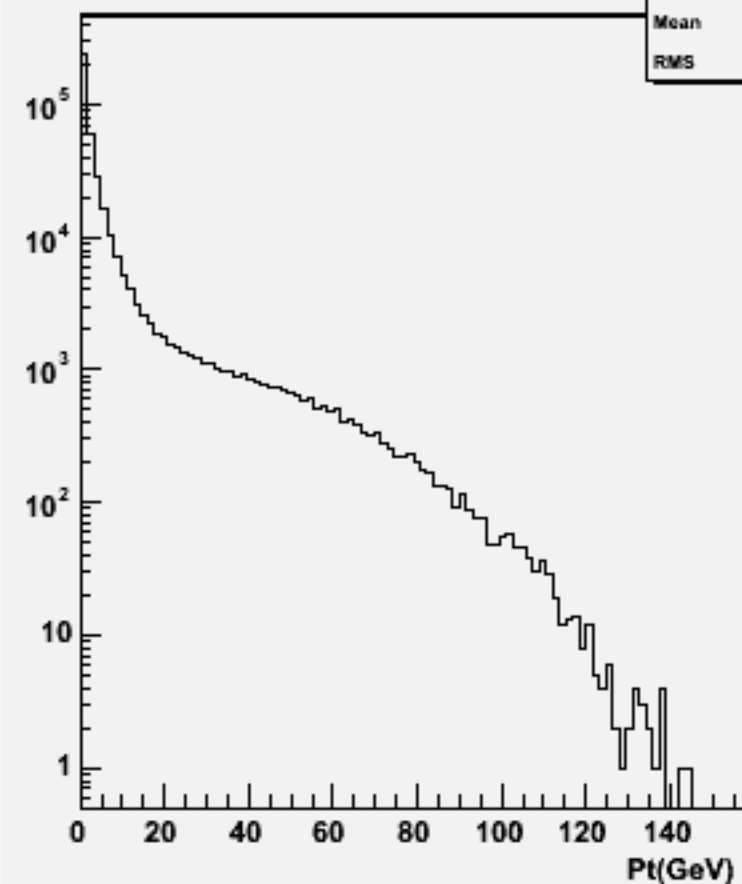
Start point Z : w101599 uun1e1e2n2_o
