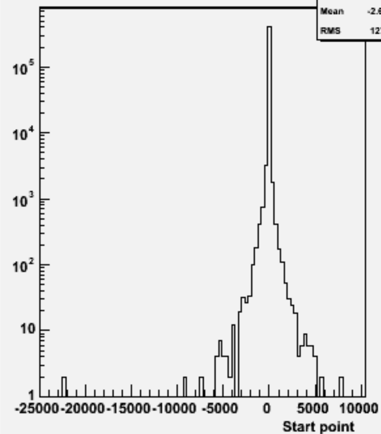
Start point Z : w101599 uun1e1e2n2_o
