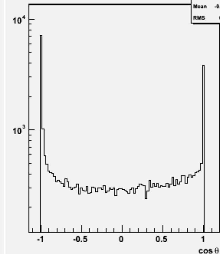
Jet cos \theta (All jets)w101599 uun1e1e2n2_o
