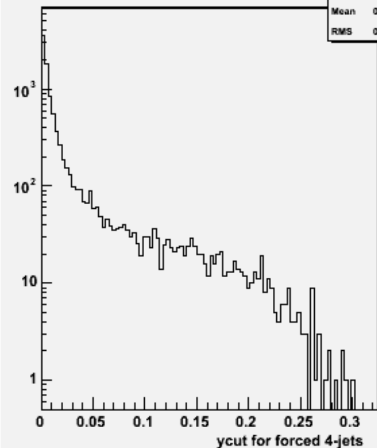
Ycut for 4-jets :w101599 uun1e1e2n2_o
