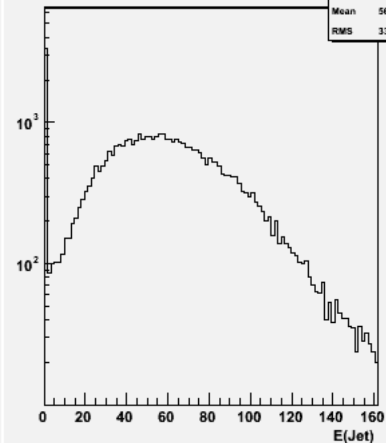
Jet energies(All jets)w101599 uun1e1e2n2_o
