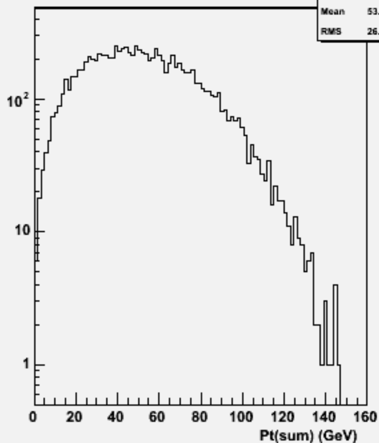
Pt Sum: w101598 uun1e1e1n1_o
