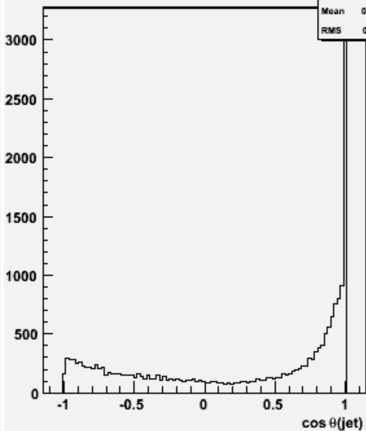
cos \theta for 2-jets :w101598 uun1e1e1n1_o
