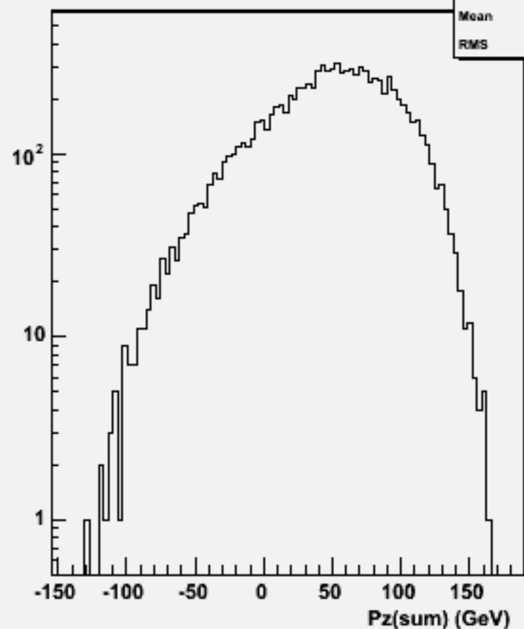
Pz Sum: w101598 uun1e1e1n1_o
