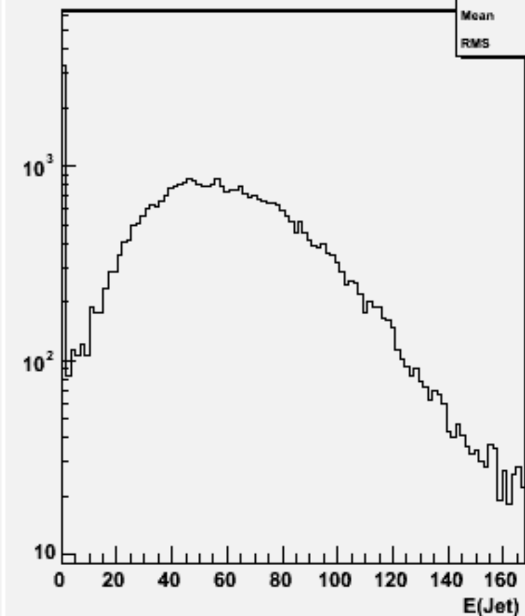
Jet energies(All jets)w101598 uun1e1e1n1_o
