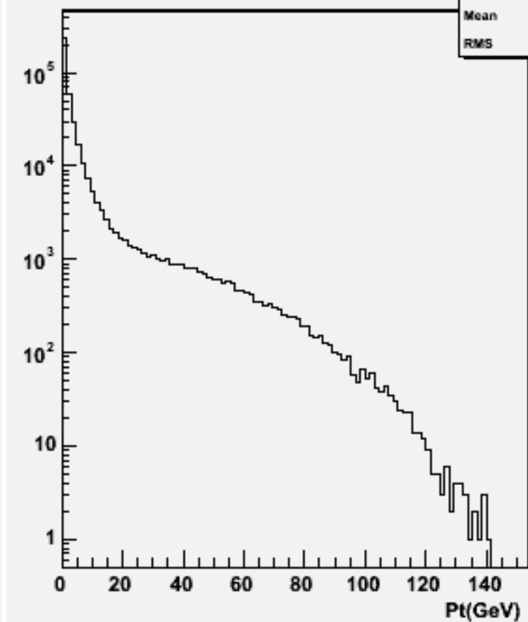
Particle Pt : w101598 uun1e1e1n1_o
