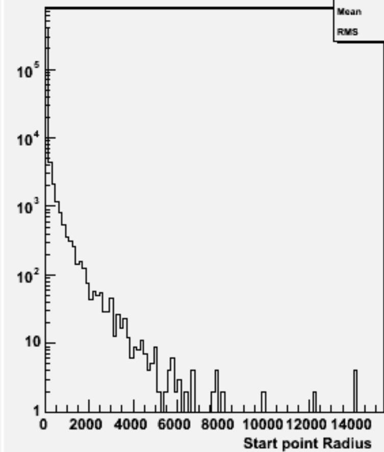
Start point R : w101598 uun1e1e1n1_o
