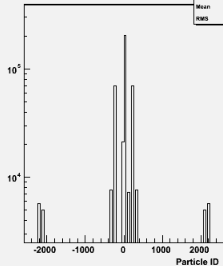
Particle ID : w101598 uun1e1e1n1_o
