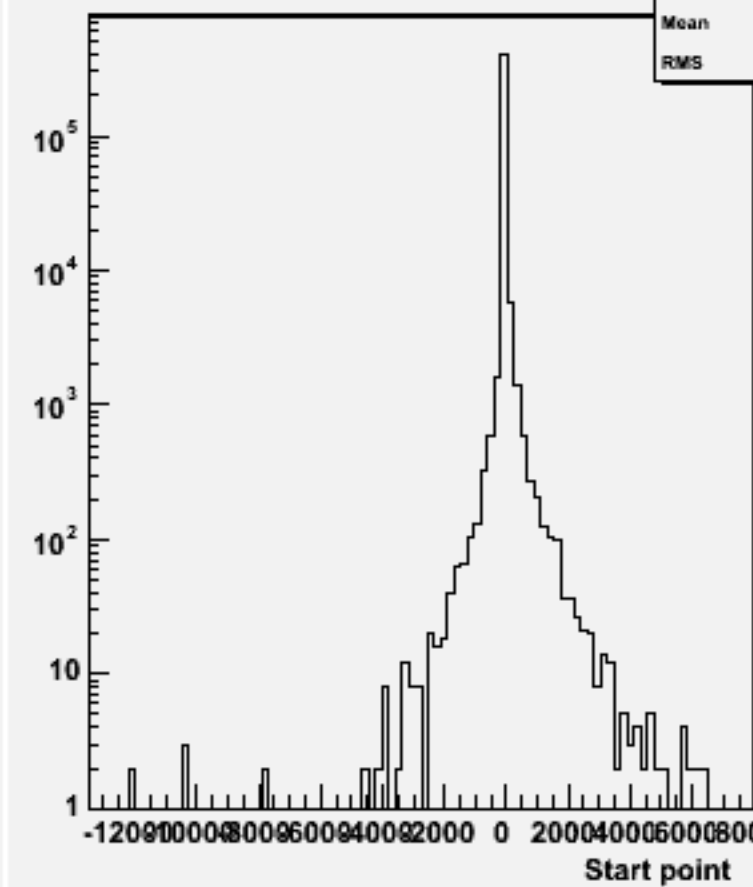
Start point Z : w101598 uun1e1e1n1_o
