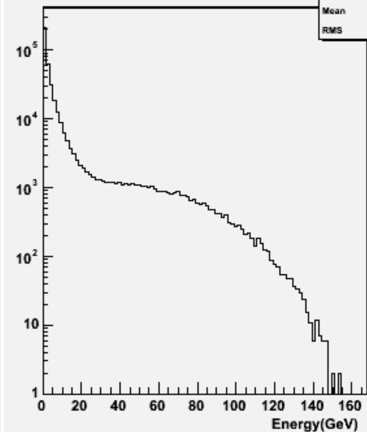
Particle Energy : w101598 uun1e1e1n1_o
