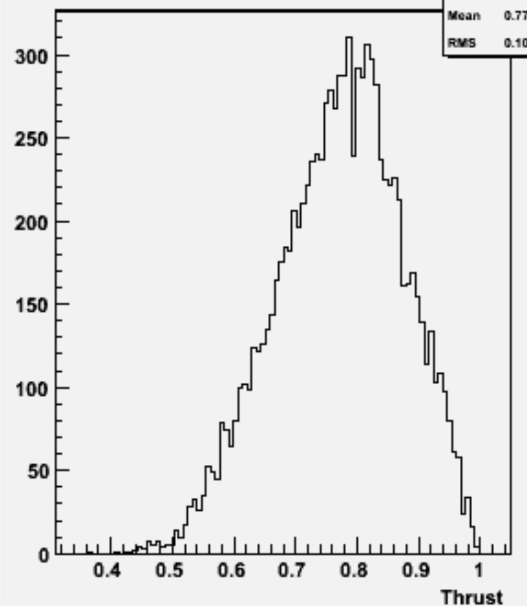
Thrust w101598 uun1e1e1n1_o
