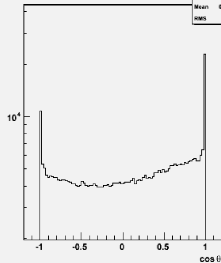
Particle cos \theta : w101598 uun1e1e1n1_o
