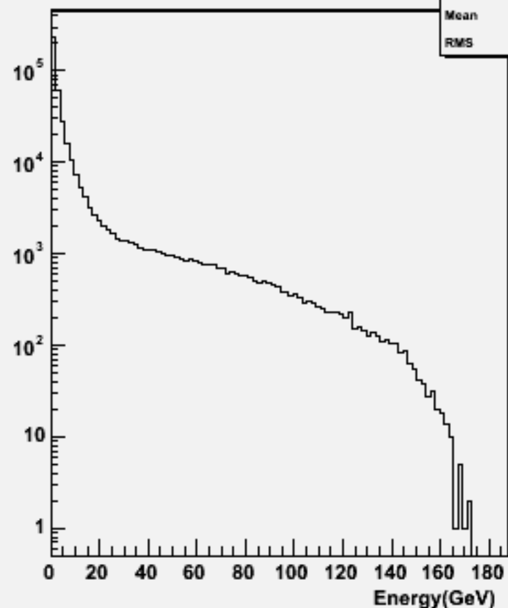
Start point R : w101597 uun1e1e1n1_o
