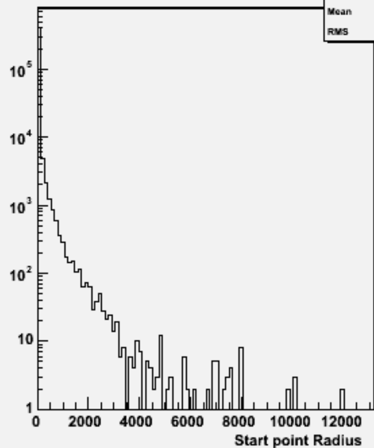
Start point R : w101597 uun1e1e1n1_o
