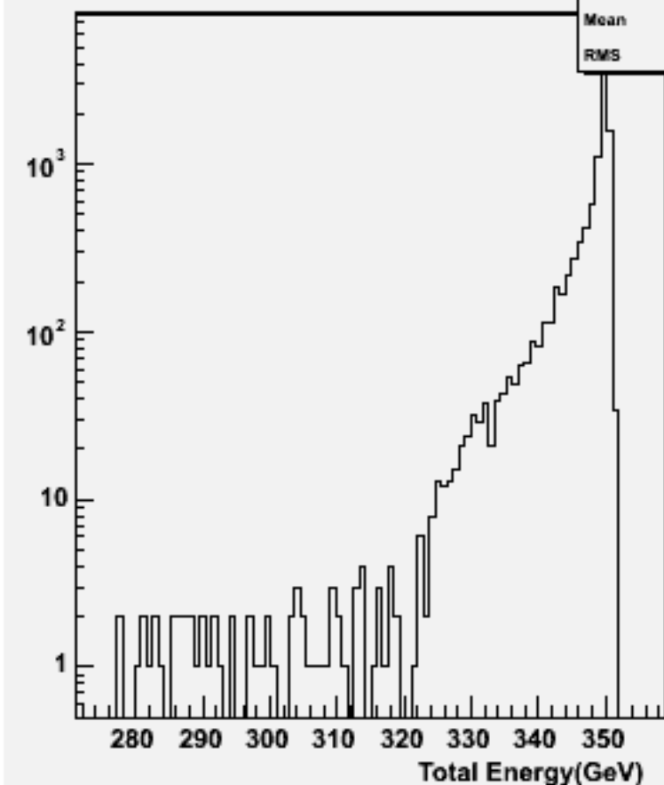
Pt Sum: w101597 uun1e1e1n1_o
