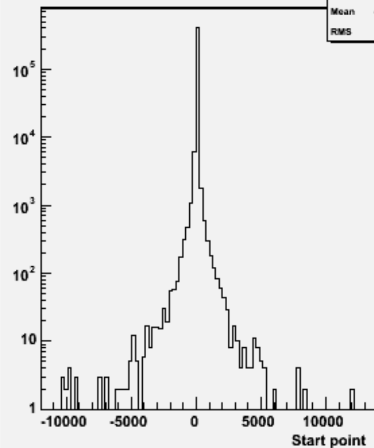
Start point Z : w101597 uun1e1e1n1_o
