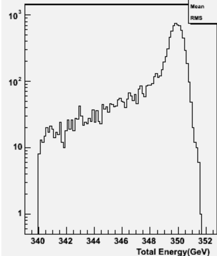
Pz Sum: w101597 uun1e1e1n1_o
