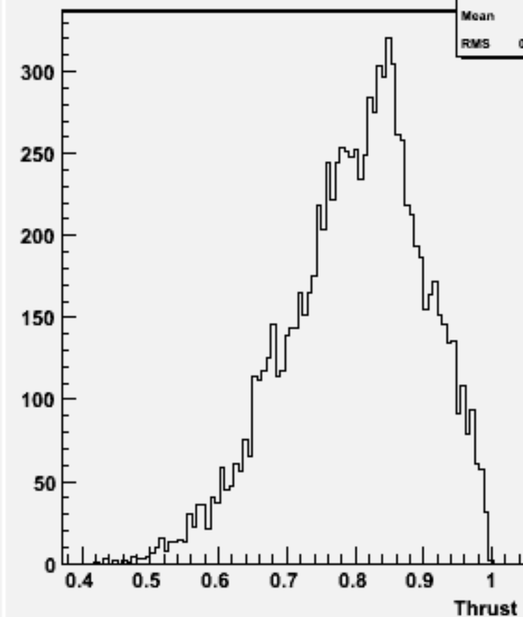
Thrust w101597 uun1e1e1n1_o
