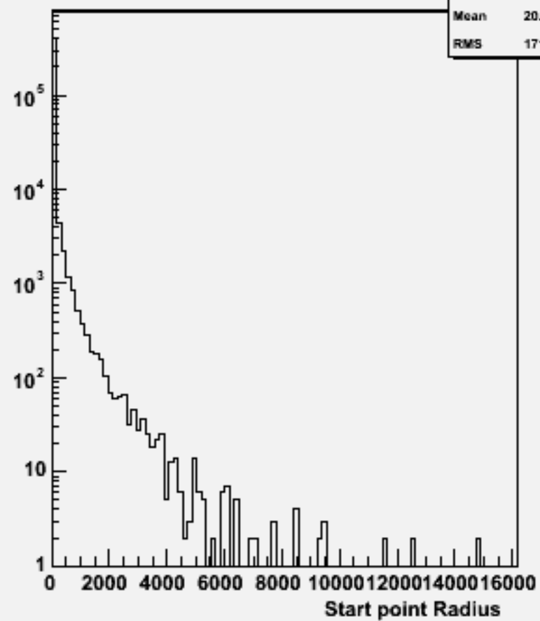
Start point R : w101595 uun1e1e1n1_o
