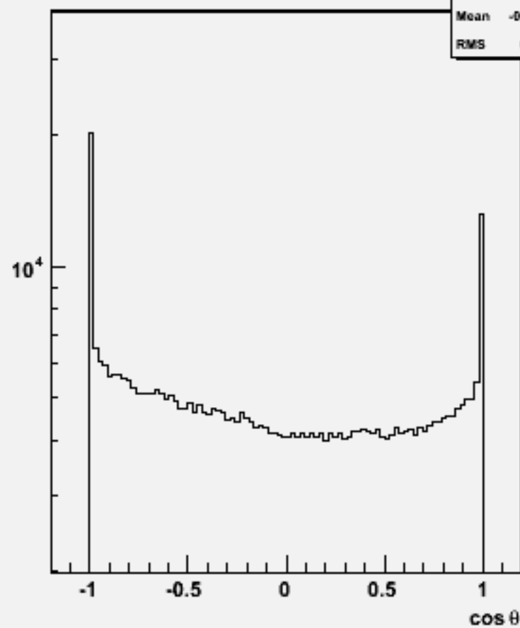
Particle cosθ : w101595 uun1e1e1n1_o
