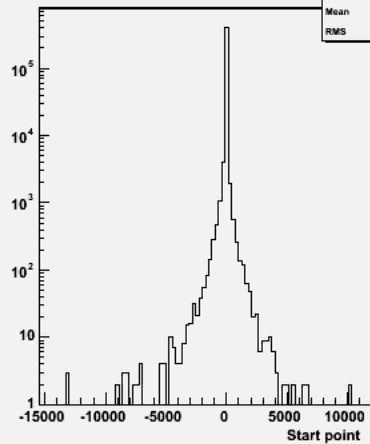
Start point Z : w101595 uun1e1e1n1_o
