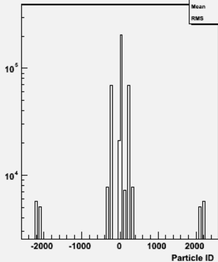
Particle ID : w101595 uun1e1e1n1_o
