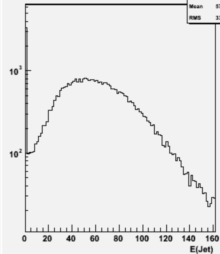
Jet energies(All jets)w101595 uun1e1e1n1_o
