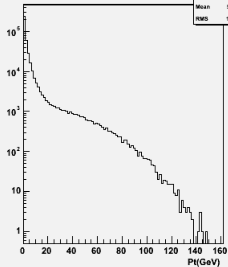
Particle Pt : w101595 uun1e1e1n1_o
