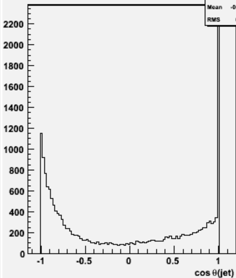
cos \theta for 2-jets :w101595 uun1e1e1n1_o
