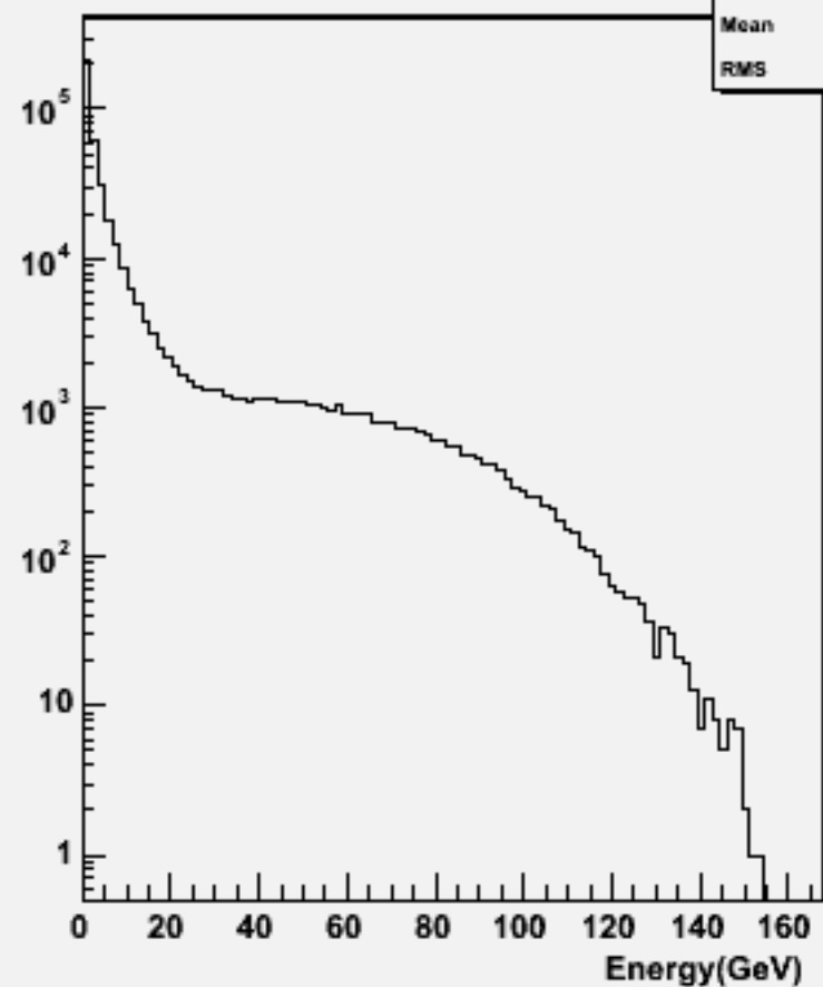
Particle Energy : w101595 uun1e1e1n1_o
