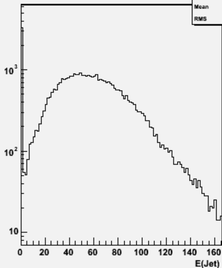
Jet energies(All jets)w101593 n3n3cssc_o
