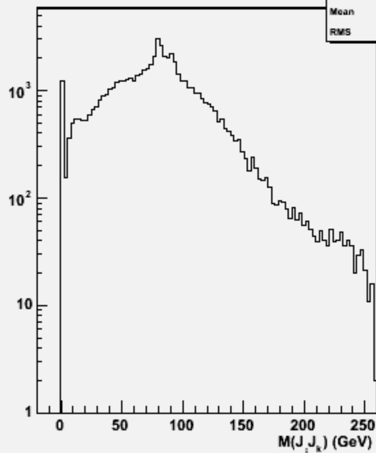
2jets mass(All comb)w101593 n3n3cssc_o
