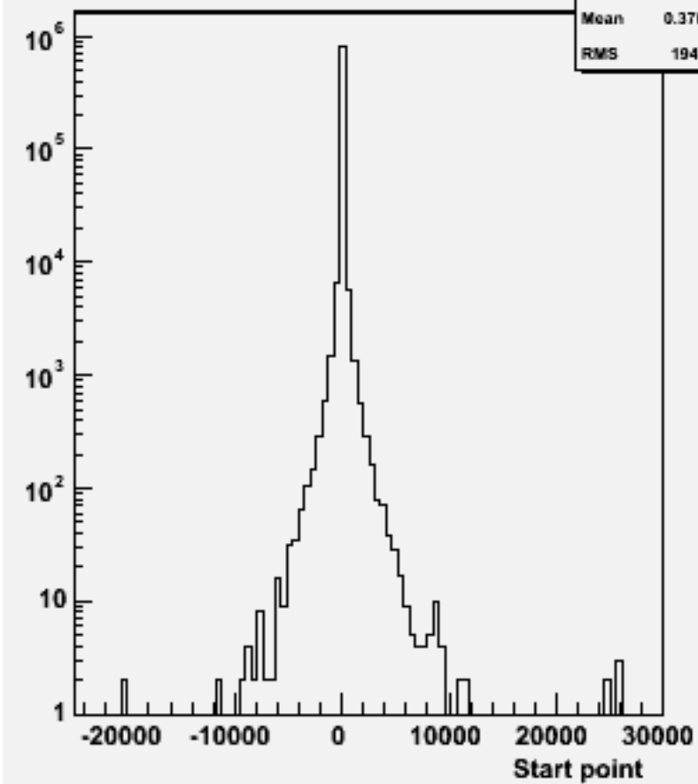
Start point Z : w101593 n3n3cssc_o
