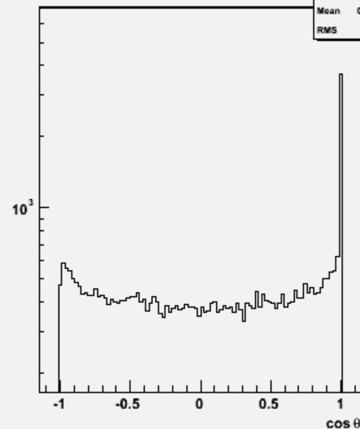
Jet cos \theta (All jets)w101593 n3n3cssc_o
