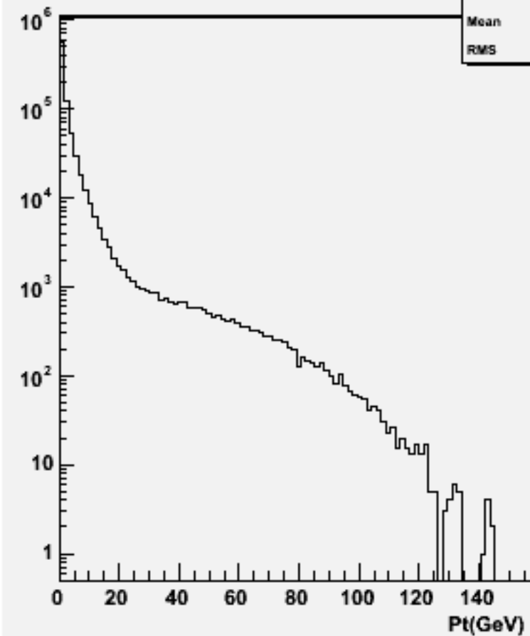
Particle Pt : w101593 n3n3cssc_o
