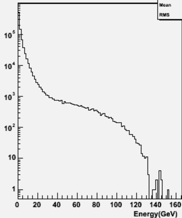
Particle Energy : w101592 n3n3cssc_o
