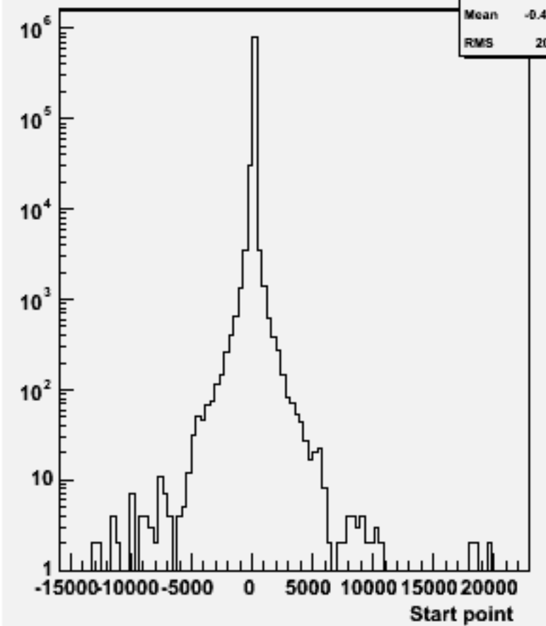
Start point Z : w101592 n3n3cssc_o
