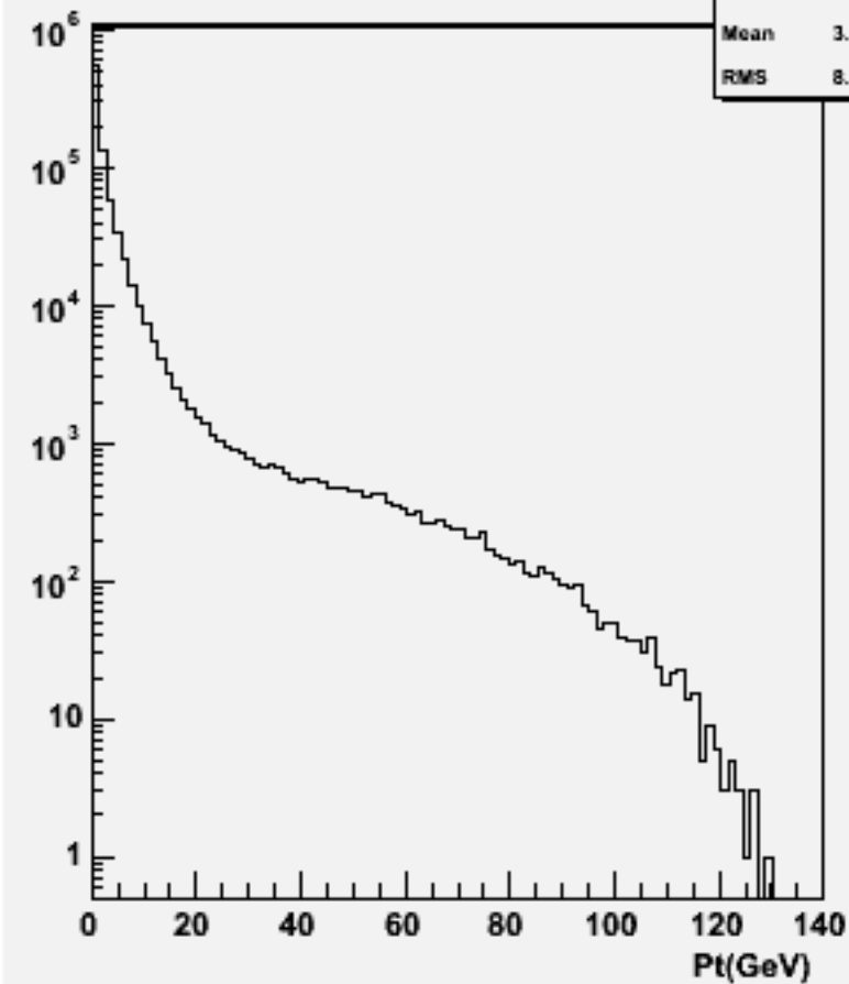
Particle Pt : w101592 n3n3cssc_o
