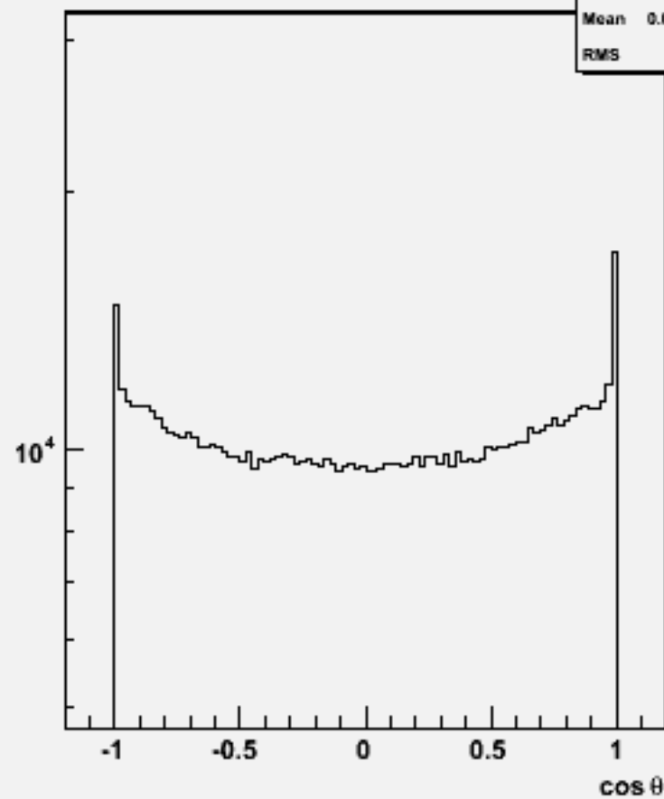
Particle cos \theta : w101592 n3n3cssc_o
