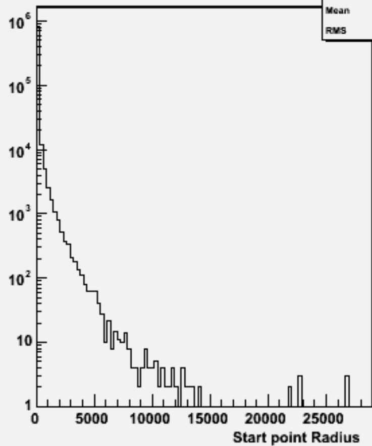
Start point R : w101592 n3n3cssc_o
