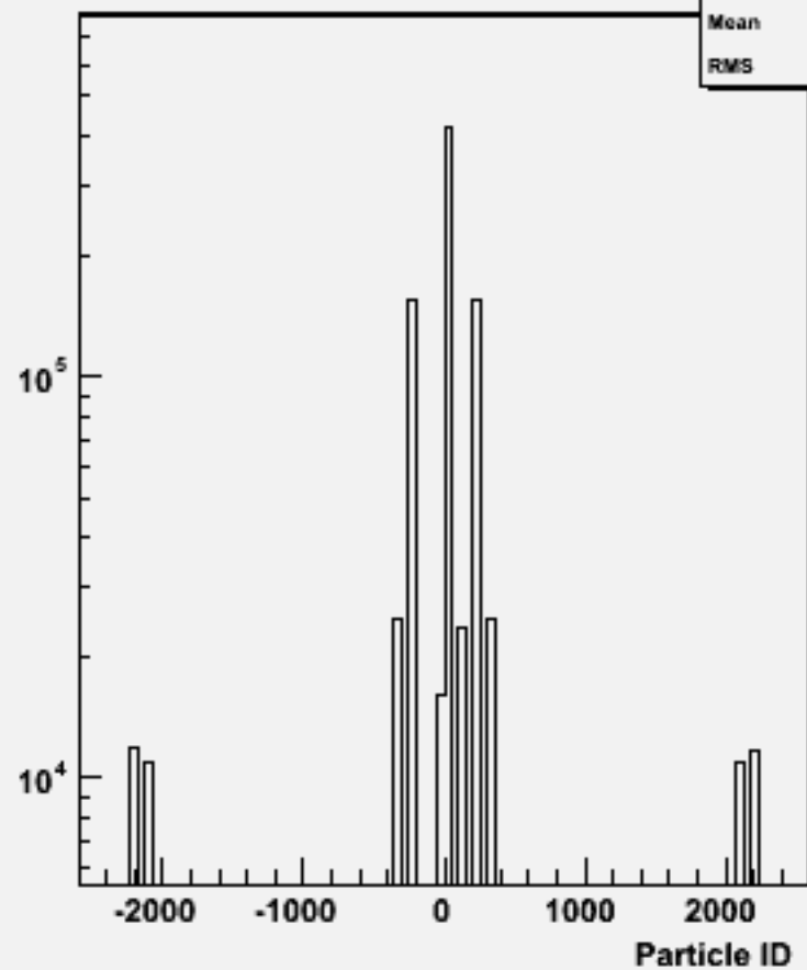
Particle ID : w101592 n3n3cssc_o
