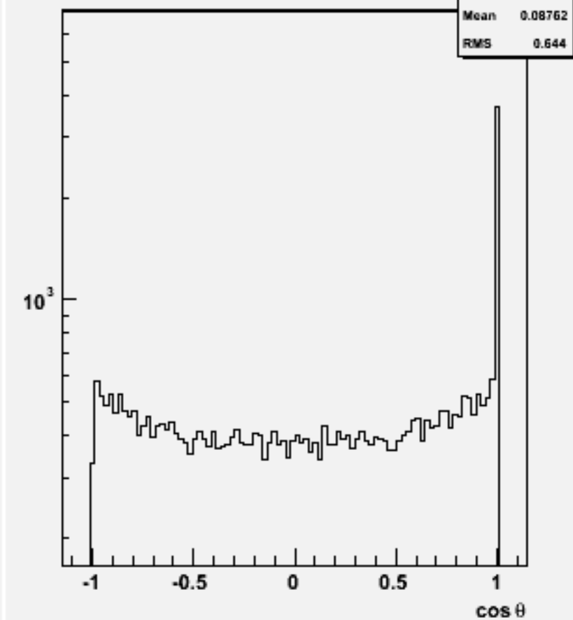
Jet cosθ (All jets)w101592 n3n3cssc_o
