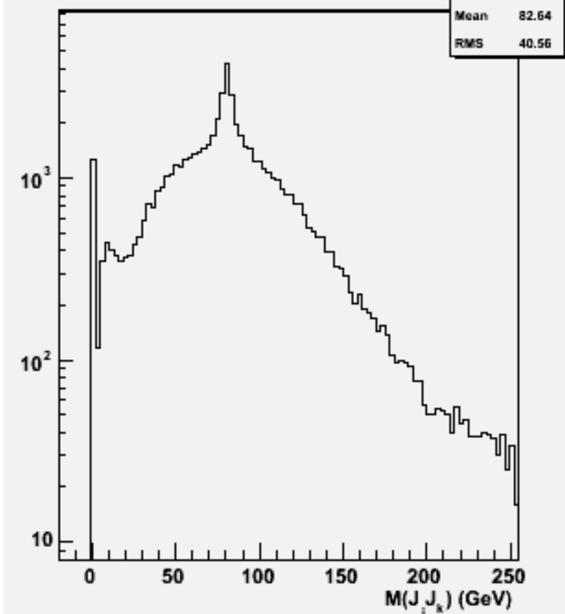
2jets mass(All comb)w101592 n3n3cssc_o
