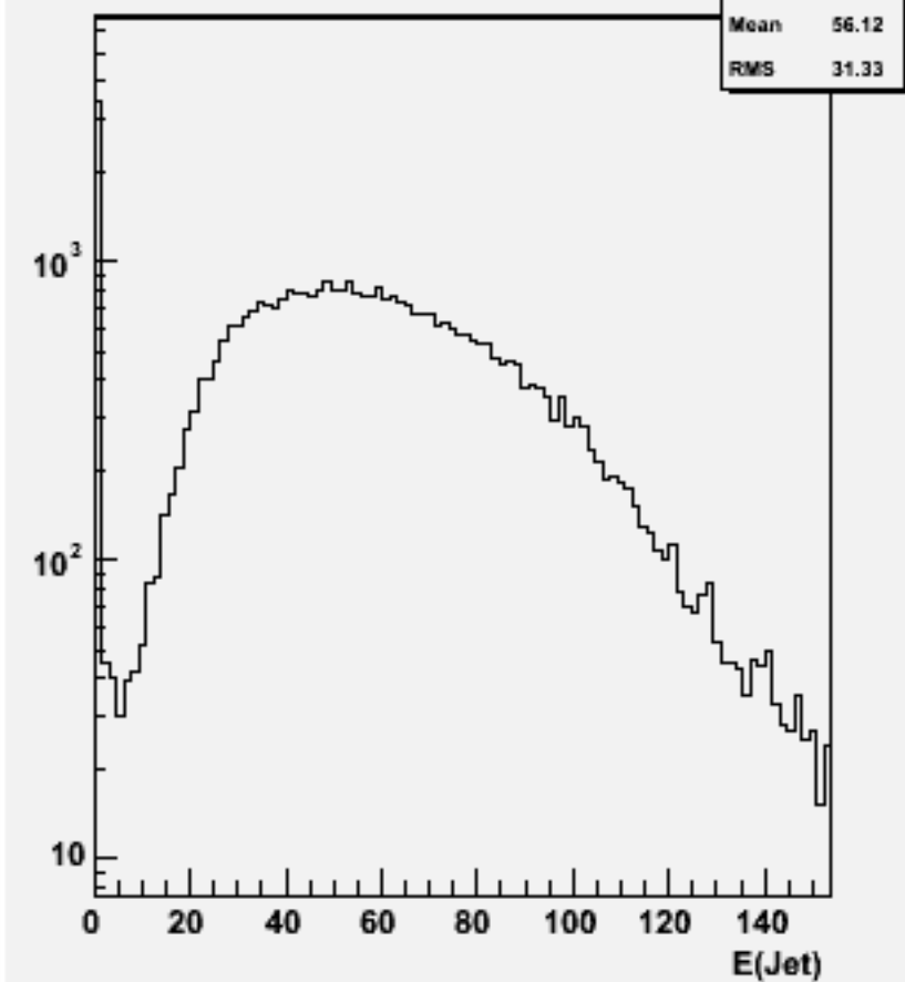
Jet energies(All jets)w101592 n3n3cssc_o
