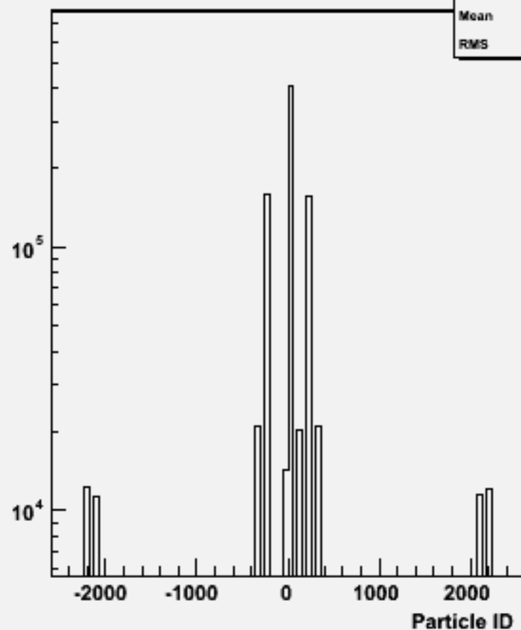
Particle ID : w101589 n3n3csdu_o
