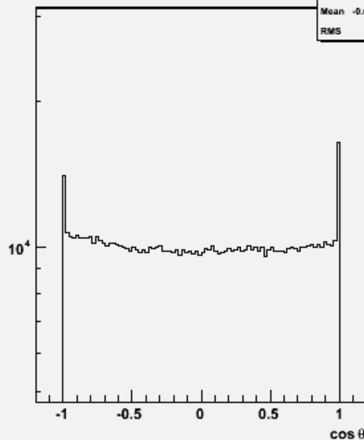
Particle cos \theta : w101589 n3n3csdu_o
