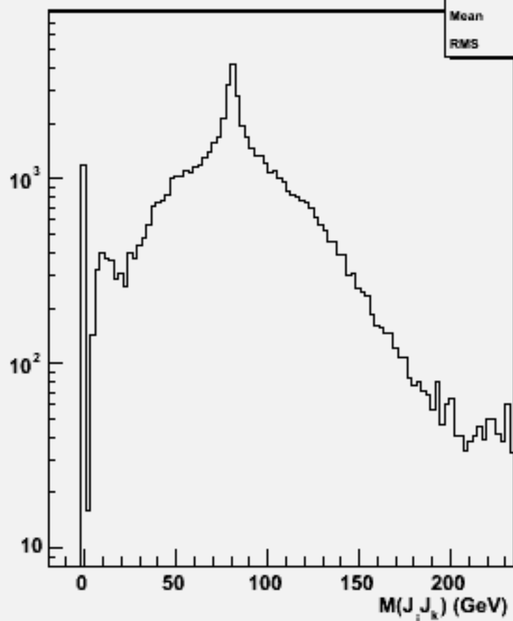
2jets mass(All comb)w101589 n3n3csdu_o
