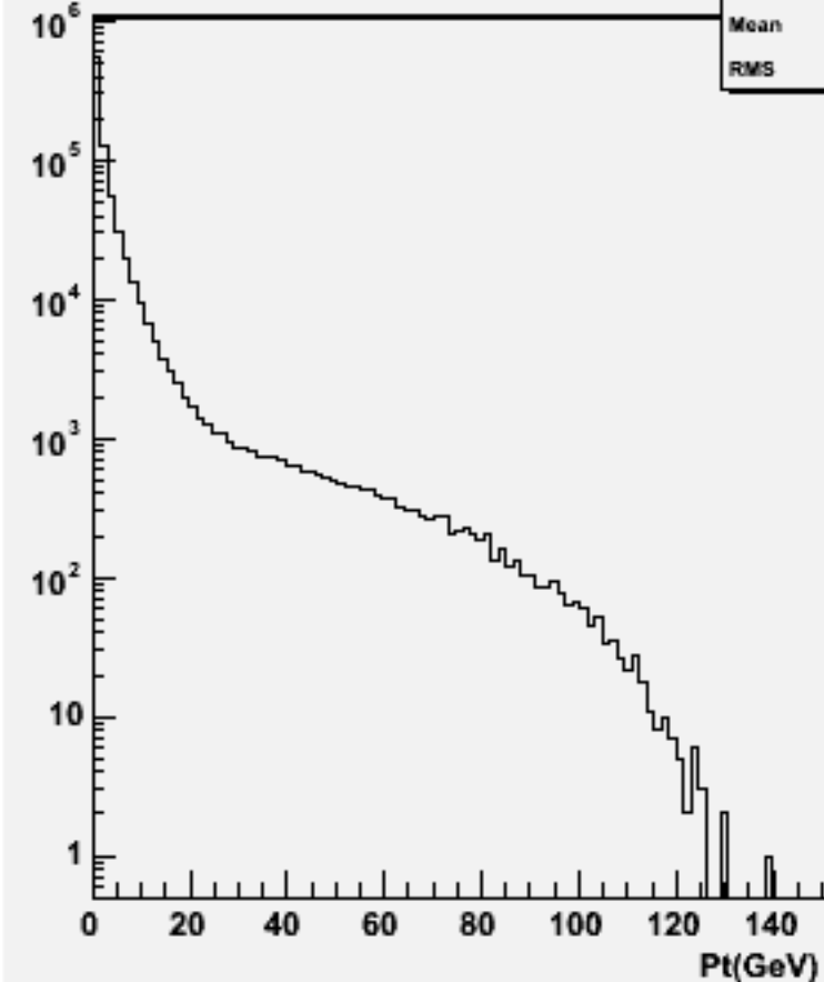
Particle Pt : w101589 n3n3csdu_o
