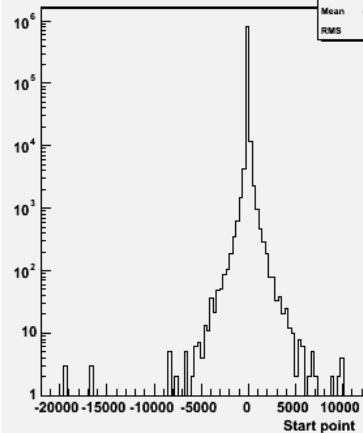
Start point Z : w101589 n3n3csdu_o
