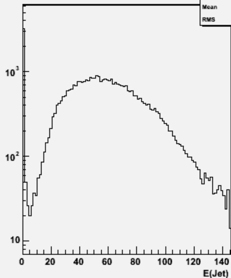
Jet energies(All jets)w101589 n3n3csdu_o
