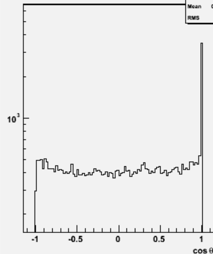
Jet cos \theta (All jets)w101589 n3n3csdu_o
