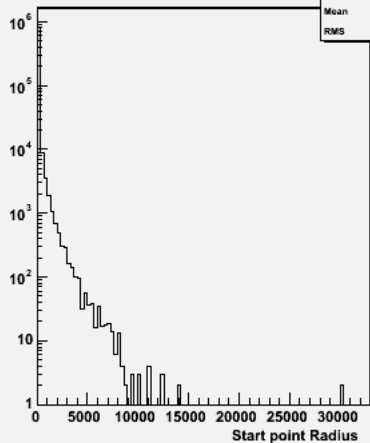
Start point R : w101589 n3n3csdu_o
