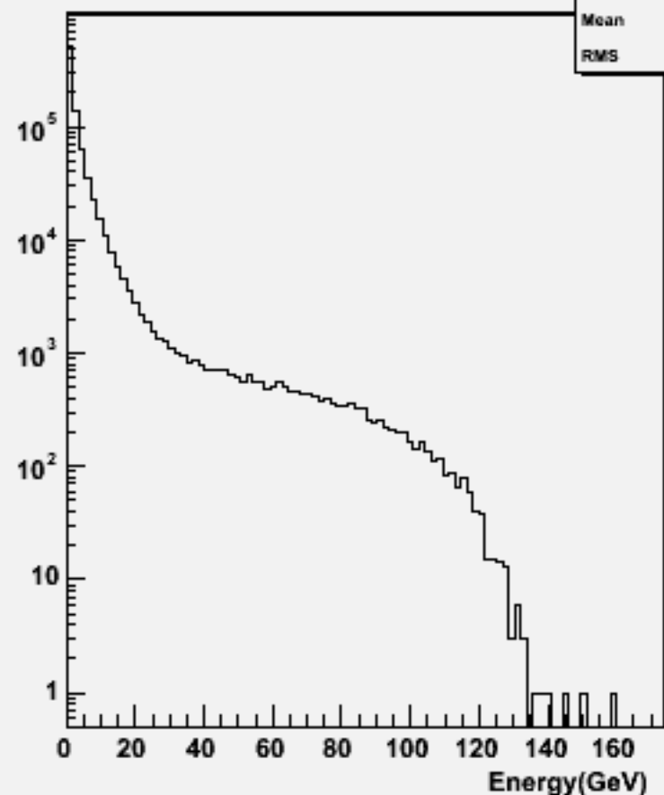
Particle Energy : w101589 n3n3csdu_o
