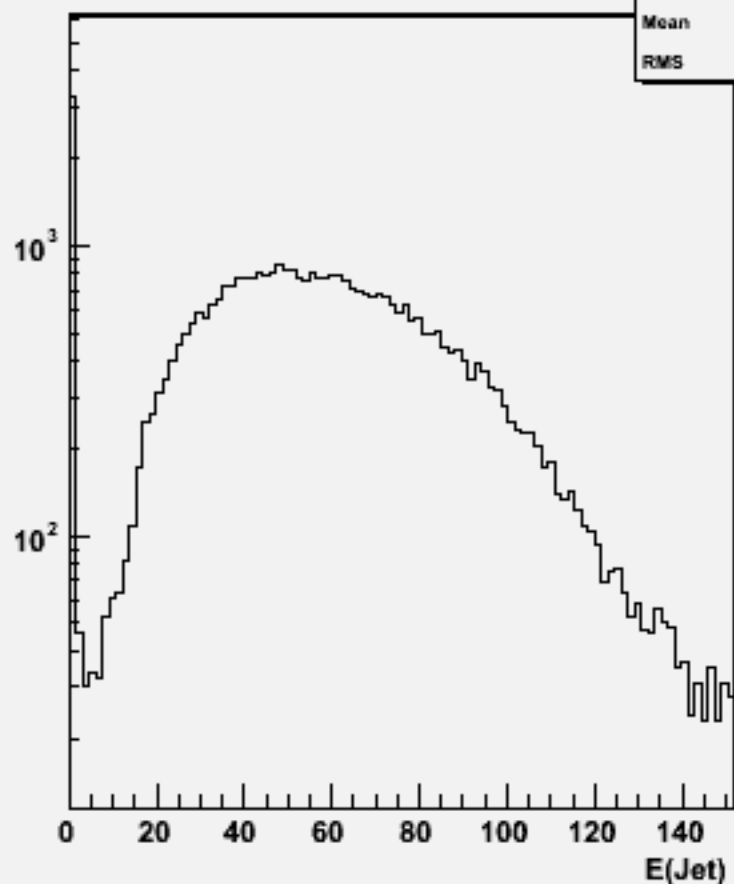
Jet energies(All jets)w101588 n3n3csdu_o
