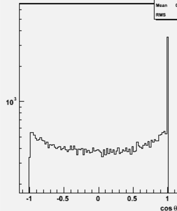
Jet cos \theta (All jets)w101588 n3n3csdu_o
