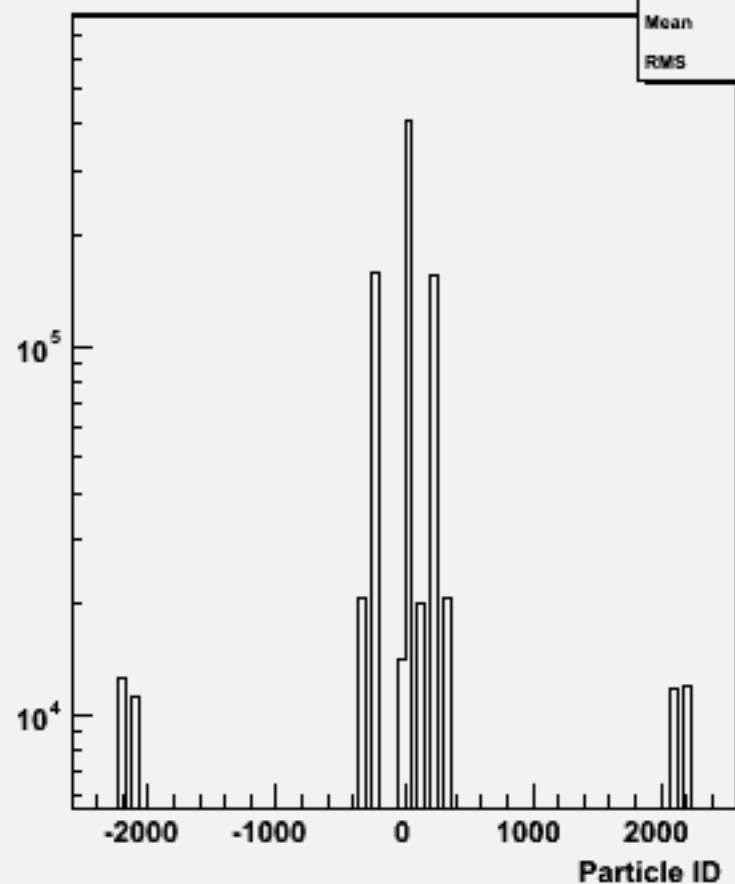
Particle ID : w101588 n3n3csdu_o
