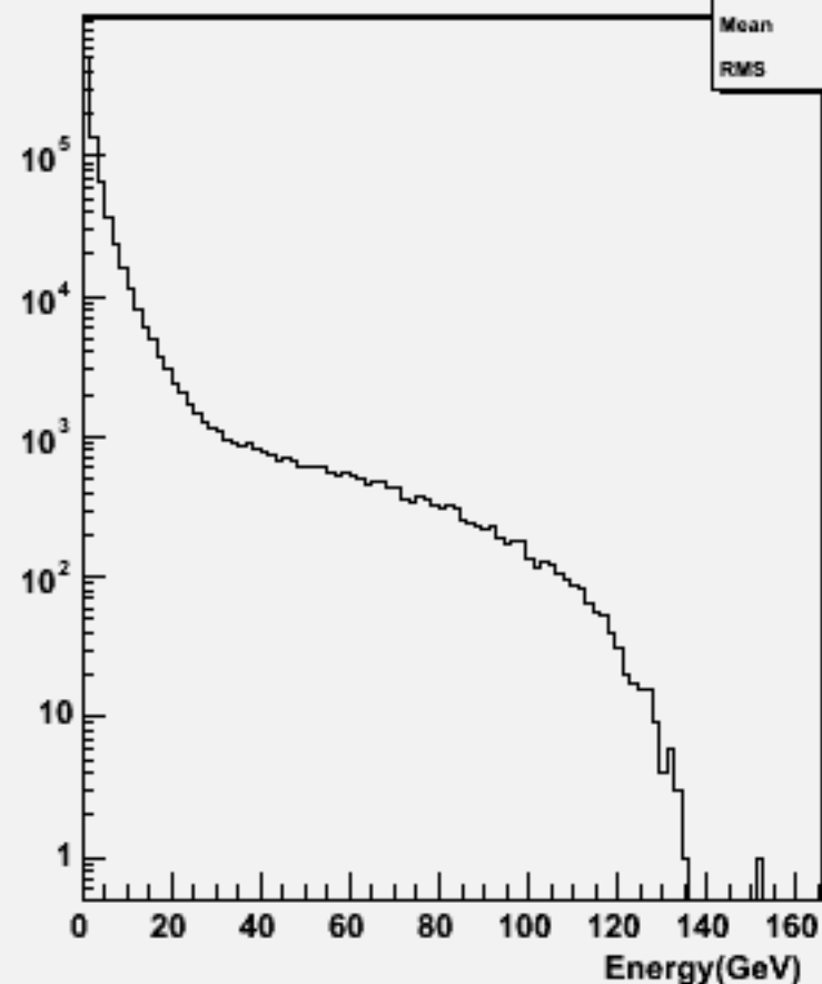
Particle Energy : w101588 n3n3csdu_o
