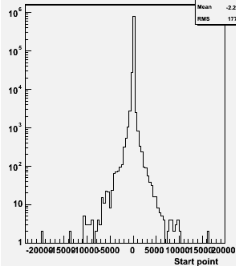
Start point Z : w101588 n3n3csdu_o
