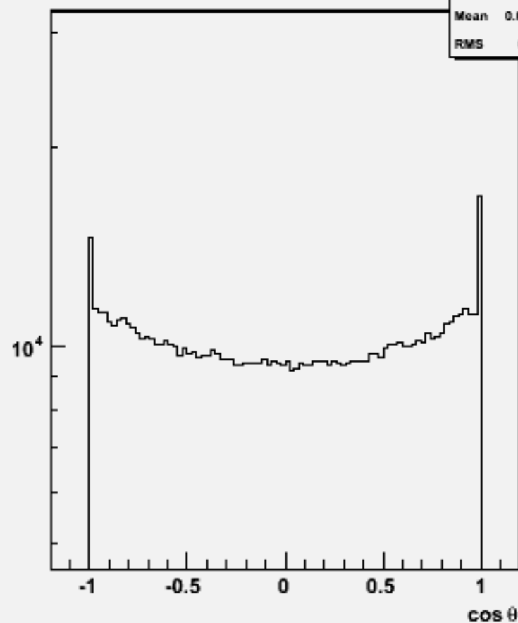
Particle cos \theta : w101588 n3n3csdu_o
