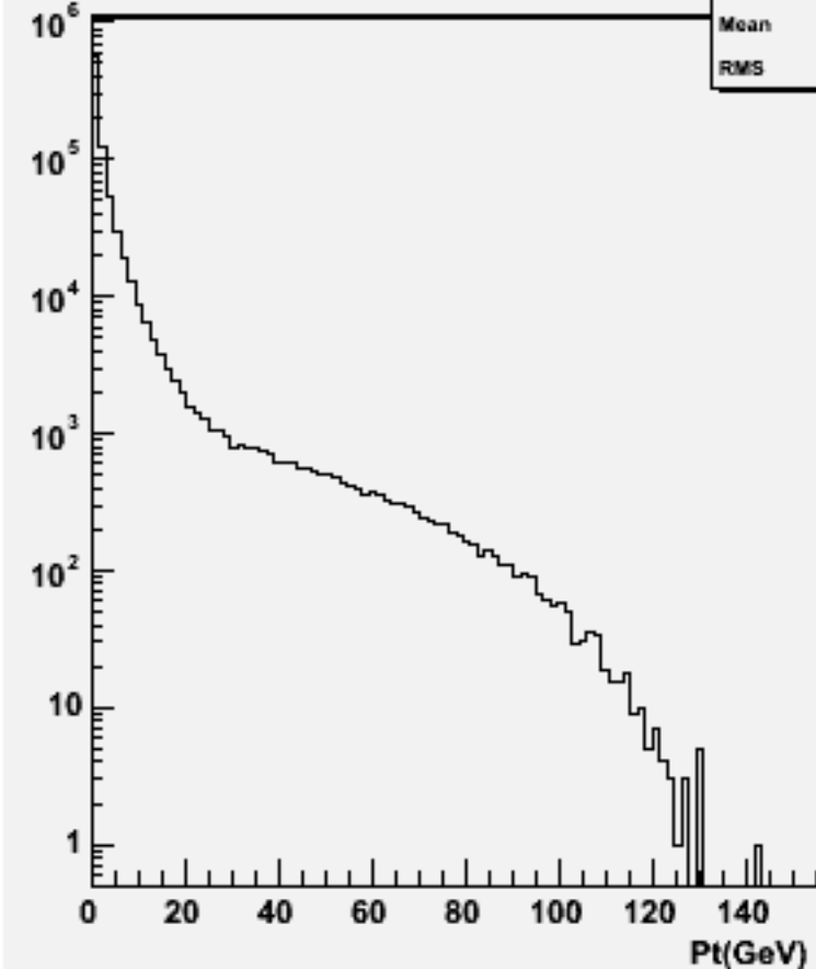
Particle Pt : w101588 n3n3csdu_o
