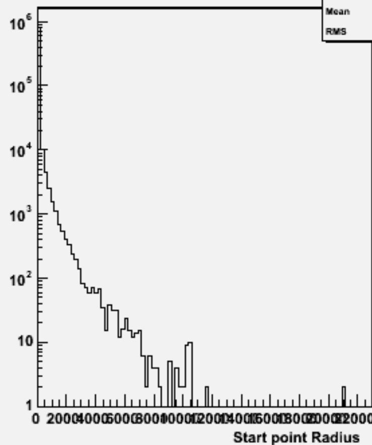
Start point R : w101588 n3n3csdu_o
