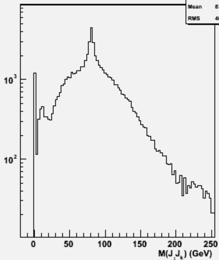
2jets mass(All comb)w101588 n3n3csdu_o
