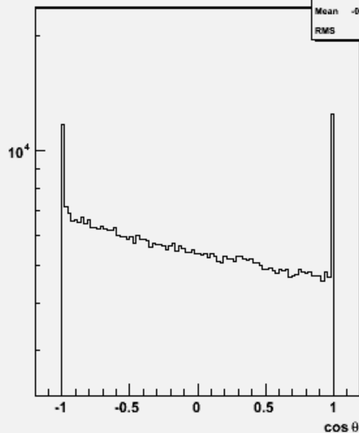
Particle cos \theta : w101581 n3n3cse2n2_o
