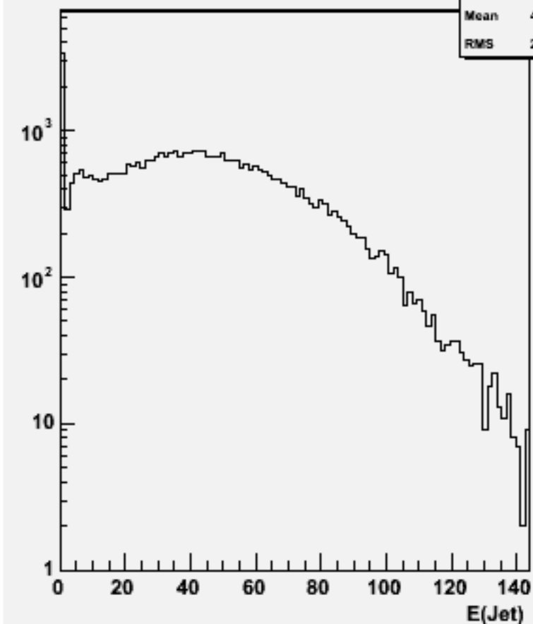
Jet energies(All jets)w101581 n3n3cse2n2_o
