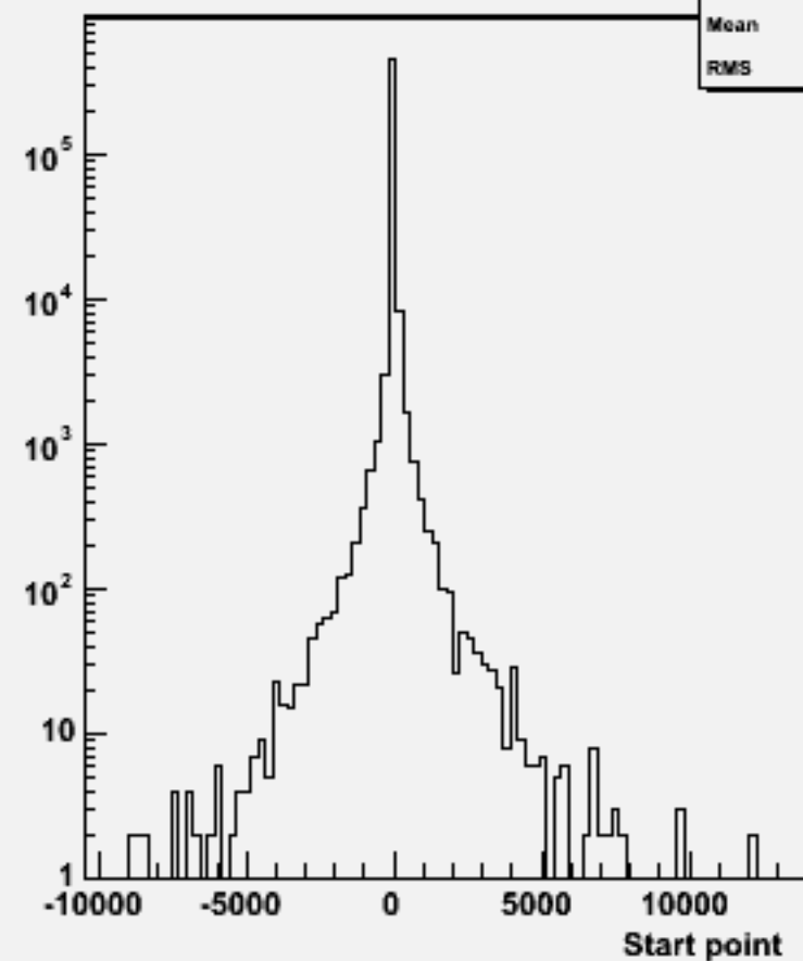
Start point Z : w101581 n3n3cse2n2_o
