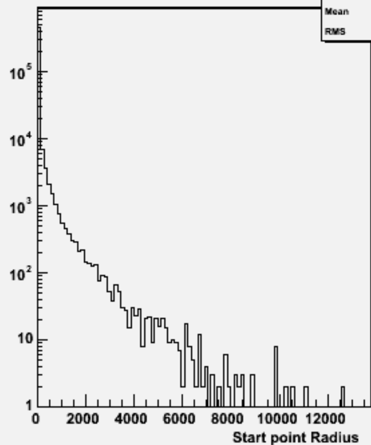
Start point R : w101581 n3n3cse2n2_o
