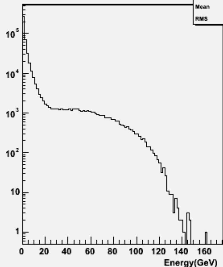
Start point R : w101581 n3n3cse2n2_o
