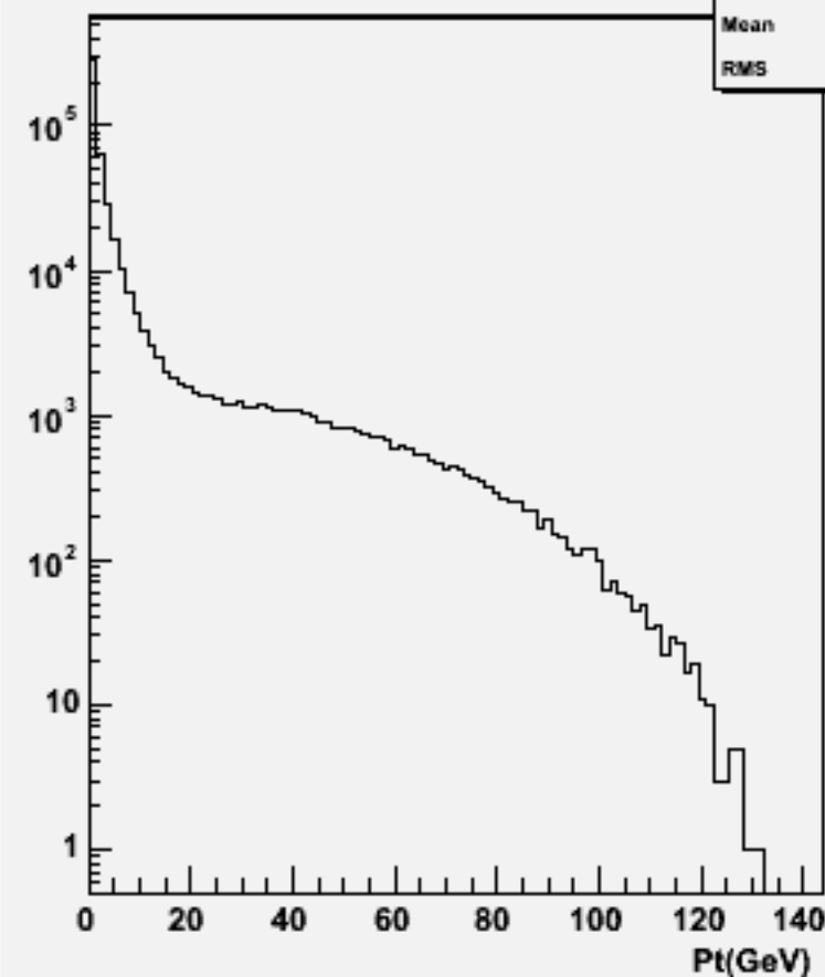
Start point Z : w101580 n3n3cse2n2_o
