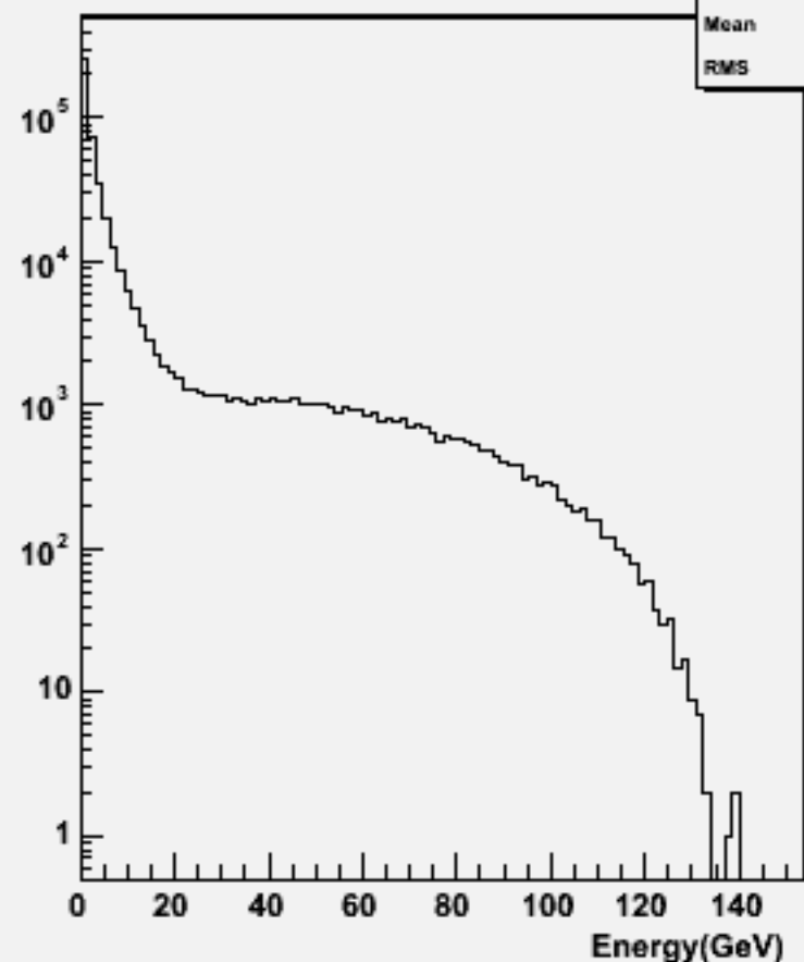
Start point R : w101580 n3n3cse2n2_o
