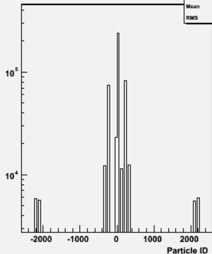
Particle cos \theta : w101580 n3n3cse2n2_o
