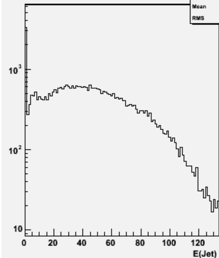
Jet energies(All jets)w101580 n3n3cse2n2_o
