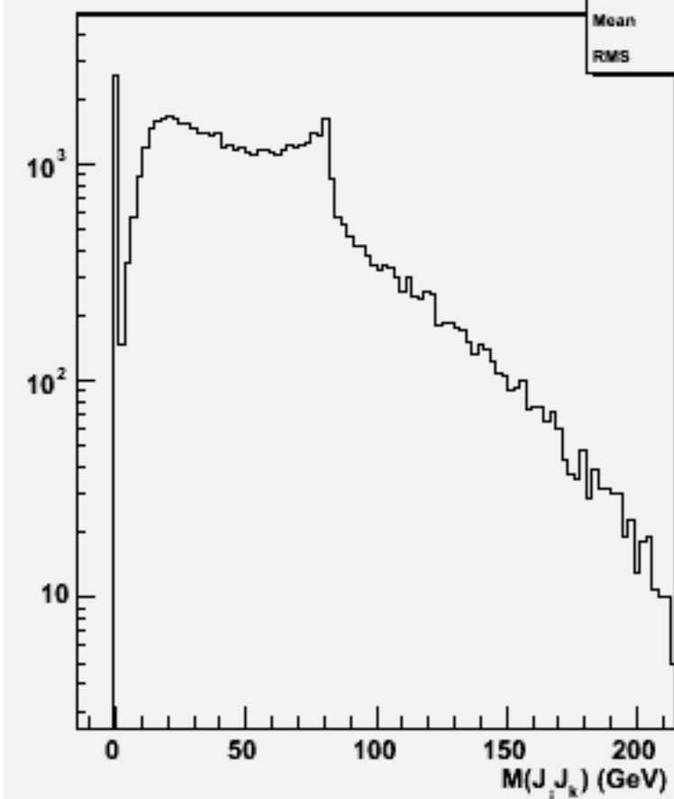
2jets mass(All comb)w101580 n3n3cse2n2_o
