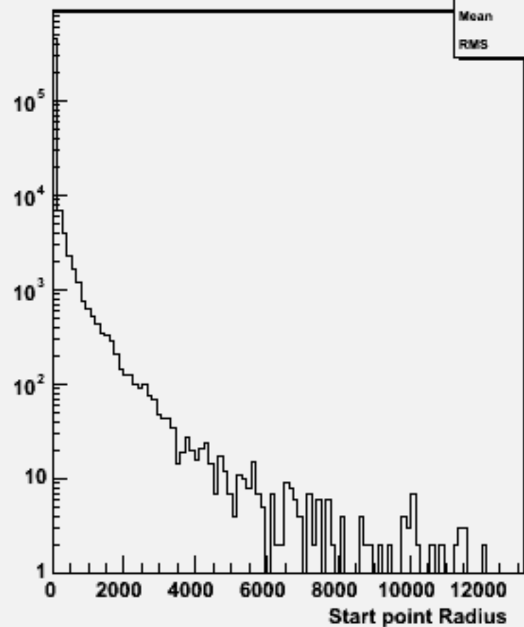
Start point R : w101580 n3n3cse2n2_o
