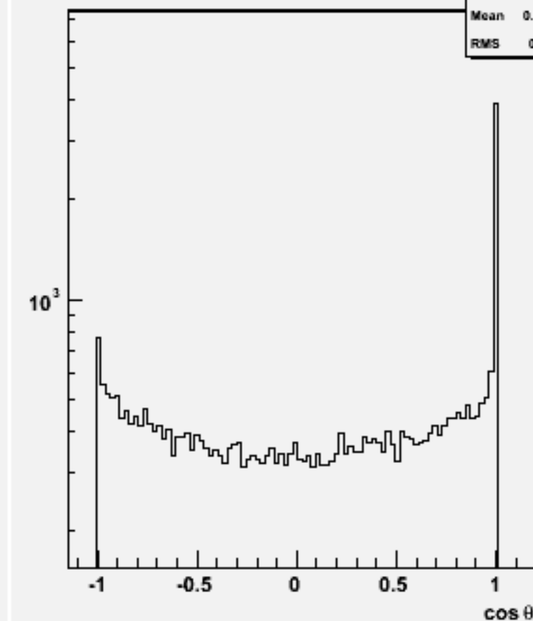
Jet cos \theta (All jets)w101580 n3n3cse2n2_o
